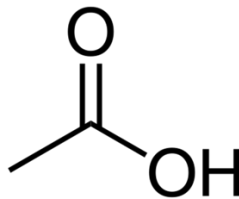
Figure 11 : Représentation schématique de l'acide acétique
