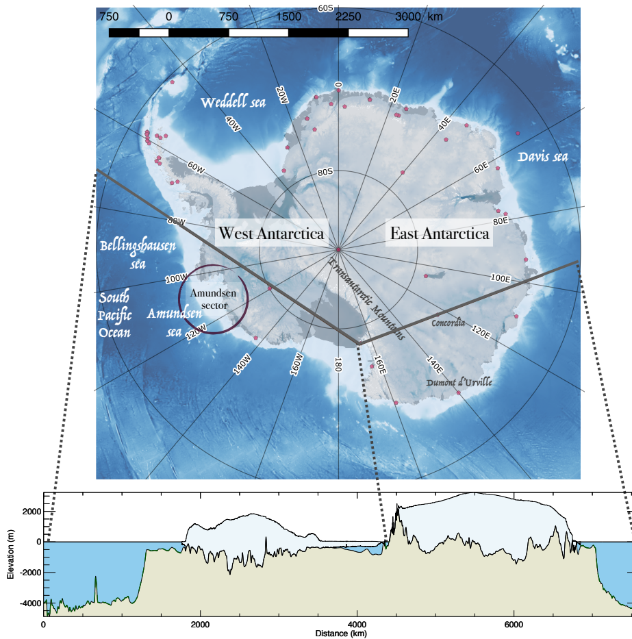
Figure 1 : Carte du continent Antarctique montrant la partie Ouest et Est du continent et le socle rocheux. Le socle rocheux est majoritairement rétrograde sous la partie Ouest. Les bases sont représentées avec des points rouge, Concordia et Dumont d'Urville étant les bases françaises. Les données du socle rocheux sont extraites de Morlighem et al (in prep).
