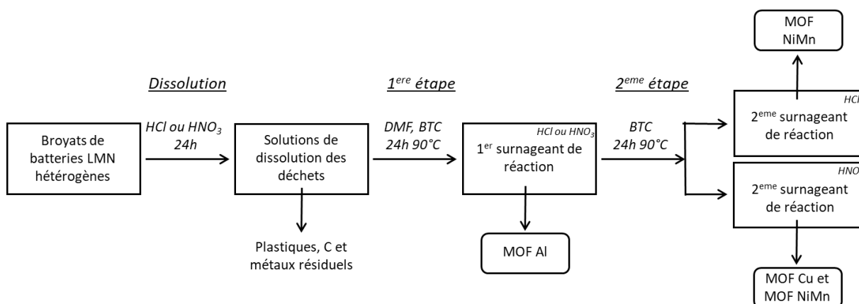
Figure 3-20 : Schéma de la méthode de recyclage par précipitations successives de MOFs
