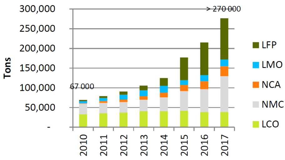
Figure 1-10 : Demande en tonnes au cours du temps des différents types de cathode (Source données : AVICENNE Energy 2018, réf 18)
