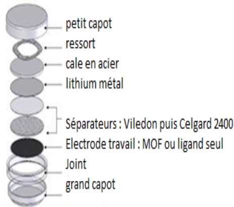
Figure 2-11 : Schéma d'une pile bouton
