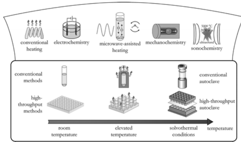
Figure 1-23 : Schéma représentant les différentes méthodes pour synthétiser des MOFs (@2012, American Chemical Society, réf 51)
