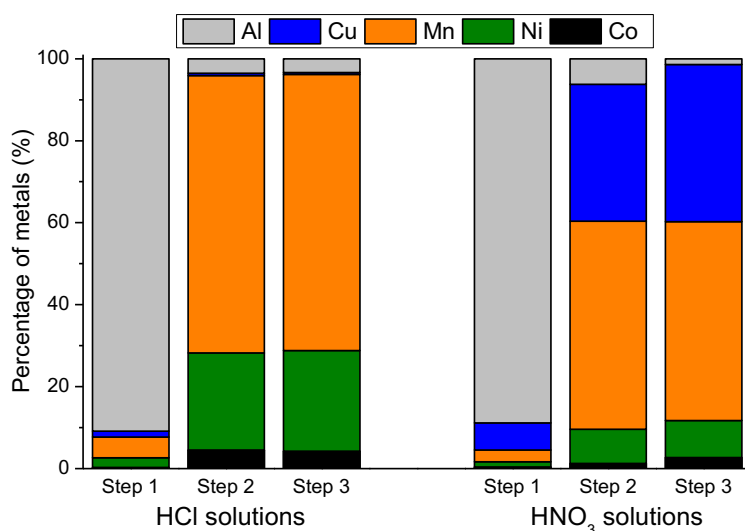
Figure 3-16 : Métaux présents dans les matériaux formés durant les différentes étapes
