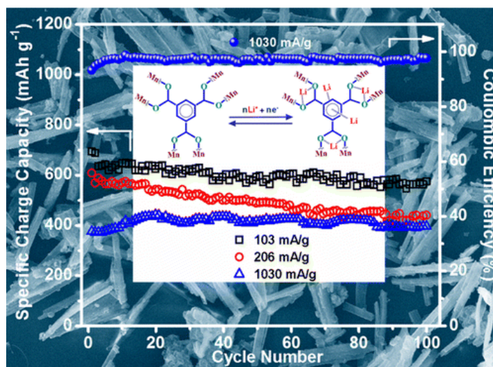
Figure 2-2 : Capacité spécifique du MOF à différentes densité de courant en fonction du nombre de cycle, efficacité coulombienne et schéma de l'insertion du lithium dans le MOF Mn-BTC (©2015, American Chemical Society, réf 11)
