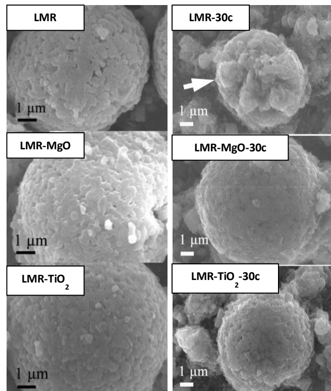
Figure 1-13 : Images MEB des particules LMR, LMR avec un traitement de surface MgO, LMR avec un traitement de surface TiO 2 avant et après 30 cycles de charge/décharge (@2019, Wiley, réf 35)
