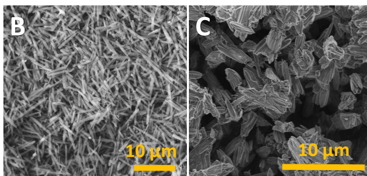
Figure 3-29 : ATG (A) et cliché MEB des MOFs synthétisé avec le BDC dans HCl (B) et dans HNO 3 (C)
