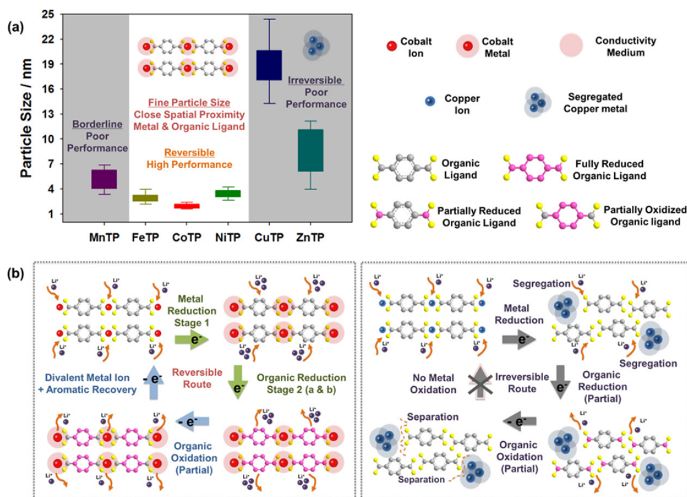
Figure 2-3 : (a) Taille des particules des différents matériaux (b) Schémas des mécanismes électrochimiques pour le MOF Co en comparaison du MOF Cu (@2018, American Chemical Society, réf 12)
