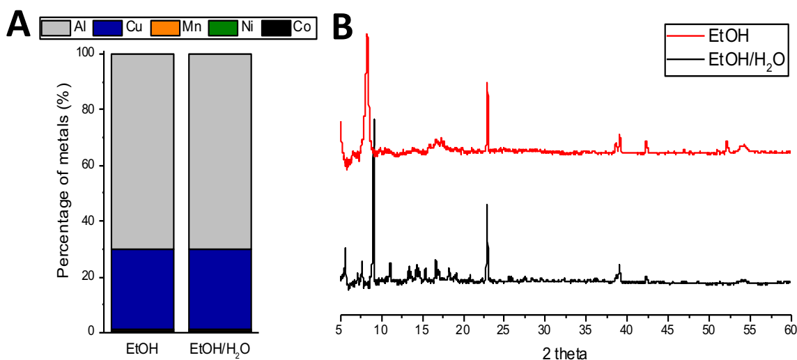
Figure 3-27 : Métaux présents (A) et DRX sur poudre (B) des matériaux formés avec d'autres solvants dans HNO 3
