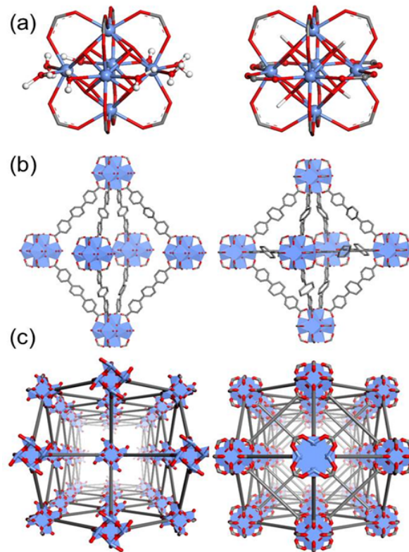
Figure 1-21 : Structures des MOFs de type UiO-68 dont les clusters sont reliés par 8 ligands (gauche) et 12 ligands (droite) (@2014, Wiley, réf 70)
