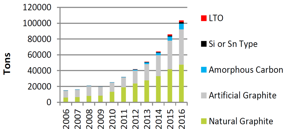
Figure 1-14 : Demande en tonnes au cours du temps des différents types d'anodes (Source données : AVICENNE Energy 2016, réf 19)
