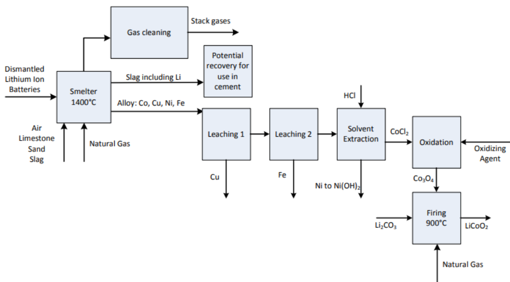
Figure 3-2 : Procédé de recyclage par pyroméallurgie (Source : Tytgat 2011, Umicore 2013)
