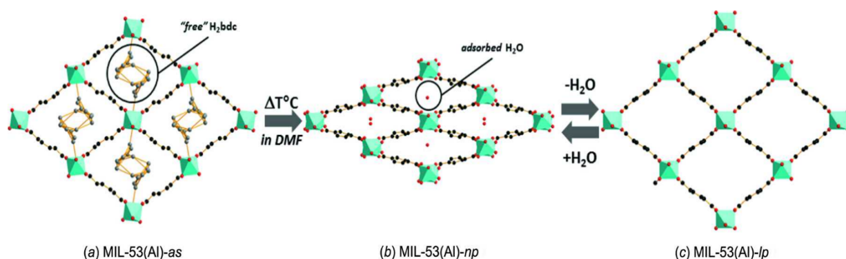
Figure 1-22 : Structure du MOF MIL-53(Al) (a) en fin de synthèse avec la présence de BDC libre dans les pores, (b) avec la présence de molécule d'eau dans les pores donnant lieu à une contraction du réseau et (c) avec les pores ouverts et vides (@2017, Wiley, réf 73)
