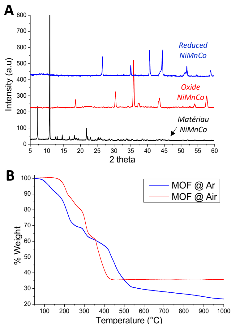
Figure 2-20 : Diffractogrammes des matériaux (A) et analyses thermogravimétriques (B)
