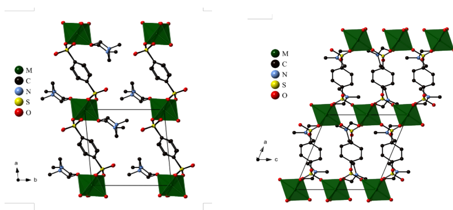
Figure 2-15 : Vues de la structure cristallographique du MOF Mn(BDS)(DMF) 2
