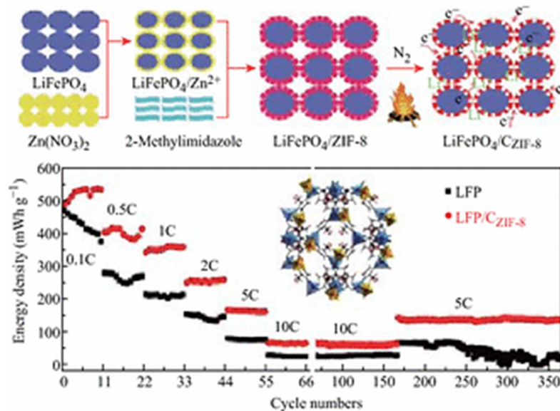
Figure 2-7 : Stratégie de synthèse de LFP/CZIF-8 et performances électrochimique du matériau comparé au LFP simple (@2018, Springer Berlin Heidelberg, réf 20)
