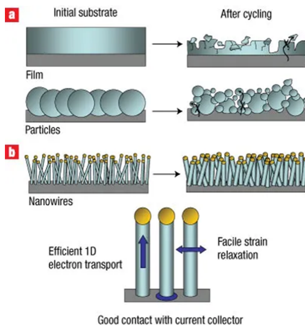
Figure 1-15 : Schéma des changements morphologiques durant le cyclage dans le silicium (a) mis en forme de film ou de particules (b) sous forme de nanofils (@2008, Nature, ref 38)
