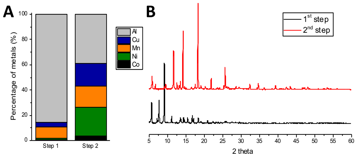
Figure 3-23 : Proportions des métaux présents dans les matériaux formés dans H_2SO_4:H_2O_2 (A) et leur DRX sur poudre (B)
