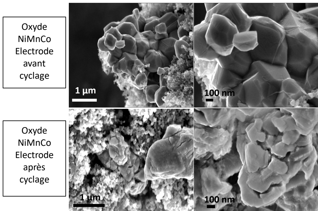
Figure 2-25 : Images MEB de l'électrode avec l'oxyde avant cyclage (haut) et après cyclage (bas)
