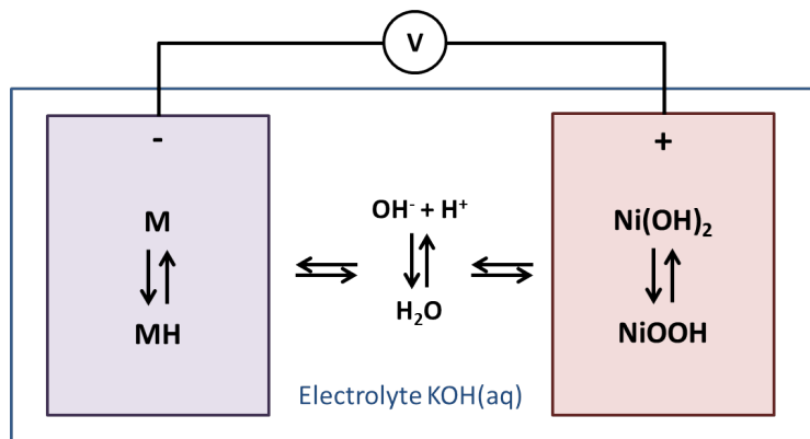
Figure 1-3 : Schéma de fonctionnement d'une batterie Ni-MH
