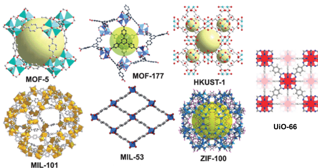
Figure 1-16 : Structures de quelques MOFs connus (Adapté de ©2010, Royal Society of Chemistry)
