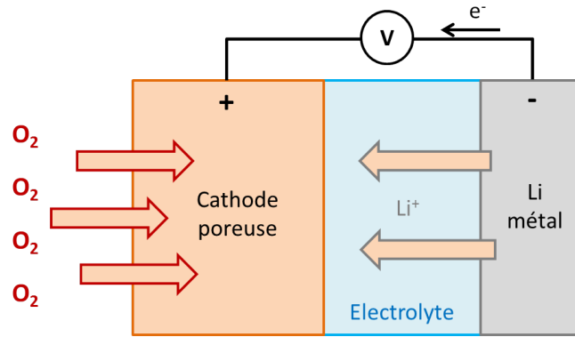
Figure 1-5 : Schéma de fonctionnement d'une batterie Li/air
