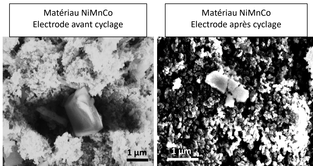
Figure 2-26 : Images MEB de l'électrode avec le matériau hybride avant et après cyclage
