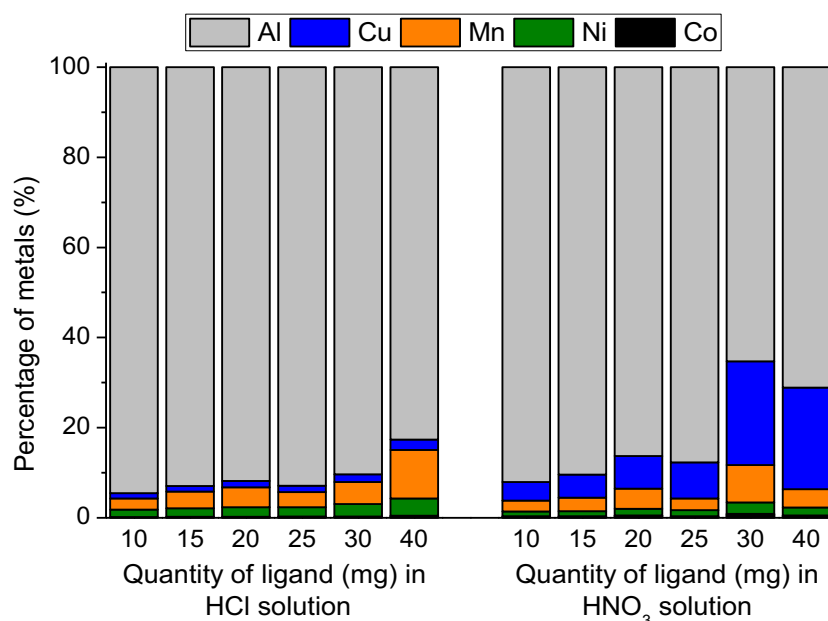
Figure 3-14 : Métaux présents dans les matériaux formés avec différentes quantités de ligand
