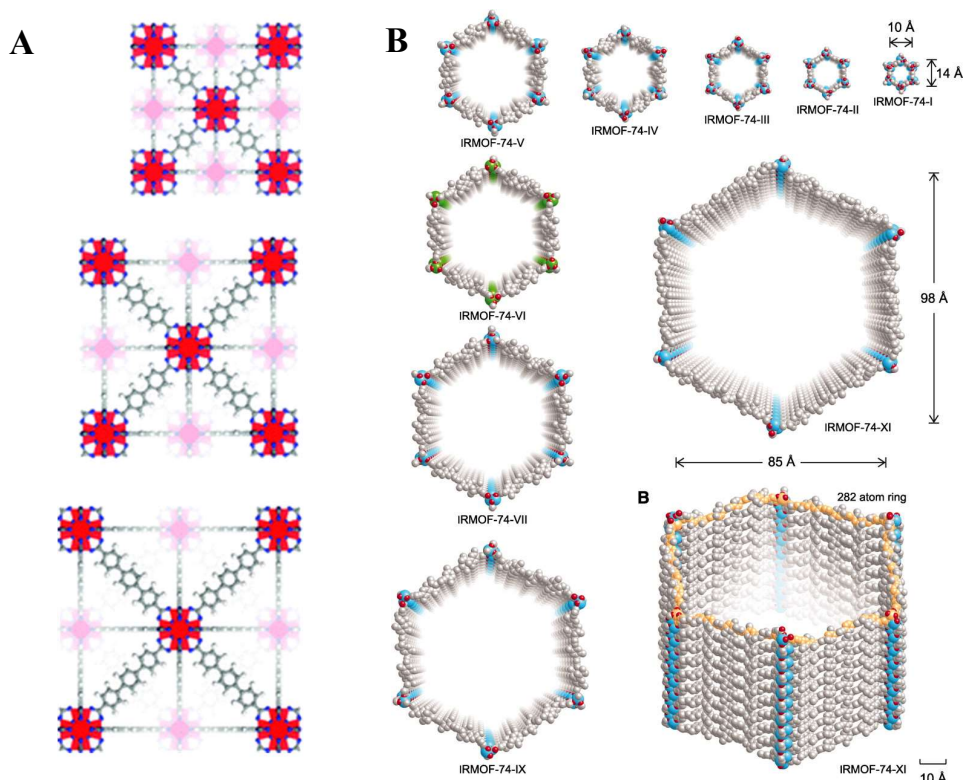
Figure 1-18 : (A) Série isostructurale des MOFs UiO-66, UiO-67 et UiO-68 (@2008, American Society of Chemistry, réf 47 ), (B) Représentation des MOFs de I à XI de la série IRMOF-74 (@2012, Science, réf 61)
