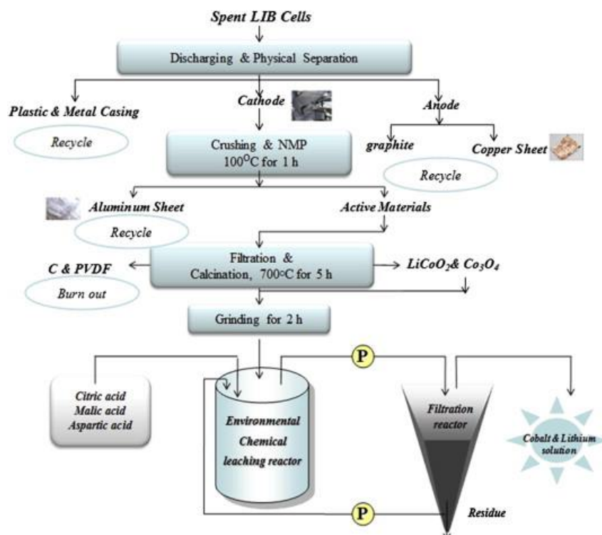
Figure 3-3 : Exemple de procédé par hydrométallurgie (©2013, Elsevier)
