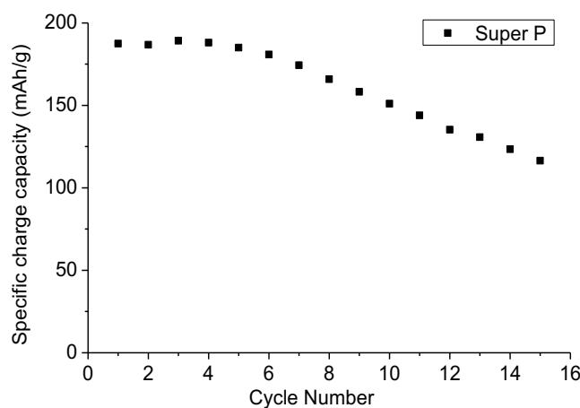
Figure 2-14 : Capacité spécifique du carbone Super P seul en fonction du nombre de cycles
