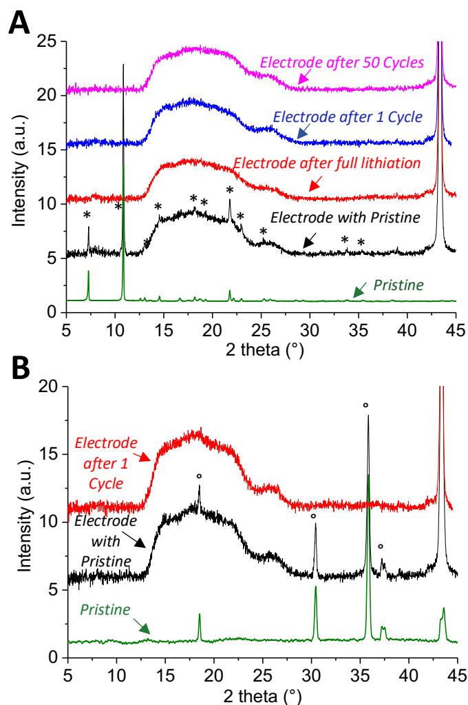
Figure 2-24 : Analyses DRX ex situ des piles du MOF NiMnCo (A) et de l'oxyde (B)
