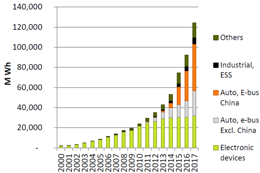
Figure 1-8 : Ventes de batteries Li-ion en MWh dans le monde entre 2000 et 2017 (Source données : AVICENNE Energy 2018, réf 18)
