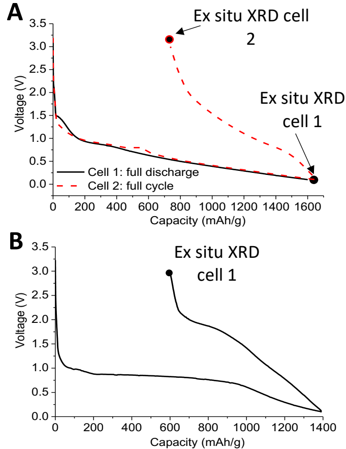
Figure 2-23 : Courbes galvanostatiques des piles utilisées pour les analyses ex situ du matériau NiMnCo (A) et de l'oxyde (B)
