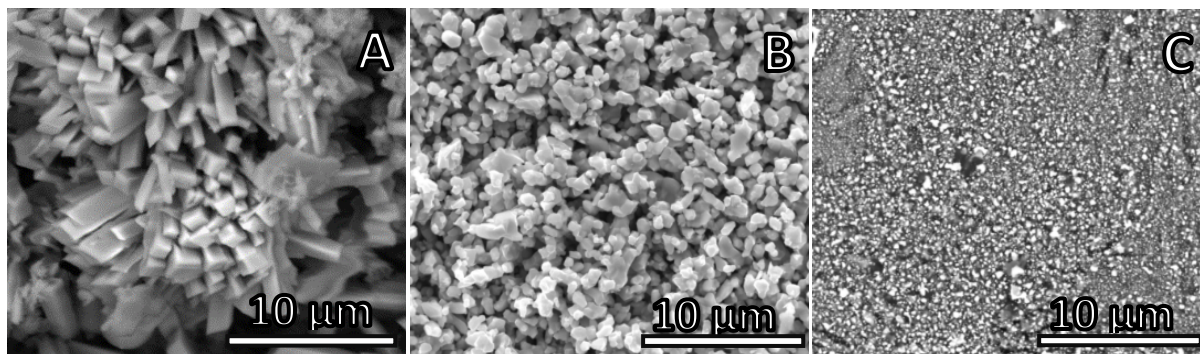
Figure 2-19 : Images MEB du composé NiMnCo (A), de l'oxyde NiMnCo (B) et du matériau réduit NiMnCo (C)
