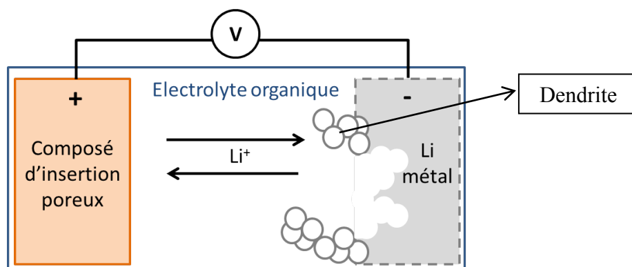
Figure 1-4 : Schéma de fonctionnement d'une batterie Li métal avec le risque de formation de dendrites
