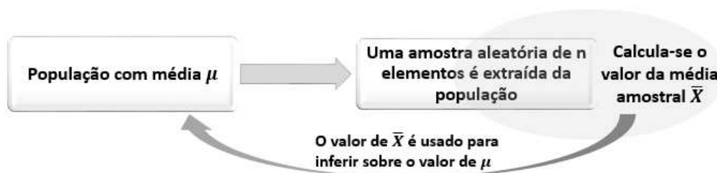
Figura 35 - Distribuição amostral da média: com e sem reposição
