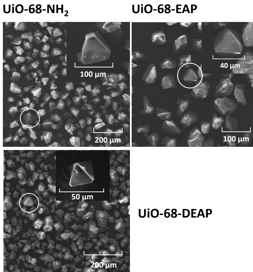
Figure 89 : Clichés MEB des matériaux UiO-68-NH 2 , UiO-68-DEAP et UiO-68-EAP
