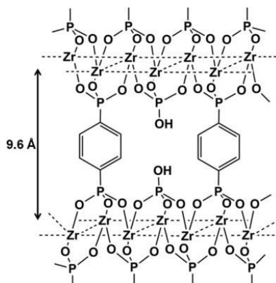
Figure 38 : Structure d'un matériau type zirconium phosphonate-phosphate d'après Silbernel et al. 151
