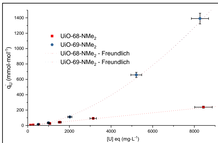
Figure 96 : Isothermes d'adsorption corrélées avec le modèle de Freundlich pour les MOFs UiO-68-NMe 2 et UiO-69-NMe 2
