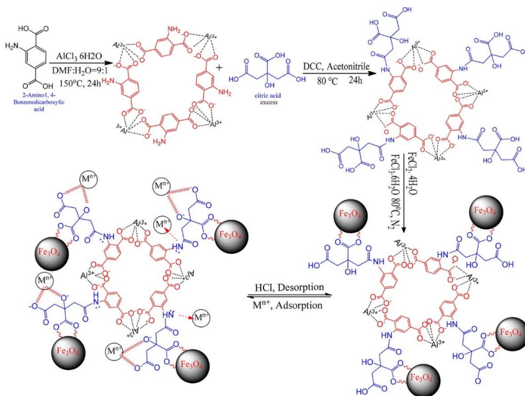
Figure 23 : Schéma de synthèse du MOF Fe 3 O 4 @AMCA-MIL-53(Al)
