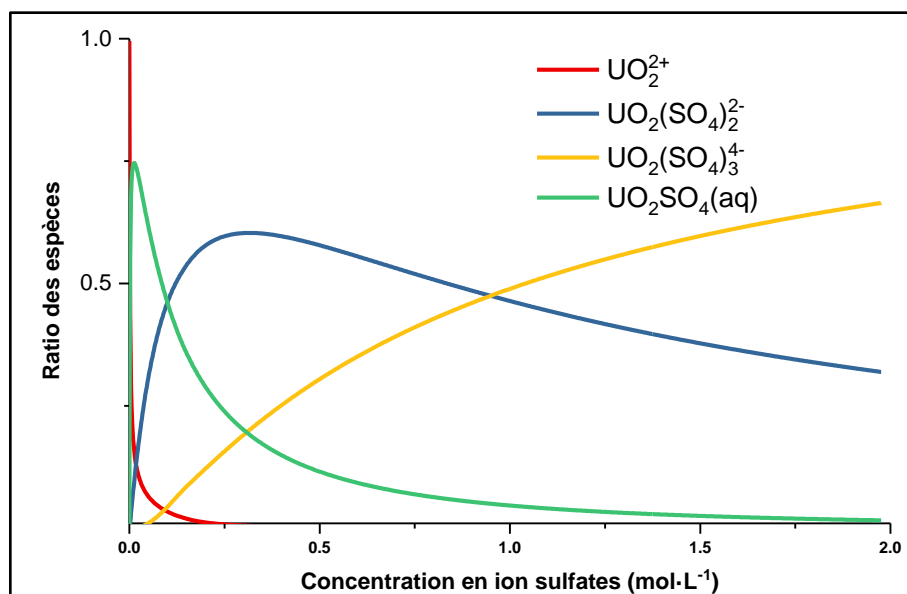
Figure 99 : Diagramme de spéciation de l'uranium(VI) en fonction de la concentration en sulfates (pH = 2, C_{U\text{ initial}} = 1000\text{ mg}\cdot\text{L}^{-1} ) modélisé à partir des données de la base NEA
