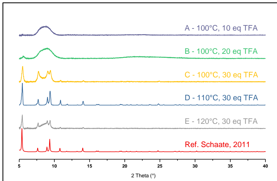
Figure 72 : Comparaison des diffractogrammes poudres obtenus à partir du criblage pour la synthèse de l'UiO-68-NH 2
