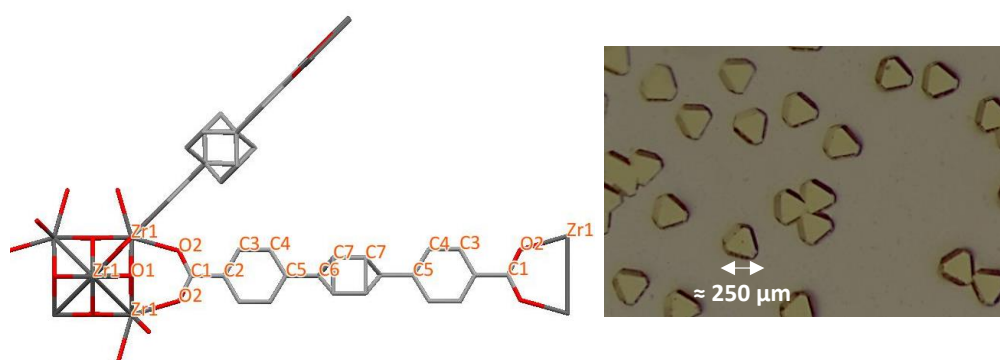
Figure 73 : Gauche, schéma d'un cluster de zirconium et du ligand TPDC coordonné. Droite, cliché pris au microscope optique des cristaux UiO-68-NMe 2 avec un zoom x40
