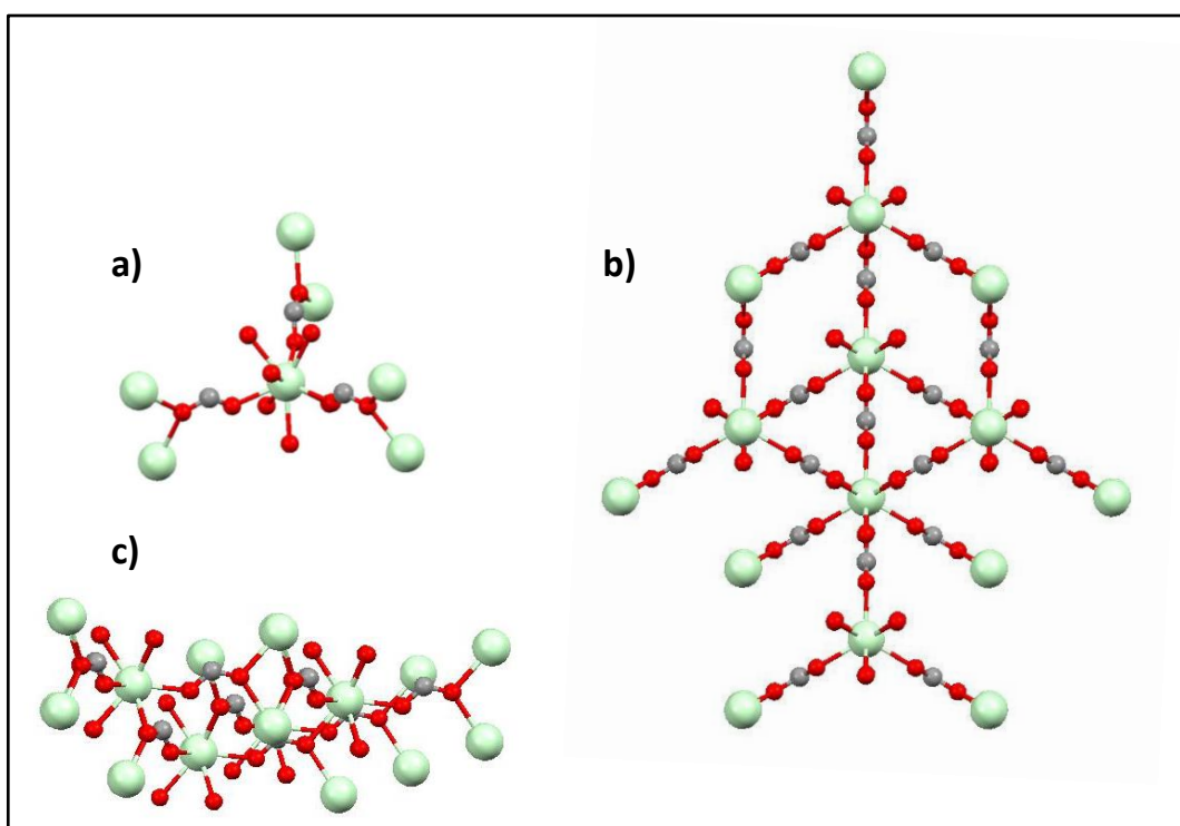
Figure 47 : Structure en 3D du matériau C_3H_3Nd_1O_6 . a), Motif de base, b) Projection celons l'axe Z, c) Projection celons l'axe Y
