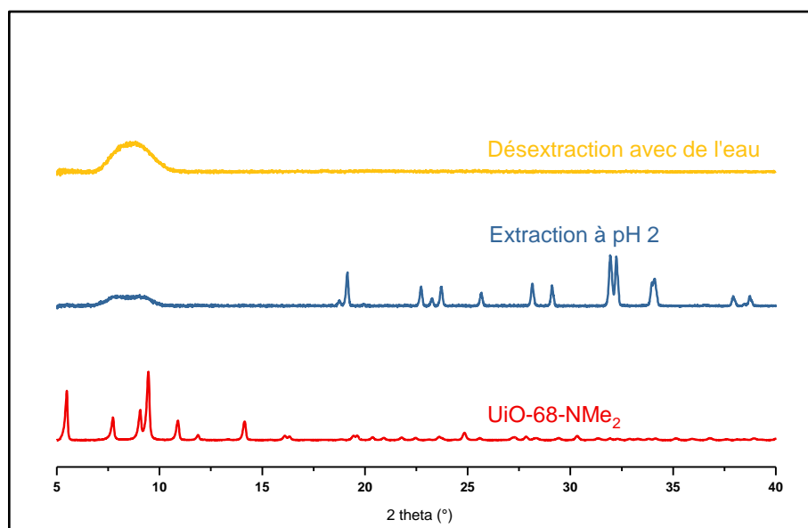
Figure 110 : Suivi de la cristallinité par DRX après extraction à pH 2 et dés extraction avec de l'eau pour l'UiO-68-NMe 2
