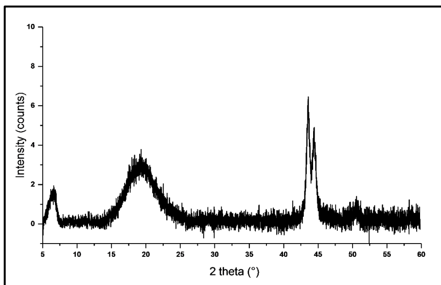
Figure 30 : Diffractogramme DRX poudre d'un matériau Zr-BDS avec ZrCl_4 , DMF, sans modulateur, 120^\circ C
