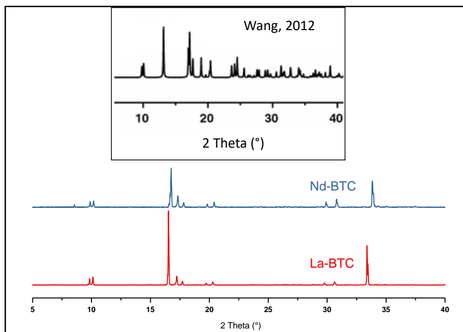
Figure 43 : Comparaison des diffractogrammes expérimentaux des MOFs La-BTC et Nd-BTC avec le diffractogramme théorique du \text{LaBTC}(\text{H}_2\text{O})_6 à partir d'un graphique de Wang (2012)
