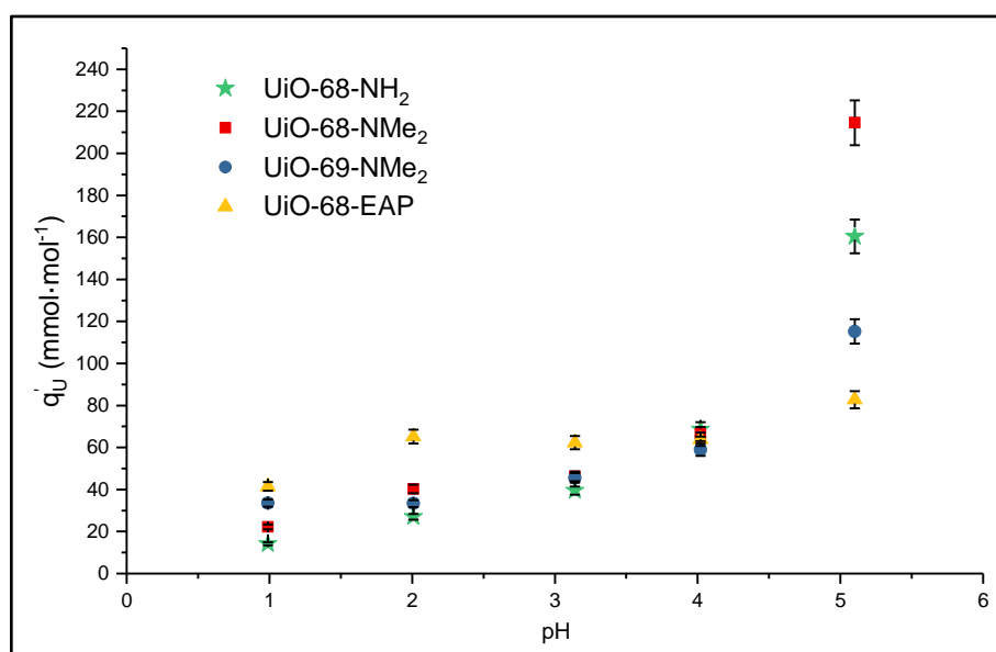
Figure 103 : Capacité d'extraction en fonction du pH en milieu sulfaté pour UiO-68-NH 2 , UiO-68-NMe 2 , UiO-69-NMe 2 et UiO-68-EAP
