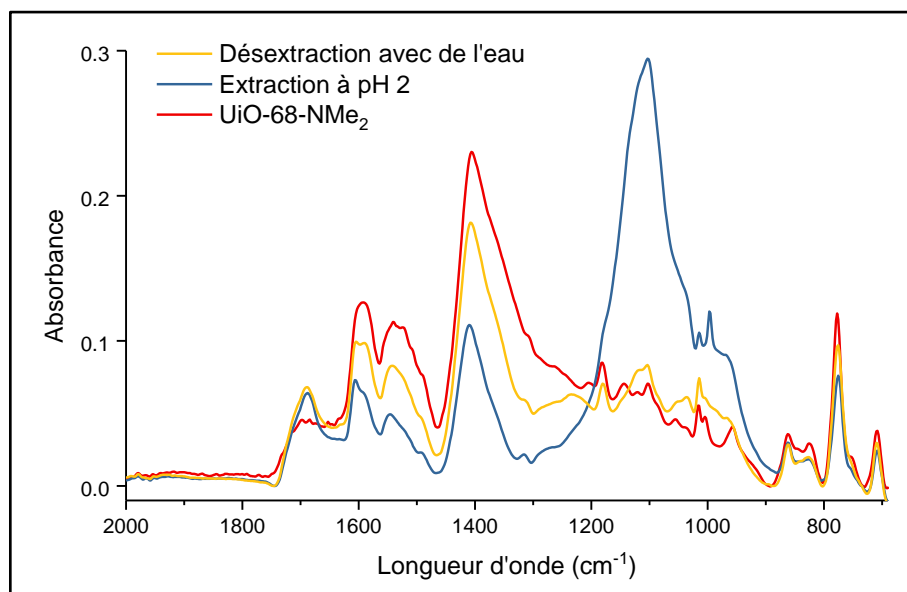
Figure 111 : Analyse FT-IR après extraction à pH 2 et désorption avec de l'eau pour l'UiO-68-NMe 2
