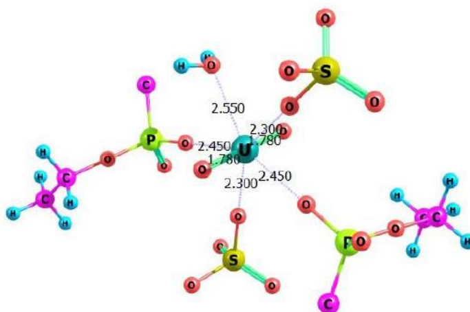
Figure 101 : Complexation du complexe [\text{UO}_2(\text{SO}_4)_2]^{2-} par des silices mésoporeuses fonctionnalisées (Charlot, 2016)
