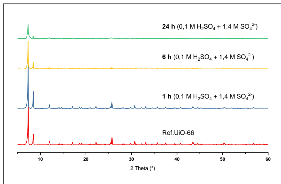
Figure 50 : Stabilité de l'UiO-66 en fonction du temps après contact avec une solution à 0,1 mol·L -1 en acide sulfurique et 1,4 mol·L -1 en sulfates ajoutés
