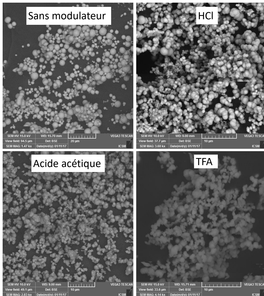
Figure 31 : Clichés MEB du matériau Zr-BDS obtenu à partir du ZrCl_4 dans le DMF sans modulateur, avec l'acide chlorhydrique, l'acide acétique et le TFA. Echelle 20 μm sans modulateur et 10 μm avec modulateur. Sonde BSE 10 ou 15 kV, distance de travail = 9 mm ou 15,7 mm
