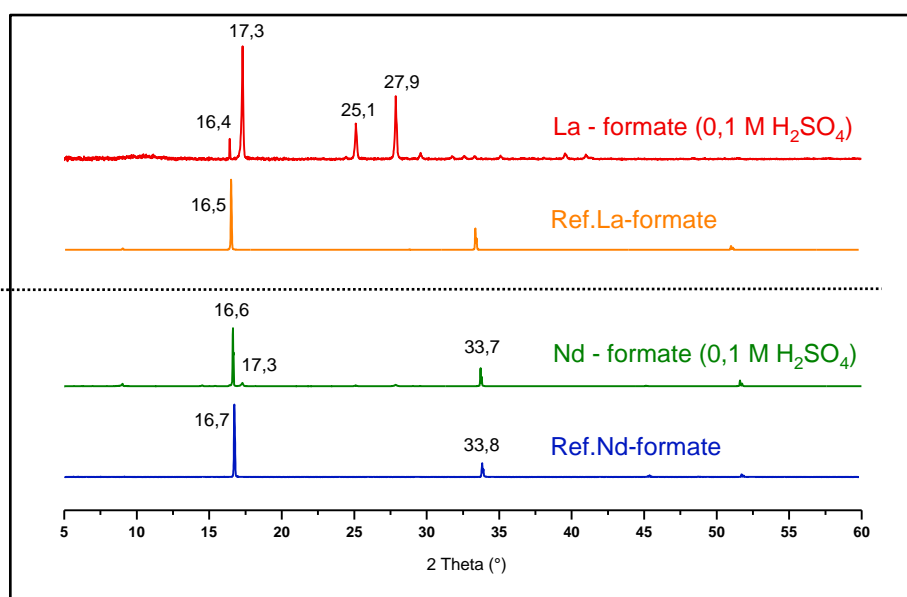
Figure 53 : Stabilité des matériaux La-formate et Nd-formate après une heure de contact avec l'acide sulfurique 0,1 \text{ mol}\cdot\text{L}^{-1}
