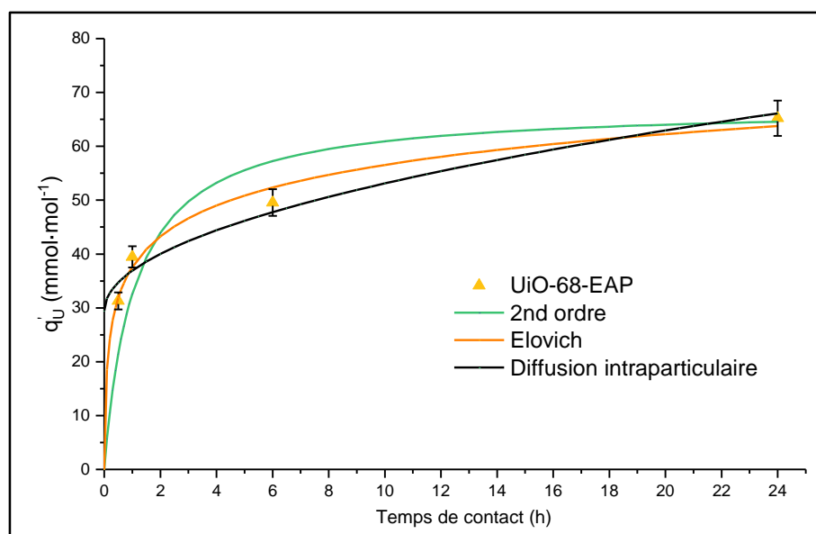
Figure 94 : Profil cinétique du MOF UiO-68-EAP comparé aux profils théoriques obtenus avec le modèle pseudo cinétique de second ordre, d'Elovich et celui de Weber et Morris
