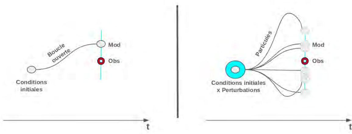
FIGURE 5.3 – Le schéma de gauche représente la modélisation en boucle ouverte, et celui de droite décrit une simulation d'ensemble de particules. Cette dernière consiste à générer des perturbations des conditions initiales afin de réduire les erreurs de modélisation ou de forçages.
