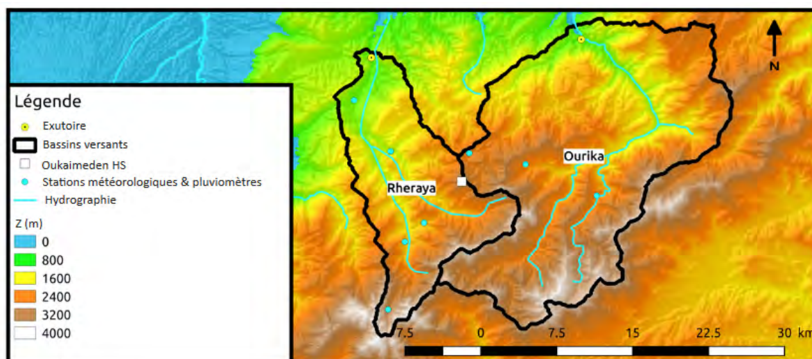
FIGURE 2.6 – Localisation des données hydro-météorologiques utilisées au cours de cette étude. Oukaïmeden HS est la station de mesure de la hauteur de la neige ( snow height ).
