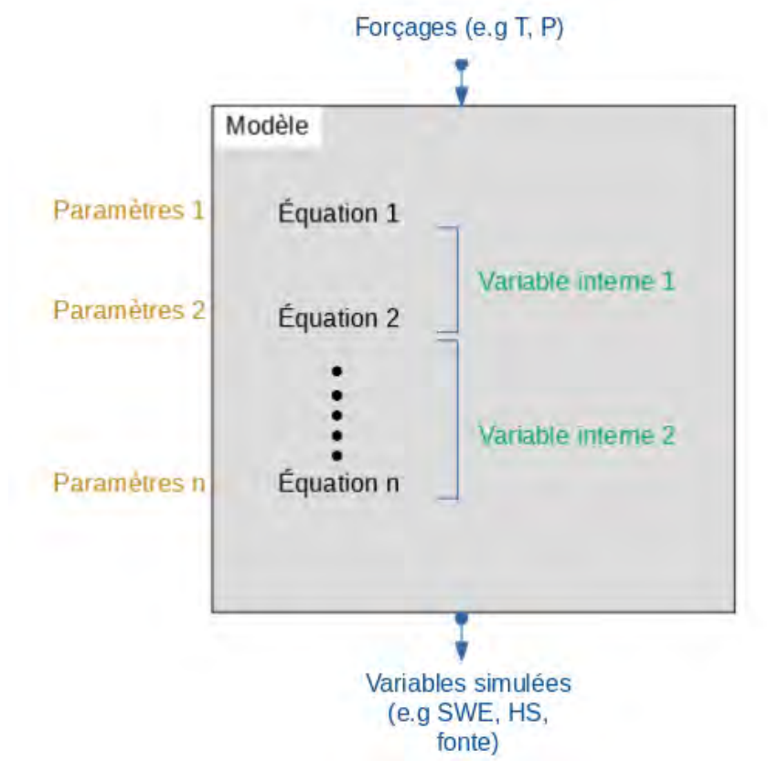
FIGURE 1.7 – Structure d'un modèle de neige
