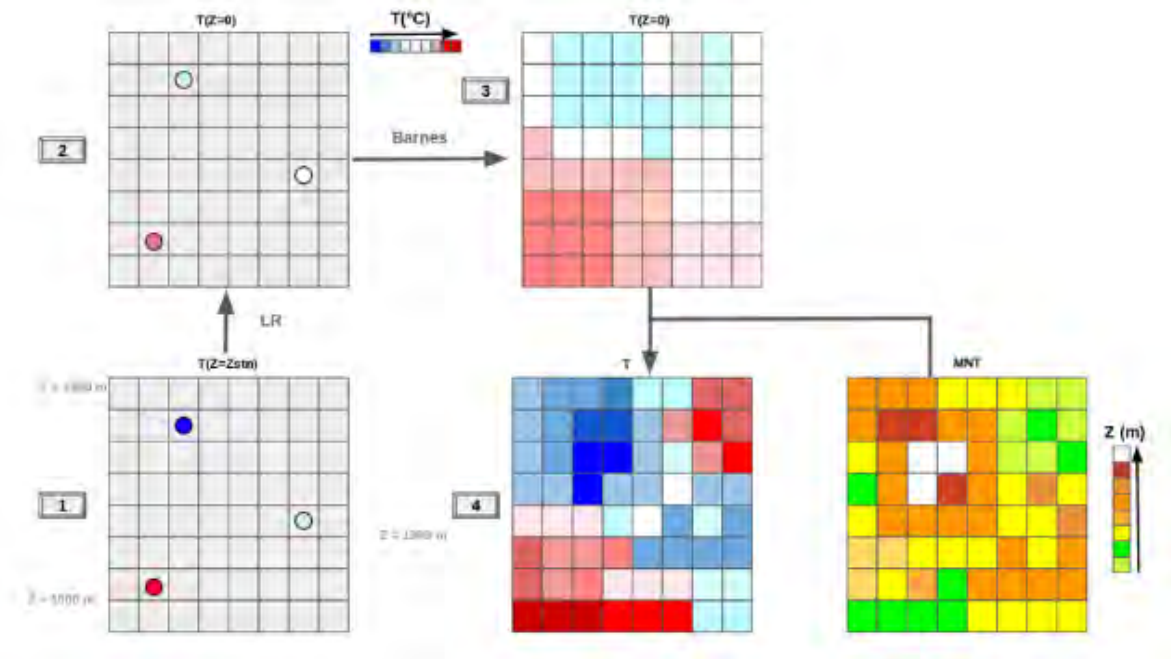
FIGURE 2.8 – Simplification du processus de spatialisation de la température par Micro-Met. De (1) à (2) : Utilisation du facteur de correction de la température ( temperature lapse rate ) pour passer les températures observées des altitudes des stations, aux températures à la surface de référence ( Z = 0 \text{ m} ). De (2) à (3) Spatialisation des températures à la surface de référence à l'aide du schéma de Barnes. De (3) à (4) Deuxième utilisation du facteur de correction de la température ( temperature lapse rate ) (Eq. 2.4)
