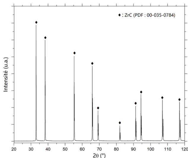
Figure III.1. Diagramme de diffraction des rayons X de l'oxycarbure de zirconium synthétisé
