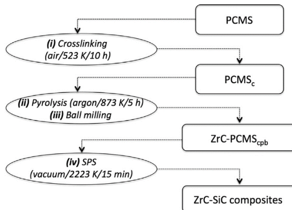
Figure I.29. Processus d'élaboration des composites ZrC/SiC par voir hybride [28]
