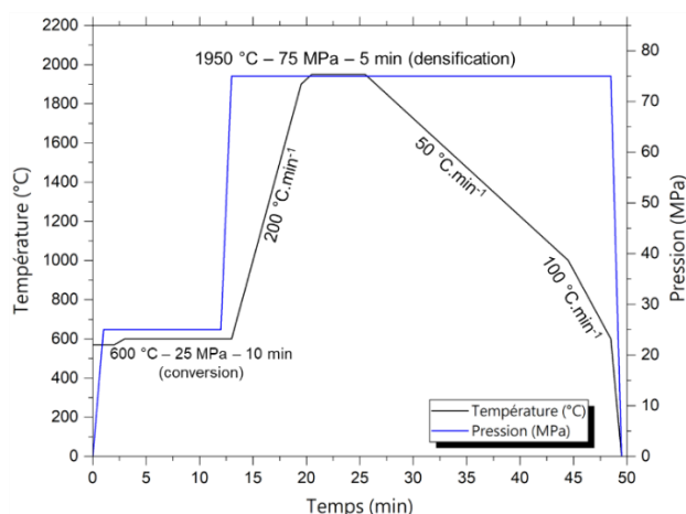
Figure IV.1. Exemple de cycle typique de conversion/frittage
