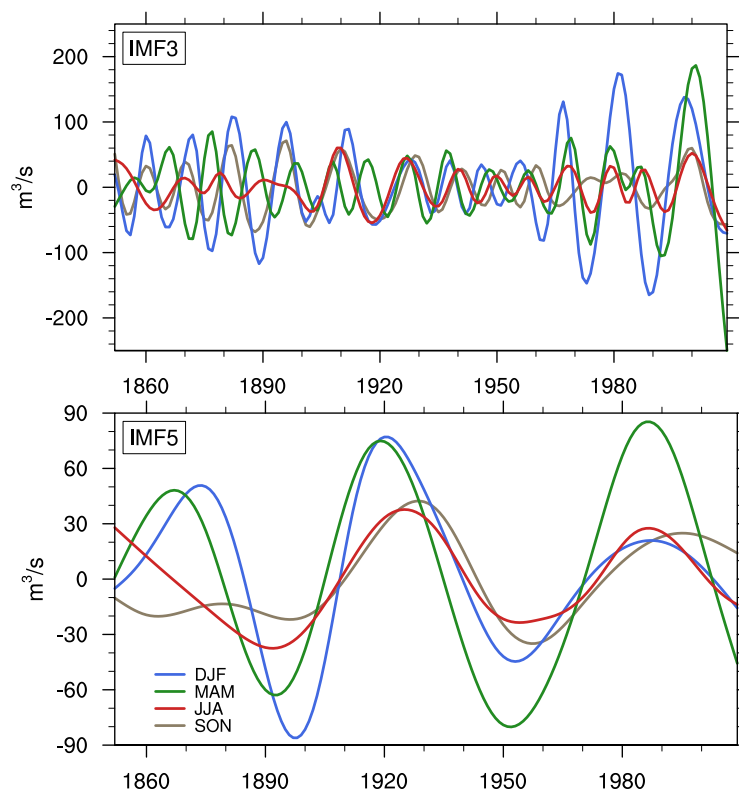
FIGURE 5.3 – Décomposition en modes empiriques d'ensemble (EEMD ; Wu et Huang, 2009) appliqué aux débits saisonniers moyens de la Seine à Poses sur la période 1852-2009. Seules les IMF3 (haut) et 5 (bas), correspondant aux périodes identifiées à partir de l'analyse en ondelette 5.2 ont été représentées en hiver (bleu), au printemps (vert), en été (rouge) et en automne (marron).
