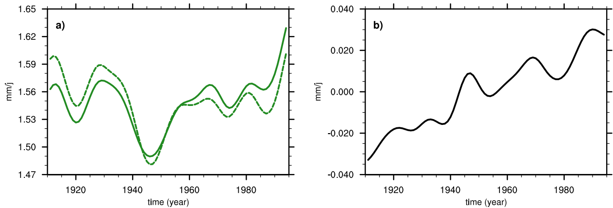
FIGURE 3.4 – (a) Séries annuelles d'évapotranspiration issues de la reconstruction ERA20Cpt (mm/j) (trait plein) et de la reconstruction ERA20Cpt-test (mm/j) (trait pointillé). (b) Différence entre les deux réanalyses. L'anomalie a été calculée sur toute la période.
