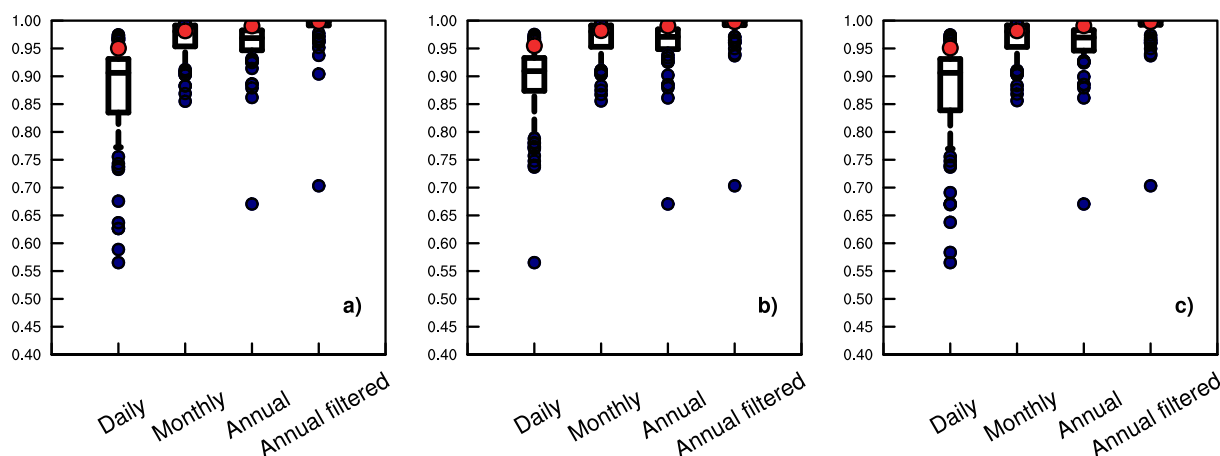
FIGURE 5.13 – Boîtes à moustaches des corrélations des débits calculées entre la reconstruction SEINE-CJM et (a) la simulation Aquif-FR, (b) la simulation Aquif-FR sans prélèvements et sans pertes en rivière et (c) la simulation Aquif-FR sans prélèvements uniquement pour toutes les stations simulées sur le bassin de la Seine. Les corrélations ont été calculées sur la période 1852-2009 pour les débits journaliers, mensuels, annuels et annuels filtrés (à partir d'un filtre de Lanczos avec une fenêtre de 21 ans). Les séries journalières et mensuelles ont été désaisonnalisées avant le calcul des corrélations. Les limites des boîtes à moustaches correspondent au premier décile, au premier quartile, à la médiane, au dernier quartile et au dernier décile. Les points bleus indiquent les stations ayant des corrélations plus faibles (fortes) que le premier (dernier) décile. Les points rouges représentent les corrélations pour la station de la Seine à Poses.
