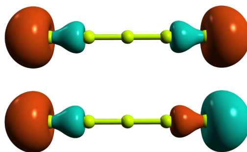
FIGURE A.24: Orbitali magnetici delle catene di berillio.
