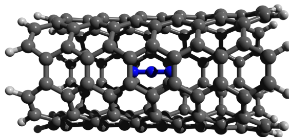
FIGURE A.9: L'anion azoture confiné dans un CNT.
