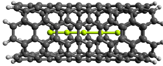
FIGURE A.25: Be 5 confinato in un CNT.
