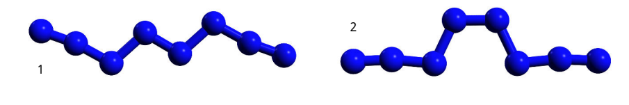
FIGURE A.23: Due isomeri stabili della molecola N_8 .
