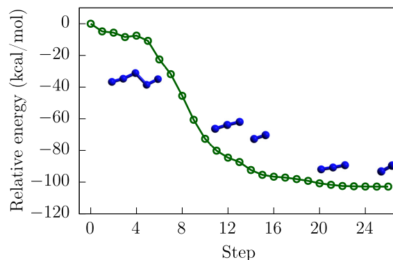
FIGURE A.22: Superficie di energia potenziale della decomposizione dell'ione N_5^+ confinato in un CNT(5,5). Alcune geometrie intermedie sono mostrate lungo la curva senza il nanotubo per una miglior rappresentazione.
