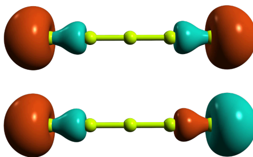
FIGURE A.13: Orbitals magnétiques des chaînes de béryllium.
