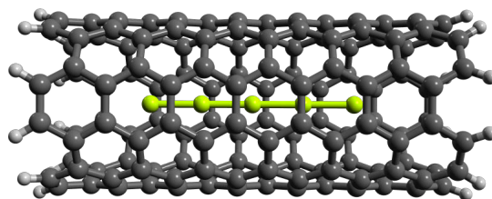
FIGURE A.14: \text{Be}_5 confiné dans un CNT.
