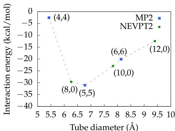
FIGURE A.21: Energie di interazione non rilassate in funzione del diametro del nanotubo.
