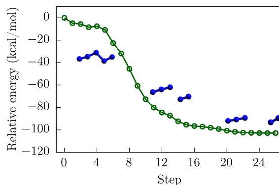
FIGURE A.11: Surface d'énergie potentielle de la décomposition de l'ion N_5^+ . Des géométries intermédiaires sont représentées sans le nanotube pour une meilleure représentation.
