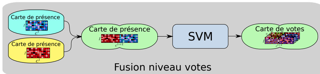
FIGURE 3.6 – Fusion d'informations niveau votes.
