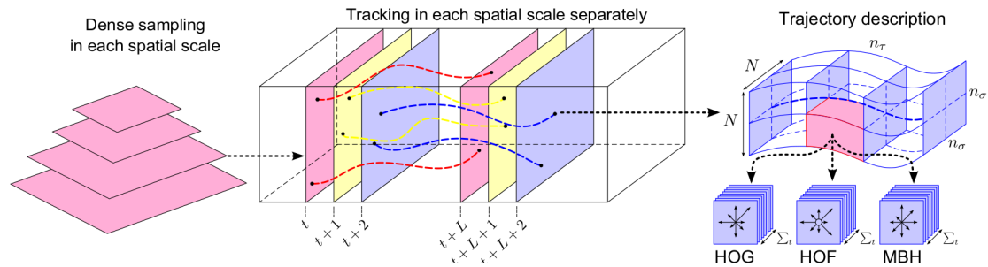
FIGURE 2.5 – Extraction des descripteurs de trajectoires denses, proposée dans [16]. Cette figure est issue de cet article.
