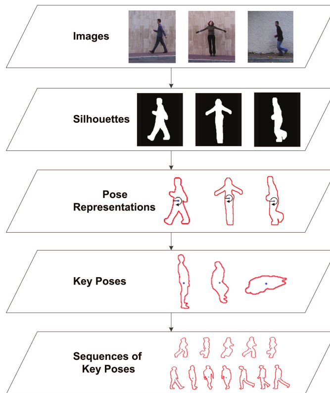
FIGURE 2.1 – Extraction de poses clés issues de la silhouette par [12]
