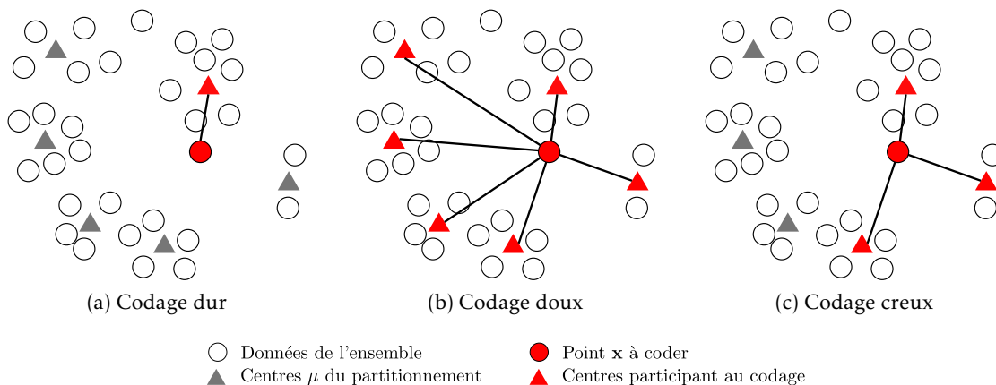
FIGURE 2.11 – Illustration des techniques de codage des descripteurs.
