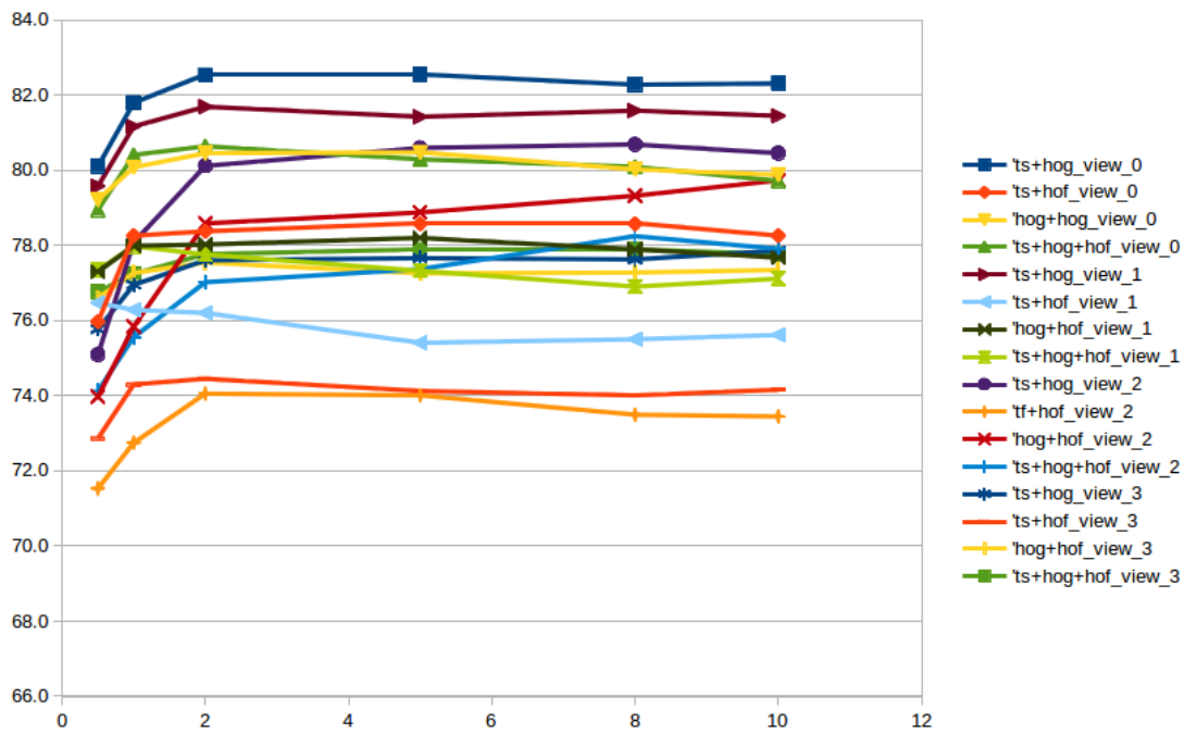
FIGURE 3.12 – Influence du paramètre C (équation 3.8) sur les résultats obtenus par fusion de descripteurs
