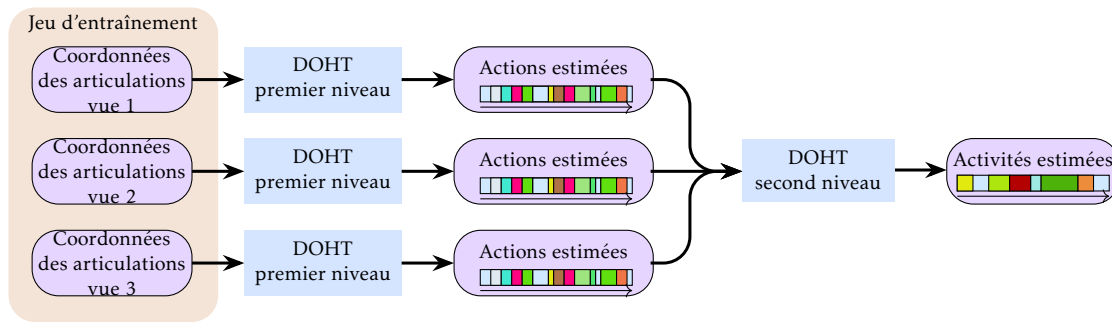
FIGURE 5.11 – Paradigme de fusion des vues en DOHT hiérarchique
