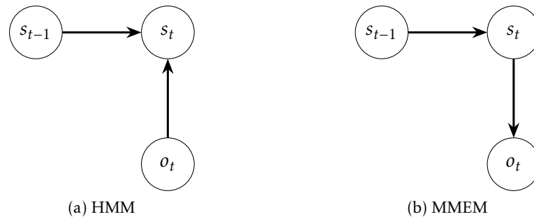
FIGURE 2.15 – Graph de dépendances des méthodes HMM et MMEM [102]
