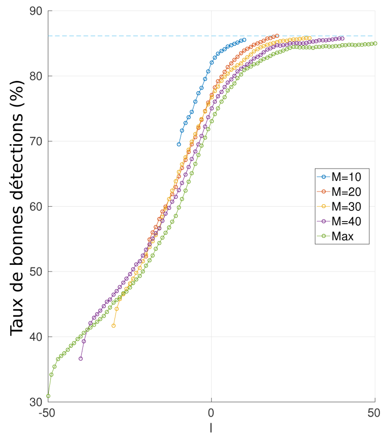
FIGURE 3.14 – Performances de l'algorithme DOHT en fonction de la latence
