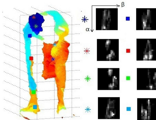
FIGURE 2.8 – Illustration du BSC [42]. \alpha et \beta sont deux composantes d'un vecteur \overrightarrow{PP_0} en coordonnées cylindriques
