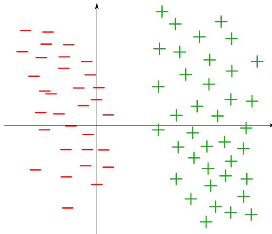
FIGURE 2.12 – Données associées à un label positif ou négatif
