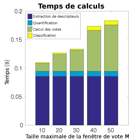
FIGURE 3.16 – Temps de calcul associés au DOHT en fusionnant les informations squelette aux trajectoires denses. Ces temps de calcul sont affichés en fonction de la demi-taille des fenêtres de vote M .
