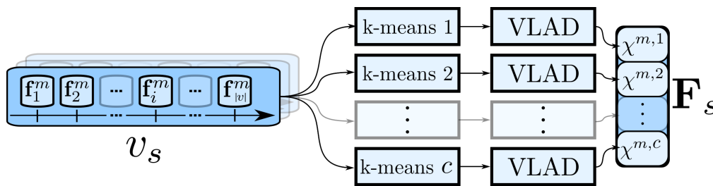
FIGURE 5.7 – Description des segments d'actions élémentaires. En entrée, un segment v_s , en sortie un descripteur \mathbf{F}_s de taille constante au travers des segments v_s
