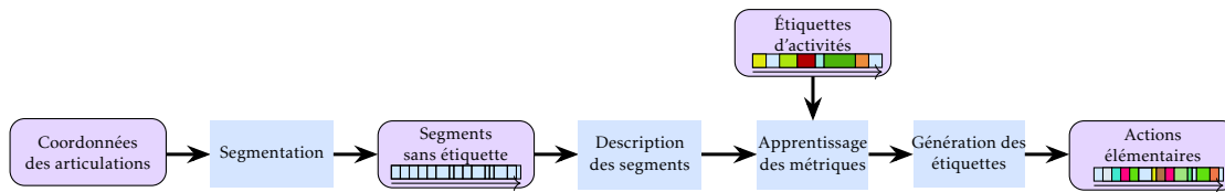
FIGURE 5.2 – Génération semi-supervisée d'actions élémentaires. Seules les activités sont connues, les actions élémentaires sont issues d'une segmentation non-supervisée suivi d'un apprentissage de métrique supervisée par les activités puis d'un regroupement type k-moyennes
