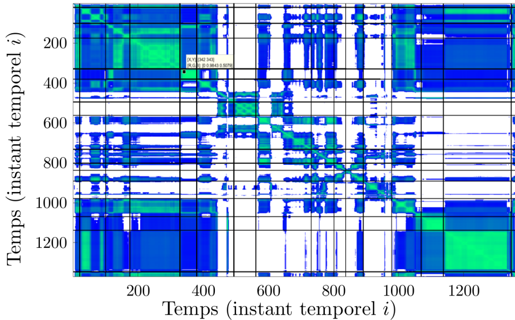
FIGURE 5.5 – Exemple de matrice SSSM obtenue sur DAHLIA
