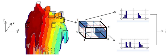
FIGURE 2.7 – Illustration de l'extraction des DCSF à partir d'une succession temporelle de cartes de profondeur. S est le vecteur de similarité calculé à partir de l'ensemble des distances de Batthacharyya entre les sous-blocs. Images extraite de [37].
