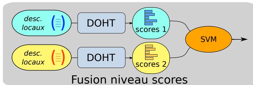
FIGURE 3.7 – Fusion d'informations niveau carte de présence
