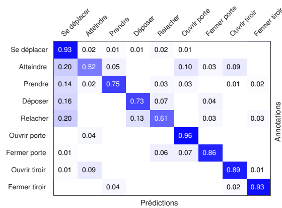
FIGURE 3.13 – Matrice de confusion après fusion au niveau votes des vues 0 et 2 sur le jeu de données TUM [126]
