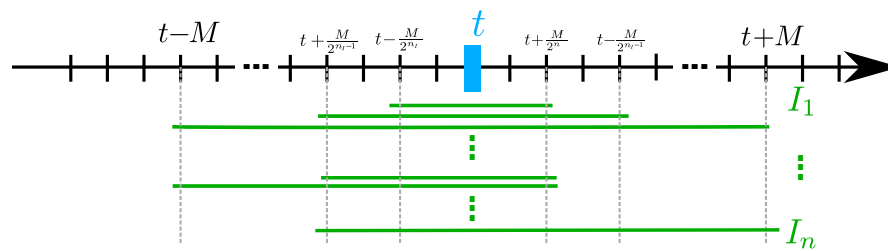
(b) Sous-ensemble considéré dans la version du DOHT approximé \mathcal{J}^{partiel}
