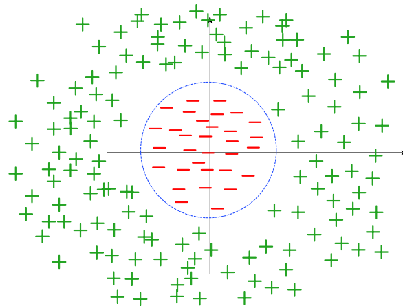
FIGURE 2.14 – Cas de données non séparables linéairement
