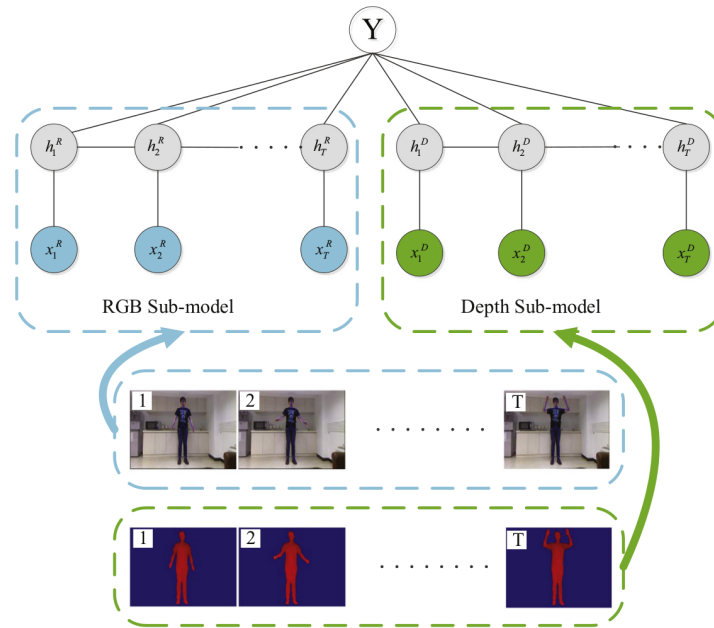
FIGURE 2.16 – Structure des HCRFs couplés (cHCRF), image extraite de [111]
