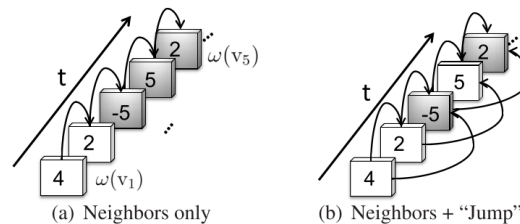
FIGURE 4.12 – Illustration des deux stratégies proposées par [171]. Chaque rectangle est un nœud et les chiffres représentent les poids associés à ces nœuds.
