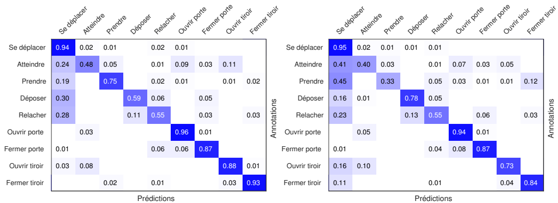
(a) Fusion de descripteurs (TS+HOG) sur la vue 0. (b) Fusion de descripteurs (TS+HOG) sur la vue 2.
