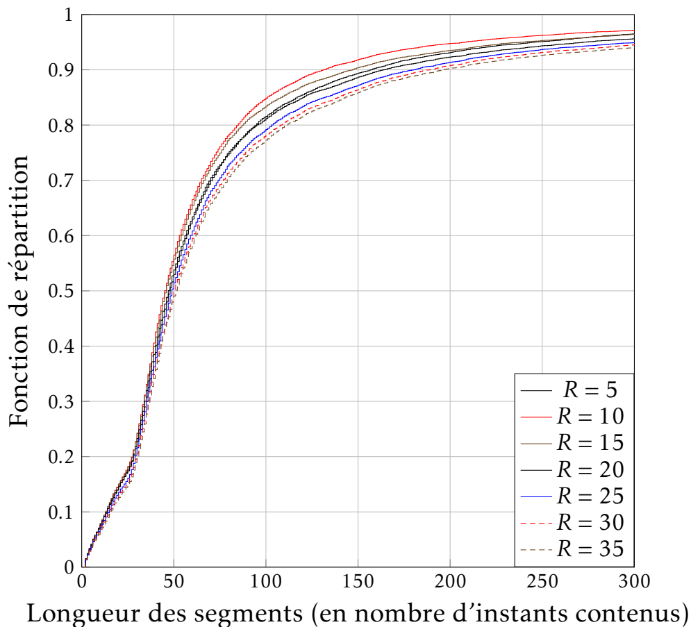
FIGURE 5.9 – Fonction de répartition empirique des longueurs des segments
