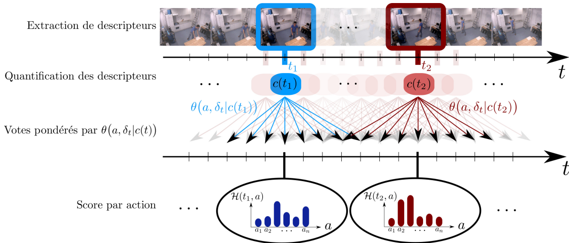
FIGURE 3.1 – Illustration d'un algorithme de détection d'actions par transformée de Hough. Sur cette figure sont représentés les votes engendrés aux temps t_1 et t_2 ainsi que l'accumulation des votes pour chaque action à ces instants.
