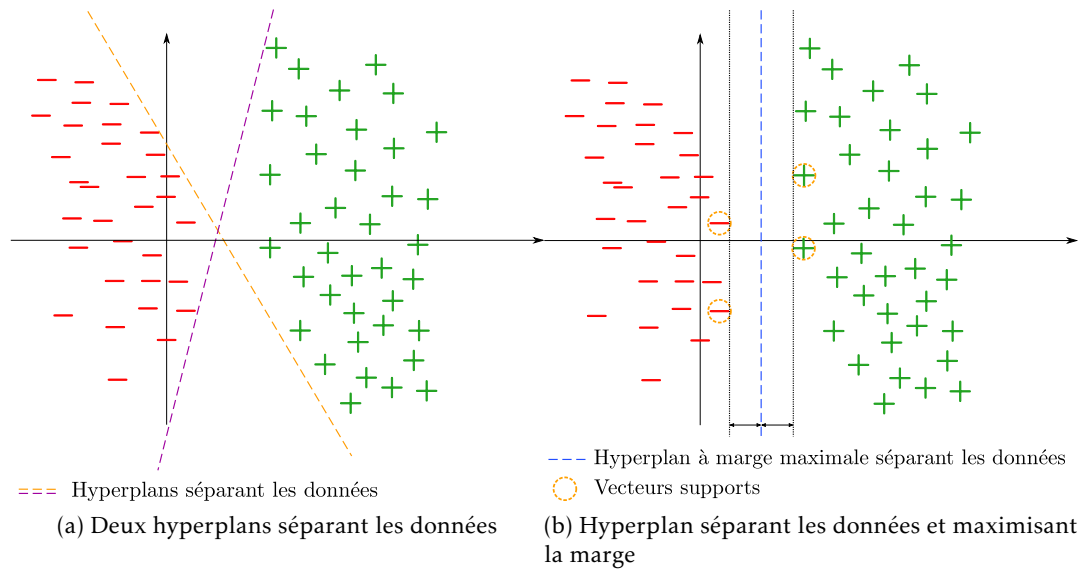
FIGURE 2.13 – Séparation de données par un hyperplan
