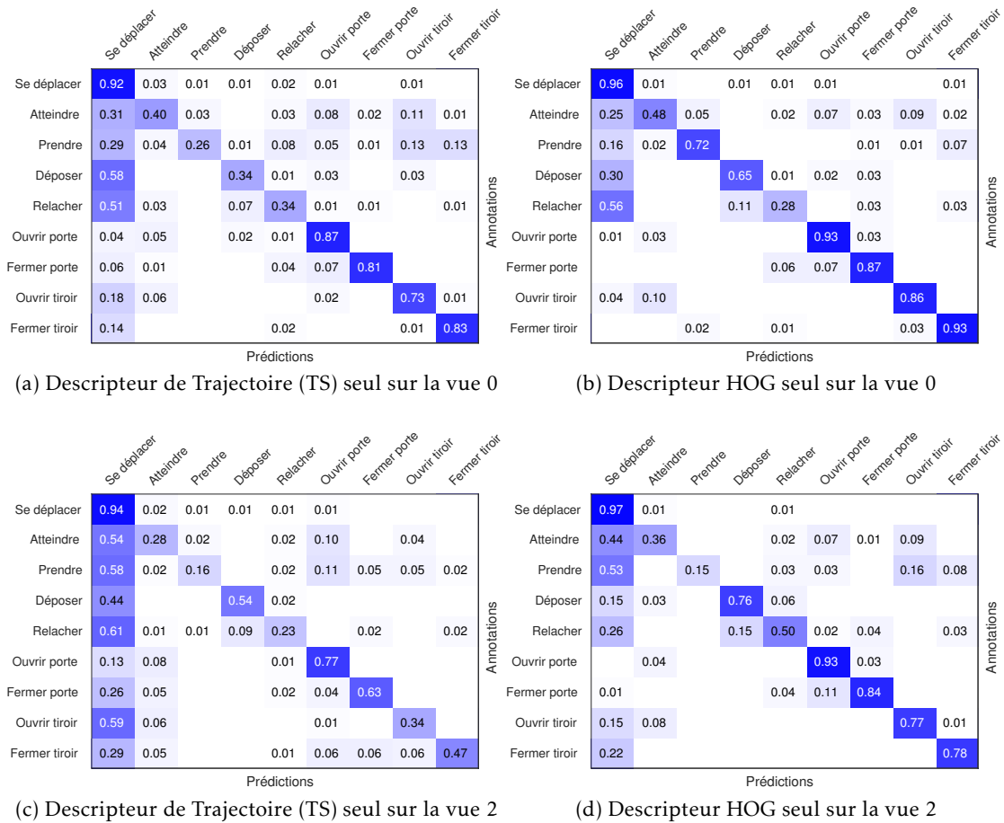
FIGURE 3.10 – Matrices de confusion sur le jeu de données TUM [126] en évaluation mono-descripteur sur les vues 0 et 2
