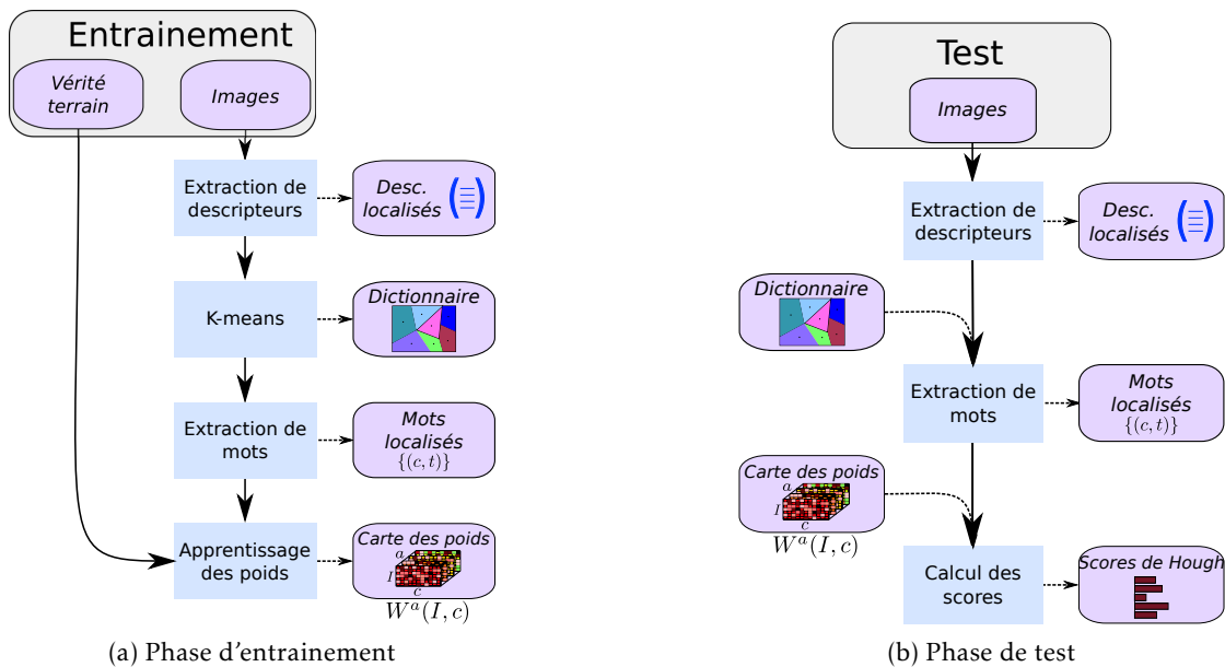
FIGURE 3.4 – Illustration de l'algorithme DOHT
