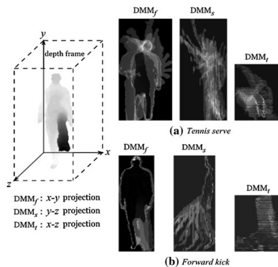
FIGURE 2.9 – Illustration des DMM utilisées dans [44]. Image extraite de cet article.
