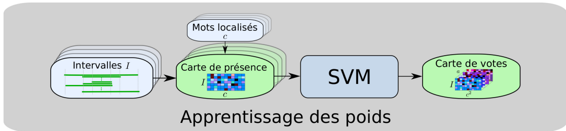
FIGURE 3.3 – Apprentissage des poids au sein du DOHT
