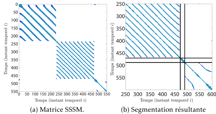
FIGURE 5.4 – Illustration de l'algorithme de segmentation en actions élémentaires. Figures extraite de [175]
