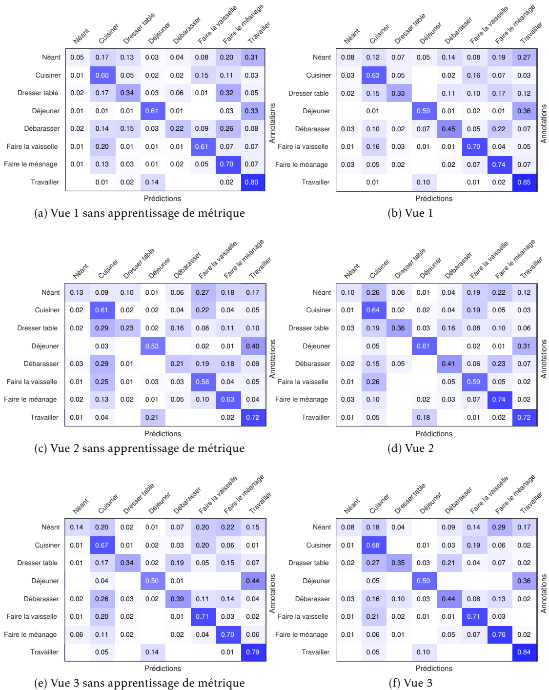
FIGURE 5.12 – Matrices de confusion obtenues avec le DOHT hiérarchique, avec et sans étape d'apprentissage de métrique
