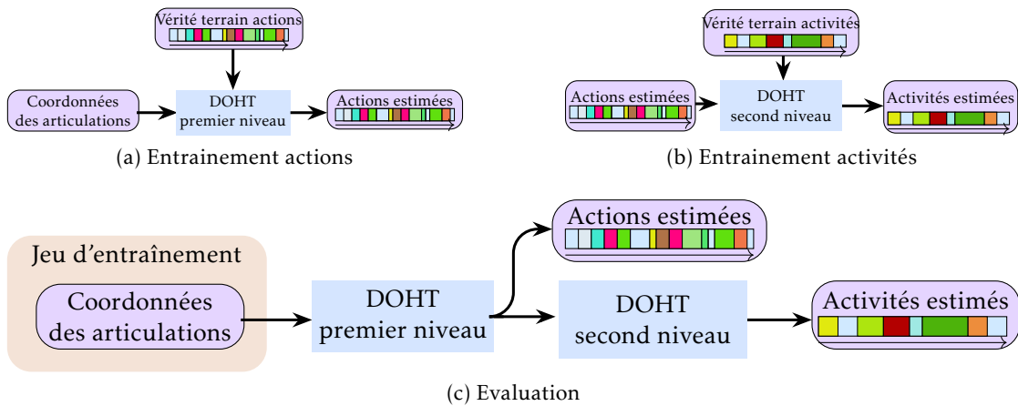
FIGURE 5.1 – Détection hiérarchique d'activités
