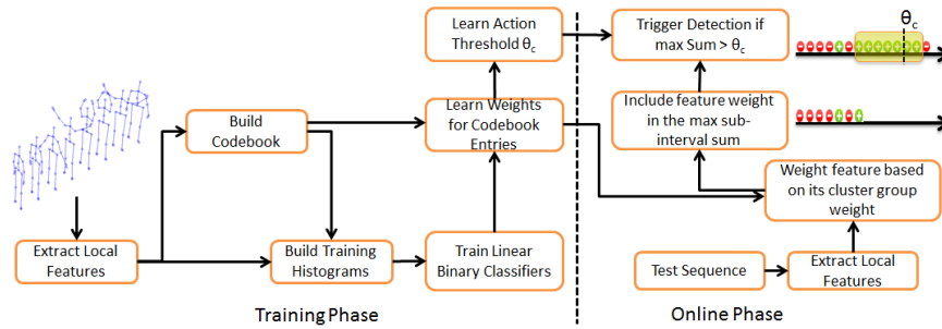
FIGURE 4.11 – Illustration de la méthode ELS [170]. Image extraite de l'article original.
