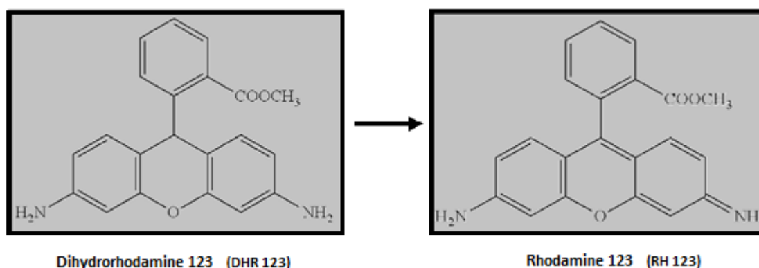
Figure 26: Schéma d'oxydation de DHR 123 en RH 123
