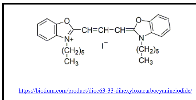
Figure 27 : Structure chimique du DiOC 6 (3) (3,3'-dihexyloxycarbocyanine iodide)
