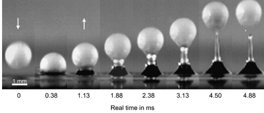
Fig. 3.11 Images de l'impact d'un grain d' \text{Al}_2\text{O}_3 arrivant à une vitesse de 2,36 \text{ m.s}^{-1} sur une surface lisse recouverte d'un film d'eau d'épaisseur 400 \mu\text{m} , issus de Antonyuk et al. [159].
