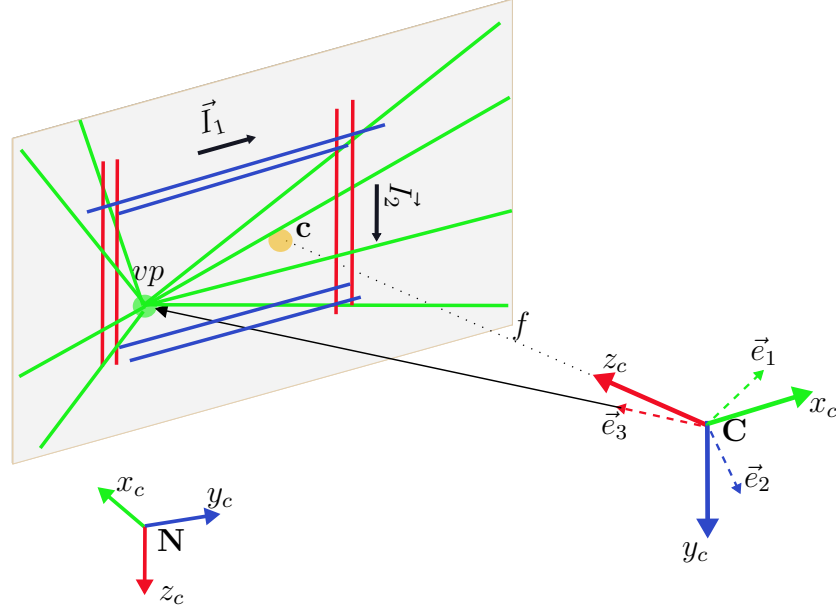
Figure 5 – Estimation de point de fuite fini.
