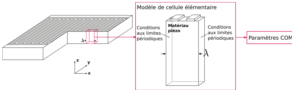
Figure ii Cellule élémentaire utilisée pour calculer les paramètres COM.
