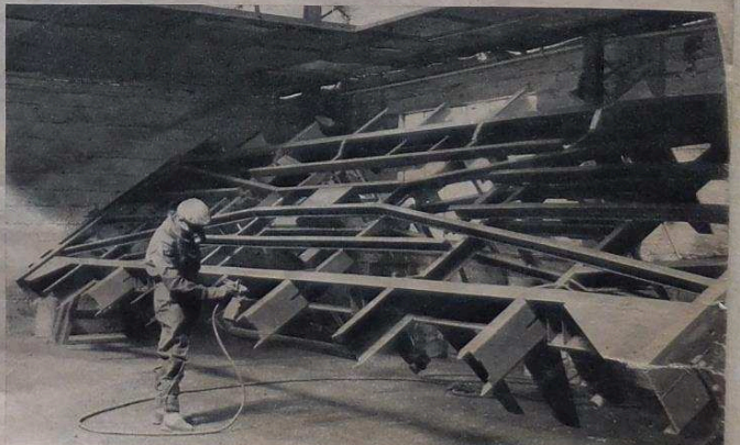
Application au pistolet d'une deuxième couche de peinture. Le châssis est monté sur positionneur tournant.
