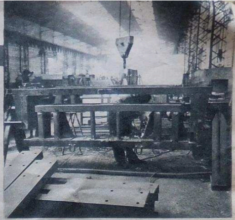
On ajoute au châssis une plate-forme de 500 mm permettant le dégagement du « garage ».
