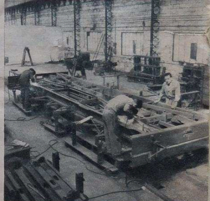
Montage des éléments du châssis type UIC, sur mannequin.
