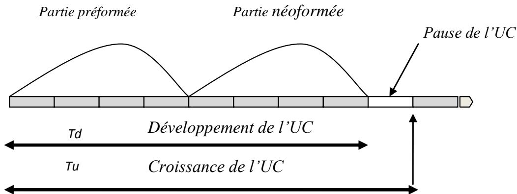
Figure 18: Schéma de développement et croissance de l'UC d'une pousse annuelle bicyclique de Teck dans le modèle GreenLab
