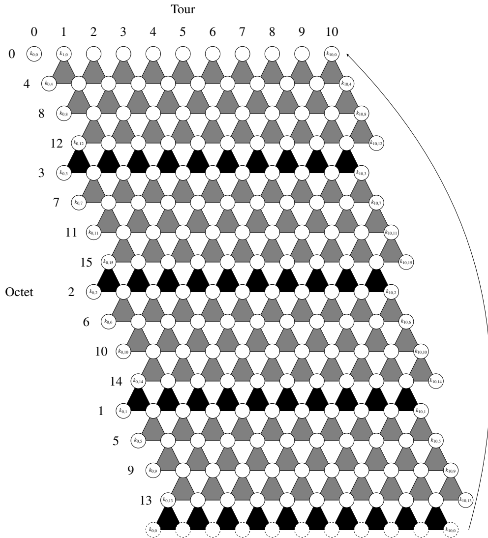
FIGURE 1.7 – Hypergraphe représentant les dépendances du key schedule
