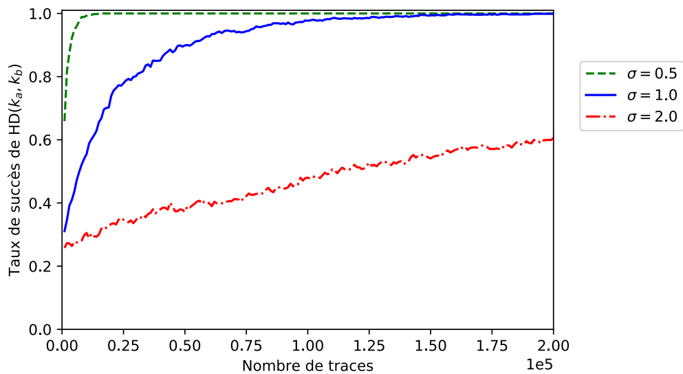
FIGURE 3.25 – Taux de succès d'attaque m_x quadrivariée pour différents niveaux de bruit
