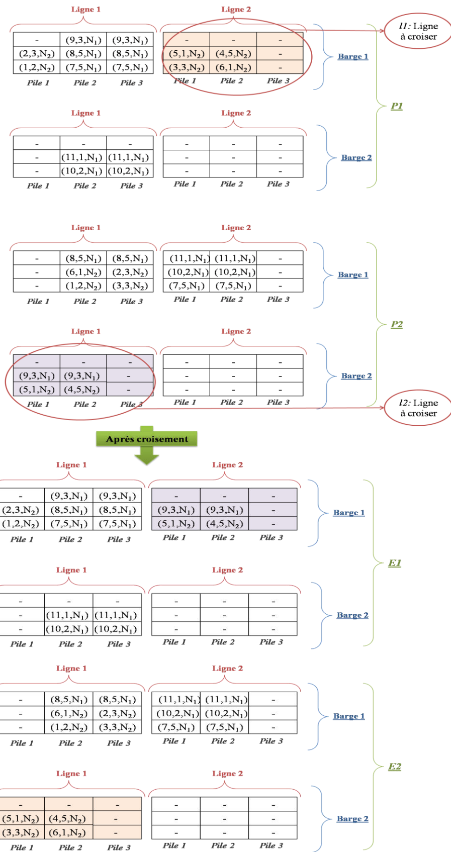
Figure IV-15. Fonctionnement de l'opérateur croisement proposé pour le 3D-CCSPP
