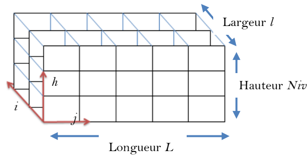
Figure III-3. Structure cellulaire générale d'une barge à conteneurs
