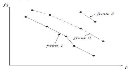
Figure IV-13. Illustration des fronts de Pareto dans un problème de minimisation bi-objectifs
