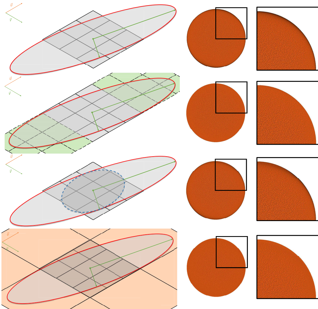
FIGURE 3.5 – Ligne du haut: Dans des cas extrêmes, l’empreinte de pixel (en rouge) peut devenir plus grande que le voisinage considéré pendant l’évaluation (en gris). Si les cellules manquantes ne sont pas prises en compte, la convolution n’est pas calculée correctement (les régions sombre sur les bordures de la sphère). Deuxième ligne: La solution correcte est de considérer toutes les cellules intersectant l’empreinte de pixel lors du calcul. Cependant, cela devient rapidement impraticable pour du temps réel. Troisième ligne: En pratique, l’empreinte de pixel est généralement limitée au voisinage considéré (en bleu), ce qui réintroduit de l’aliasage dans certains cas. Dernière ligne : Une meilleure solution pratique est de précalculer une tuile représentative du voisinage et faire une transition douce entre le filtrage analytique et cette représentation mipmappée .
