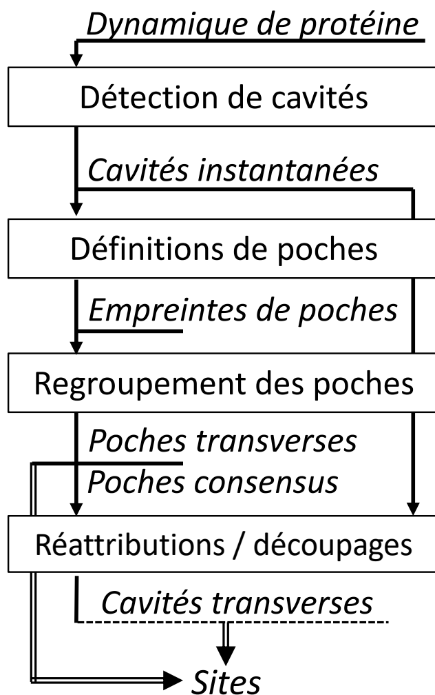
Figure IV.2 Étapes du suivi des cavités pour la détection de sites. Les routines sont représentées dans des boîtes, les données en italiques .
