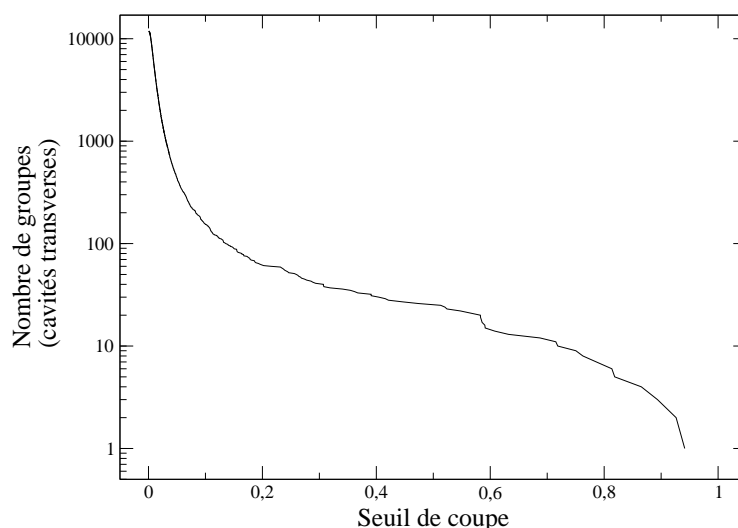
Figure IV.6 Nombre de groupes obtenus en faisant varier le paramètre de coupe lors du partitionnement. Obtenu par un partitionnement hiérarchique avec lien moyen des empreintes de cavité de la myoglobine.
