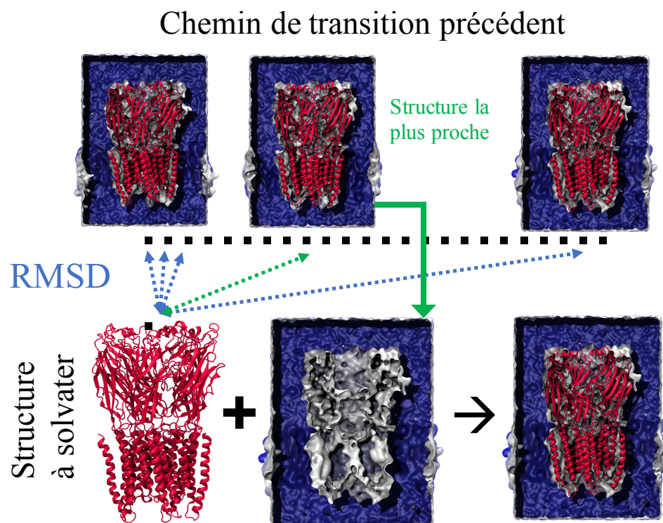
Figure III.3 Réutilisation de boîtes solvatées pré-équilibrées. La structure à solvater est insérée (copie des coordonnées atomiques) dans la boîte solvatée contenant la conformation la plus proche (RMSD minimal). Après minimisation et équilibration suffisante, le système est prêt à être utilisé par les String of Swarms .
