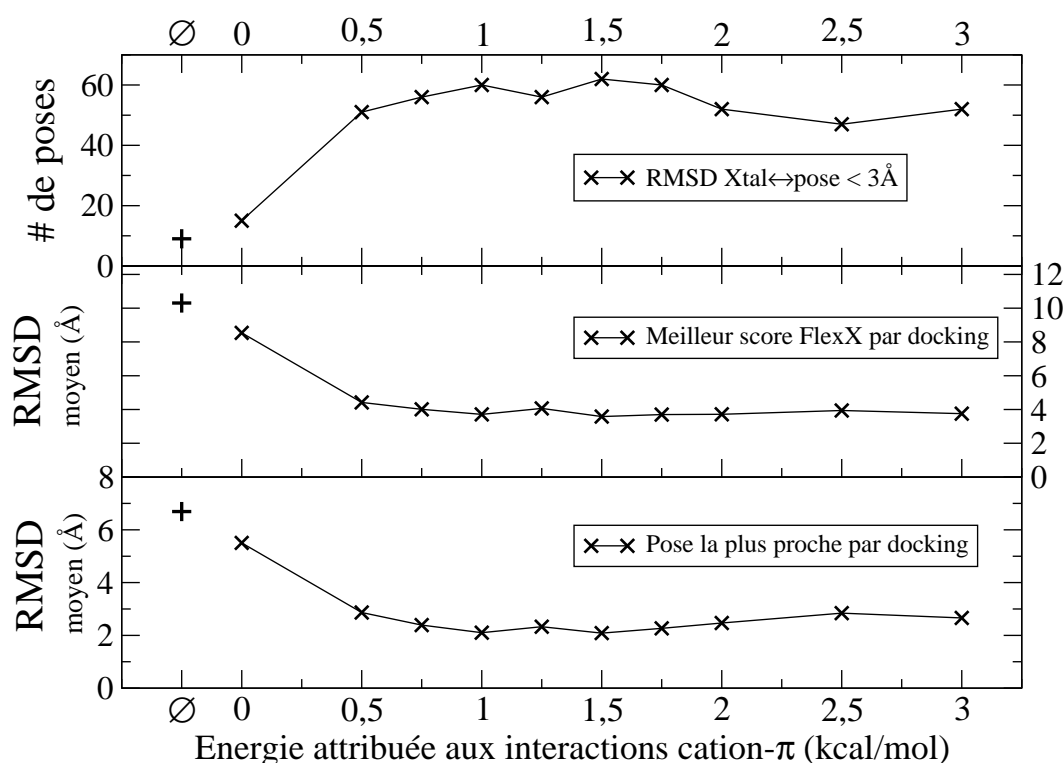
Figure V.2 Qualité des poses de docking en fonction de la contribution énergétique associée à l'interaction cation- \pi . L'abscisse \emptyset est associée à une configuration de FlexX dépourvue de l'interaction cation- \pi alors que pour l'abscisse 0 l'interaction existe et a une énergie associée nulle. Graph 1 : Nombre de poses (/160) dont le RMSD à la pose cristallographique associée est inférieur à 3 Å. Graph 2 (resp. 3) : RMSD moyen sur les 16 dockings , de la pose de meilleur score FlexX (resp. de la pose la plus proche de la pose cristallographique) par rapport à la pose cristallographique.
