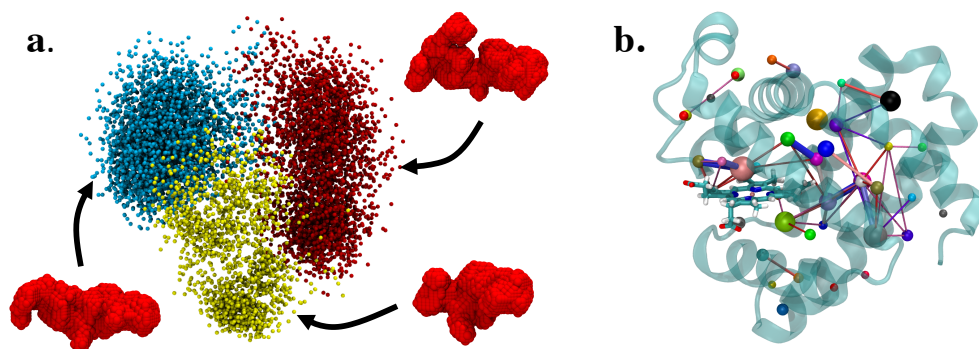
Figure IV.17 Exemples d'analyse de la dynamique des cavités. a. Sélection de poches à la géométrie diverse. L'ensemble des cavités d'un même site est extrait d'une trajectoire moléculaire. Une analyse en composantes principales sur la géométrie des cavités [9] permet d'extraire les principaux modes de variation des volumes considérés. Après projection (ici sur les 3 premiers modes d'une analyse en composantes principales), les cavités peuvent être triées en différents groupes par similarité de forme. La sous-sélection de cavités représentatives de chacun de ces groupes (critères énergétiques et autres) simplifie la prise en compte exhaustive de la dynamique du site, par exemple, pour réaliser une campagne de criblage virtuel par docking moléculaire. b. Analyse du réseau de cavités de la myoglobine. Un suivi des cavités avec découpage permet de discerner deux cavités présentes dans des sites distincts mais spatialement jointes. Un graphe dont les nœuds représentent chaque site et dont les arrêtes sont pondérées par le nombre d'évènements de fusion entre les sites peut alors être construit (cf. les billes et les tubes dans la figure). Sur de longues dynamiques de protéine il devient possible, par exemple, de mesurer la probabilité d'accessibilité d'une poche enfouie avec le solvant extérieur.
