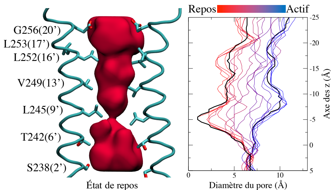
Figure III.9 Constriction du pore observée pour la dernière itération des Swarms de la série S4. Le volume du canal de la structure stable au repos (80 % de la réaction) est représenté en surface rouge à gauche. La numérotation des résidus est propre à nos modèles \alpha 7 et une numérotation consensuelle est donnée entre parenthèses (numérotation de l'hélice M2 de C.Miller [169]). À droite, les profils de diamètre du pore en fonction de l'axe des z, calculées avec mkgridXf, et tiennent compte du rayon de Van der Waals des atomes. Les structures stables repos et actifs (20 % et 80 % de la réaction) sont surlignées en noire.
