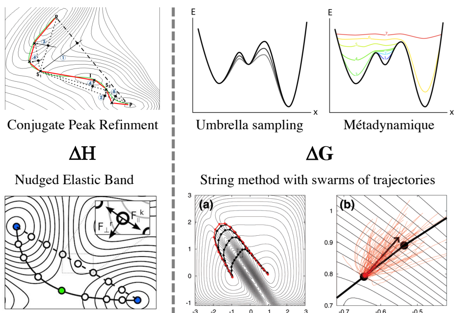
Figure 1.4 Exemples de méthodes pour le calcul de chemins de transitions. À gauche, méthodes adiabatiques pour le calcul de chemin d'énergie minimum : Conjugate Peak Refinement et Nudged Elastic Band . À droite, méthodes dynamiques pour le calcul de chemin d'énergie libre : Umbrella Sampling , Métadynamique , et String method with swarms of trajectories .
