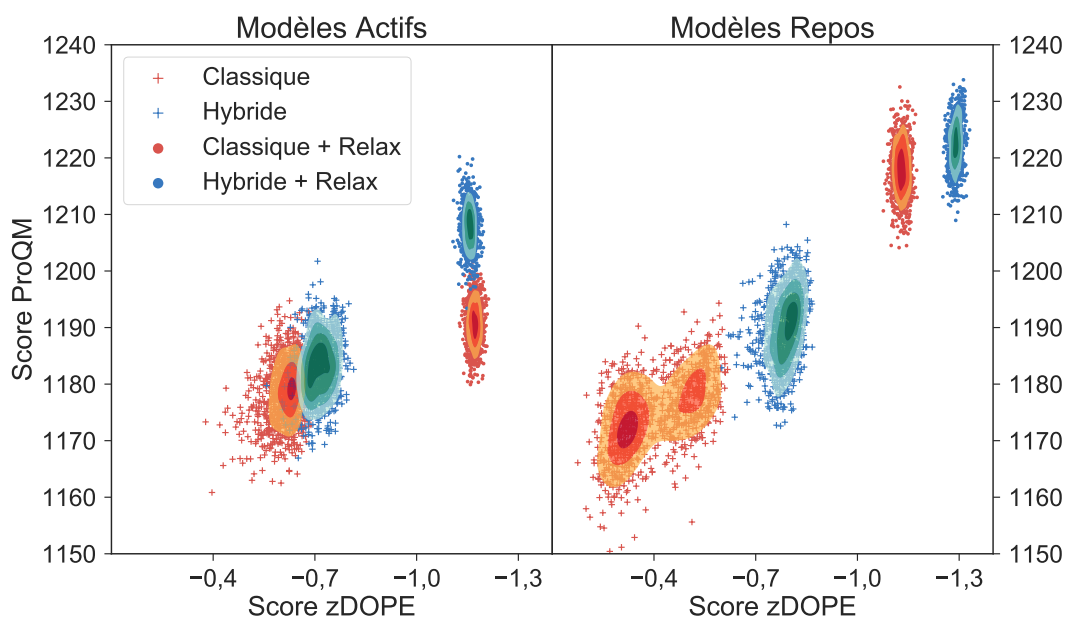
Figure II.6 Distribution des scores ProQM et zDOPE de modèles classiques et de modèles utilisant l'approche hybride. Les meilleurs scores de qualité sont vers le haut pour le score ProQM et vers la droite pour le score zDOPE. Les deux ensembles représentés par des points correspondent aux raffinements des “meilleurs” candidats des structures représentées par des croix. Le raffinement est réalisé par le script “Rosetta Membrane Relax” [92] et produit un ensemble de 1 000 nouveaux modèles.
