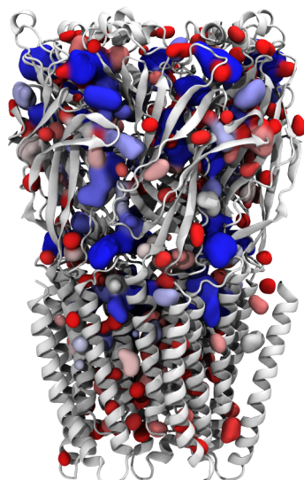
Figure IV.15 Cavités moyennes et leur pourcentage d'apparition. Le pourcentage d'apparition des cavités moyennes (seuil à 25 %) des 68x5 cavités transverses détectées le long de la transition est renseigné par un gradient de couleur de rouge (0 %) à bleu (100 %).
