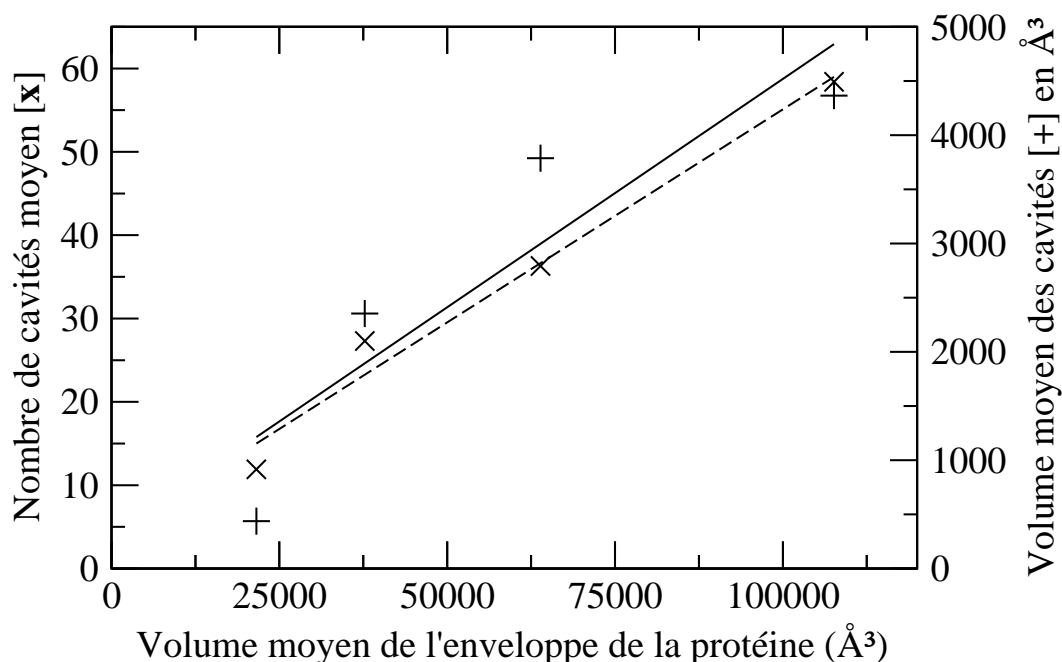
Figure IV.4 Statistiques de la dynamique des cavités. Nombre de cavités moyen par conformation (×) et volume moyen des cavités (+) en fonction du volume moyen de la protéine. Les régressions linéaires sont respectivement tracées en traits hachurés et pleins.
