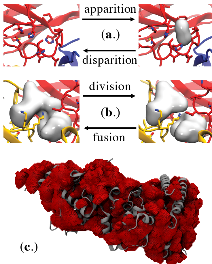
Figure IV.1 Difficultés d'attribution d'une définition consensus pour un site.. a. Apparition ou disparition d'une cavité lorsque sa géométrie atteint un seuil, par exemple, un volume minimum ou le solvant extérieur ( bulk solvent ). b. Fusion ou division de cavités induite par le mouvement subtil d'un acide aminé. c. Domaine de définition des cavités. Les cavités apparaissent labiles et omniprésentes dans les dynamiques de protéines.
