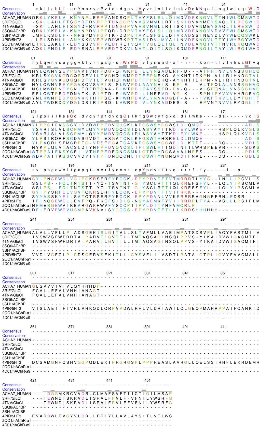
Figure VII.2 Aligement multiple des séquences templates avec la séquence \alpha 7 cible.
