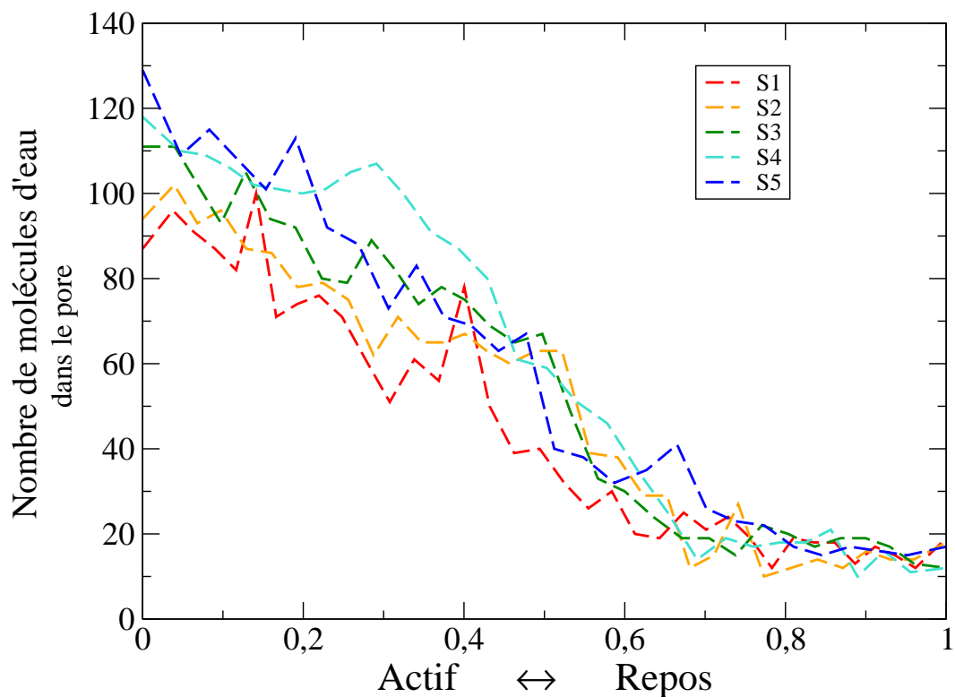
Figure VII.3 Hydratation du canal pour les dernières itérations de String of Swarms. L'hydratation du canal est calculée en comptant les molécules d'eau présentes dans le pore du récepteur. La région considérée pour le comptage correspond à un cylindre de 10 Å de rayon et de 25 Å de longueur, centré au milieu des 5 hélices transmembranaires M2 du récepteur ((x,y,z)=(0;0;-7,5)).
