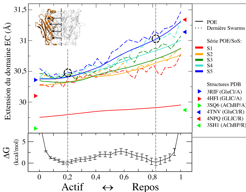
Figure III.10 Extension du domaine extracellulaire le long des modèles de transition. Les transitions POE sont représentées en traits pleins, les dernières itérations de SoS en traits pointillés. Les valeurs comparatives observées dans les structures cristallographiques de récepteurs homologues sont reportées en triangles. Les structures stables de la série S4 (20 % et 80 % de la réaction) sont pointées par des cercles pointillés noirs. Le profil d'énergie libre pour la transition S4 est aligné avec les profils d'extension.
