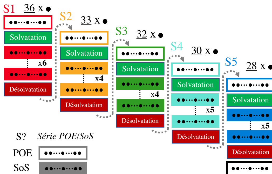
Figure III.4 Plan de simulation pour le couplage POE-SoS. Chacune des 5 colonnes schématise le passage d'un chemin de transition par "Path Optimization and Exploration" (POE) suivie de plusieurs itérations (nombres en gras) de la "String method with Swarms of Trajectories" (SoS). Le nombre de structures intermédiaires des chemins est déterminé par POE (nombres soulignés) et ne varie pas lors des itérations de SoS. Une étape de solvatation et de désolvatation (eau/ions/lipides) encadre chacune des itérations des String of Swarms .
