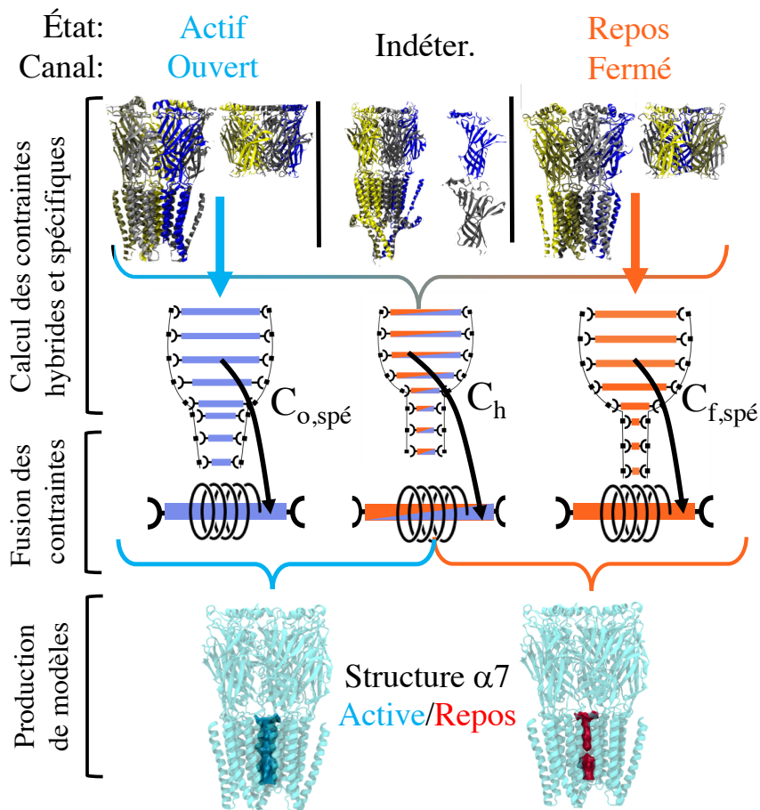
Figure II.5 Approche de modélisation hybride. Les contraintes structurales sur les atomes du récepteur \alpha 7 sont calculées à partir de l'ensemble des templates . Ces contraintes sont dites hybrides ( C_h ). D'autre part, deux autres ensembles de contraintes sont calculés à partir des templates ouverts ( C_o ) et fermés ( C_f ). Ces contraintes C_o et C_f sont alors comparées et triées pour déterminer un sous-ensemble de contraintes spécifiques à la conformation ouverte C_{o,spé} ou fermée C_{f,spé} du récepteur. Finalement, la fusion des contraintes hybrides et des contraintes spécifiques ouvertes/fermées permettent de générer des modèles du récepteur dans ses états actifs ou de repos.
