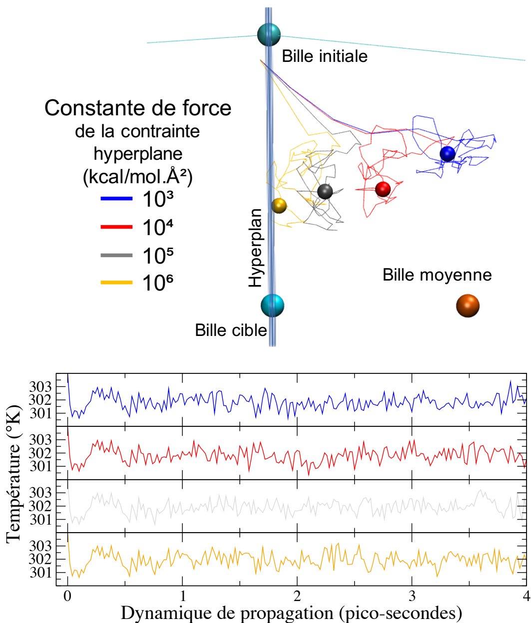
Figure VII.7 Paramétrisation de la contrainte hyperplane. Plusieurs constantes de force ont été testées pour évaluer sa capacité à contraindre les structures de propagation dans l'Hyperplan bissecteur. En haut, la projection de l'ensemble des structures de trajectoires de propagation, sur une analyse en composantes principales calculée sur le triplet de structures (bille initiale, bille cible, bille moyenne). L'hyperplan (de dimension 26 294) est directement visualisable, dans le plan orthogonal à la page et passant par la bille initiale et la bille cible. Ainsi sur la figure, l'éloignement des billes colorées de la ligne représentant l'hyperplan est directement relié au relâchement de la contrainte hyperplane. En pratique, nous avons choisi la contrainte la plus forte ( 10^6 \text{ kcal/mol.Å}^2 ), en vérifiant qu'elle ne déstabilisait pas la dynamique de propagation. Les 4 dynamiques de propagations ont été lancées avec la même graine aléatoire, et un coefficient de friction nulle sur les atomes lourds.
