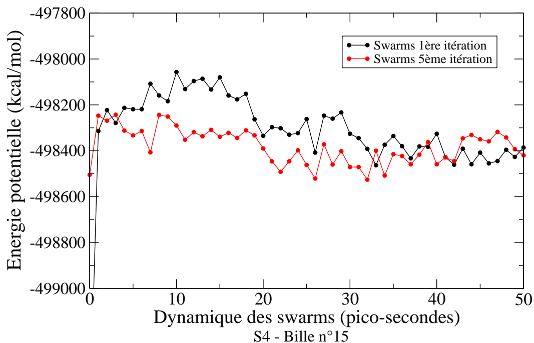
Figure VII.5 Détermination de la longueur des trajectoires de Swarms. Moyenne de l'énergie potentielle des 32 trajectoires non contraintes de Swarms mesurée toutes les pico-secondes (Série S4, bille 15, pour la 1 re et la 5 e itération de SoS). Les dynamiques de Swarms ont été rallongées à 50 ps pour évaluer un temps suffisant à la relaxation des billes. Les trajectoires atteignent un plateau énergétique entre 20 et 30 ps. En pratique, cette durée a été placée à 20 ps. En début de trajectoire la courbe rouge (5 e itération SoS) apparaît être plus stable énergétiquement que la courbe noire (1 re itération SoS, sortie de POE), ce qui est en accord avec une diffusion de la bille 15 dans un minimum du paysage d'énergie libre.
