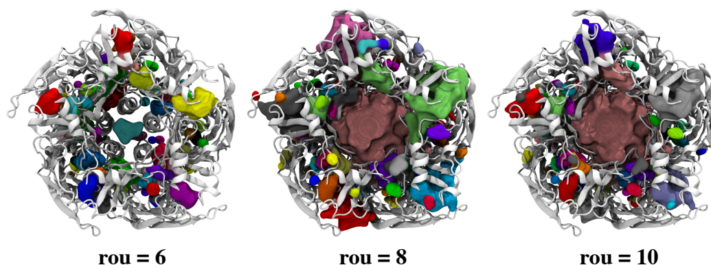
Figure IV.13 Effet du paramètre rou lors de la détection des cavités. Les cavités détectées dans cette conformation (canal en état fermé) ont été calculées avec une valeur du rou égale à 6, 8 et 10 Å. La variation du rayon de la grande sphère de détection de cavités ronge plus ou moins la cavité centrale et segmente les cavités à la surface du pore.
