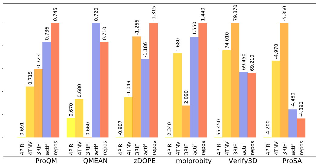
Figure II.7 Évaluation des structures selon diverses fonctions de score. Les modèles ouverts et fermés issus de l'approche hybride sont comparés aux structures cristallographiques utilisées comme templates . Pour chaque fonction de score utilisée, le moins bon score parmi les structures évaluées a une hauteur d'histogramme nulle alors que le meilleur score à une hauteur maximale.
