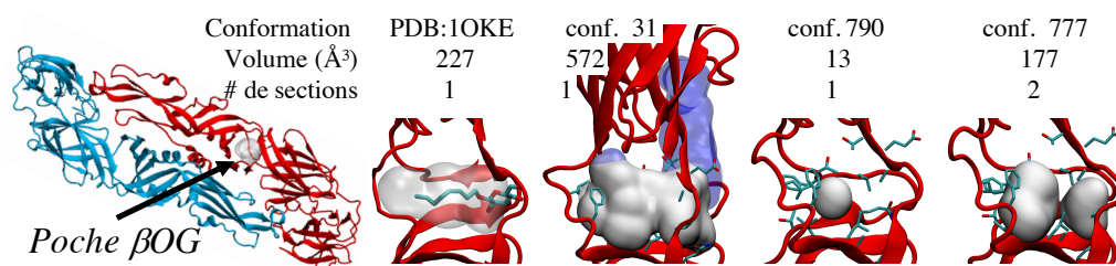
Figure IV.10 Diversité des géométries de cavités. Site \beta OG (volume gris, chaîne A de la protéine E de la dengue). La molécule \beta OG est montrée en sticks dans la structure 1OKE (en transparence de la cavité). Les volumes et nombre de morceaux des cavités de référence sont exprimés. Un exemple de fusion d'une cavité instantanée entre plusieurs sites est montré dans la conformation 31 (bleu transparent). En comparaison, la cavité de référence est confinée dans son site de référence.
