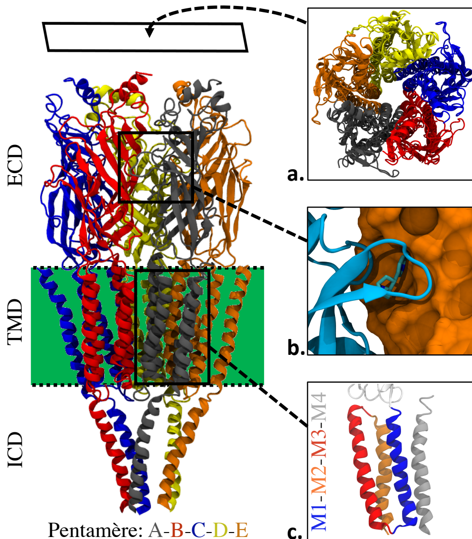
Figure 1.2 Structure tridimensionnelle du récepteur nicotinique. À gauche, vu transversale de la structure du récepteur nicotinique de type musculaire de Torpedo Marmorata (PDB : 2BG9), colorée selon ses différentes sous-unités. ECD, TMD, ICD identifient respectivement les domaines extracellulaire, transmembranaire et intracellulaire. a. vu de dessus, le pore perméable aux ions est au centre. b. poche orthostérique du récepteur \alpha 7 (chimère AchBP Lymnaea stagnalis , PDB : 3SQ6) liée à l'agoniste épibatidine. La sous-unité principale (boucle C), est en représentation Cartoon, et la sous-unité complémentaire en surface orange. c. Zoom sur les 4 hélices transmembranaires d'une des sous-unités du récepteur, colorées selon les différentes hélices.
