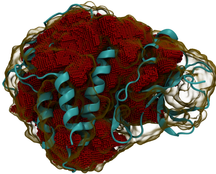
Figure IV.5 Domaine de définition des cavités de la plus large composante connexe du graphe séquentiel. Pour la trajectoire ab11 (points rouges) le volume couvert représente 67,1 % du domaine de définition de l'ensemble des cavités qui apparaissent au cours de la trajectoire (surface transparente).
