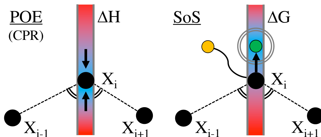
Figure III.5 Compatibilité technique entre POE et SoS. En gris, l'hyperplan bissecteur des vecteurs formés entre la structure courante ( X_i ) et ses 2 structures adjacentes ( X_{i-1} et X_{i+1} ). À la fin de POE, chacune des structures du chemin est dans un minimum énergétique local dans son hyperplan (contexte \Delta H ). Lorsque le chemin est plongé dans le contexte d'énergie libre avec la méthode des String of Swarms , ce même hyperplan est utilisé pour laisser diffuser la structure dans un minimum d'énergie libre ( \Delta G ) et garantir que les structures intermédiaires restent au même stade d'avancement de la réaction. En bille jaune, la structure moyenne des trajectoires de Swarms et en vert la structure cible, projection de la bille moyenne dans l'hyperplan.
