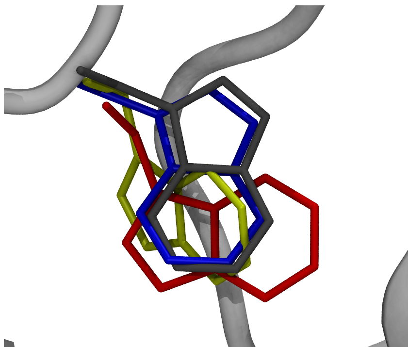
Figure II.9 Ambiguïté locale des templates . Orientation du résidu TRP146 dans la poche orthostérique du modèle \alpha 7 en état actif (résidu jaune). Les tryptophanes du template AChBP (3SQ6-TRP145) sont en bleu et 5HT 3 (PDB :4PIR-TRP156) en rouge et d' \alpha 4\beta 2 (5KXI-( \alpha 4 )TRP156) en gris. Le squelette de la structure 3SQ6 est représenté en cartoon blanc. L'alignement des résidus a été réalisé par alignement structural de la chaîne A des 3 structures grâce au module MultiSeq de VMD.
