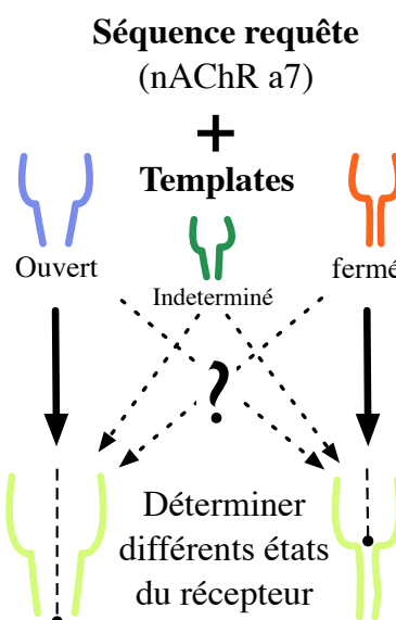
Figure II.2 Problématique de la modélisation d'états conformationnels. L'approche classique de modélisation par homologie n'utilise que les templates dont la conformation correspond à celle à modéliser (flèches pleines). L'approche hybride (flèches pointillées) cherche à utiliser l'ensemble des templates disponibles en triant lors de la modélisation les contraintes dictant la structure globale du récepteur.
