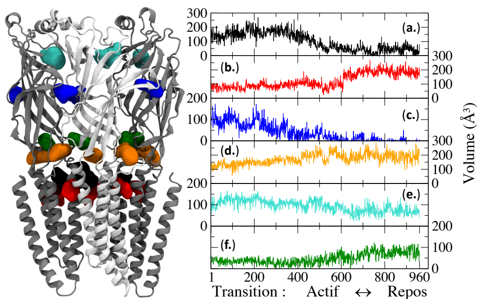
Figure V.7 Sous-ensemble des sites évoluant le plus avec le changement conformationnel. À gauche, cavité moyenne (tronquée à 0,25) de chacun des sites sélectionnés. À droite, volumes des différents sites (moyenné sur les 5 poches symétriques), en fonction du pas de trajectoire (fermeture du canal). Les sites, notés de a. à f., sont triés en fonction de la valeur absolue de la pente de la régression linéaire sur les volumes de la transition.
