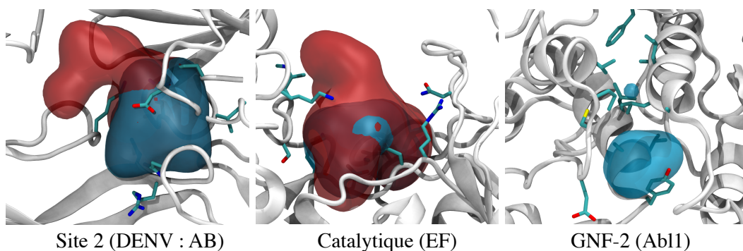
Figure IV.12 Comparaison visuelle entre la cavité moyenne des cavités de référence \bar{C}^{50\%} (en bleu) et la cavité moyenne des cavités instantanées assignées à la poche de référence pour chaque site \bar{A}^{50\%} (en rouge). L'ensemble des cavités considérées pour A ne prend en compte que la plus petite cavité instantanée lorsque plusieurs sont assignées à une même conformation. Les cavités moyennes sont tronquées à 50 % d'apparition.
