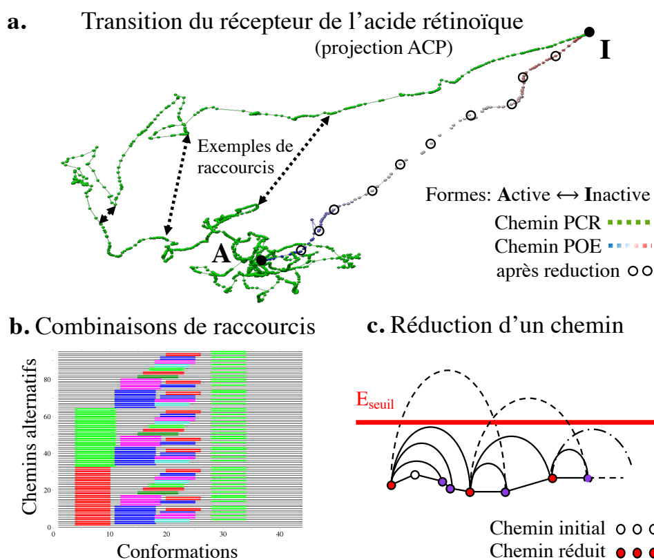
Figure III.2 Optimisation de chemins de transition à l'aide de POE. a. Projection sur les deux premiers modes d'une analyse en composante principale des chemins PCR et POE d'une transition du récepteur de l'acide rétinoïque. Le chemin PCR est topologiquement très complexe (points verts). POE recherche les raccourcis topologiques entre les structures intermédiaires du chemin PCR (flèches noires). Après plusieurs itérations, le chemin obtenu avec POE est beaucoup plus court (points en dégradé du bleu au rouge). Une procédure de réduction du chemin POE permet de supprimer les structures intermédiaires superflues à une échelle plus locale à différentes étapes de la méthode (ronds noirs, voir c. ). b. Combinatoire des combinaisons de raccourcis. Les lignes correspondent à des chemins de transition alternatifs qui seront confrontés au chemin initial grâce à des critères énergétiques (énergie maximale le long du chemin) et topologiques (nombre de points intermédiaires et longueur totale du chemin). Les lignes noires réfèrent à des portions du chemin initial. Les lignes en couleurs sont des raccourcis topologiques trouvés par POE. c. Procédure de réduction d'un chemin de transition à l'échelle plus locale. La réduction préserve la continuité énergétique du chemin. En d'autres termes, les structures calculées sur une interpolation entre chacune des paires consécutives de structures du chemin ne dépassent pas un plateau d'énergie E_{\text{plat.}} . Sous cette contrainte de continuité, la réduction supprime un maximum de structures intermédiaires.
