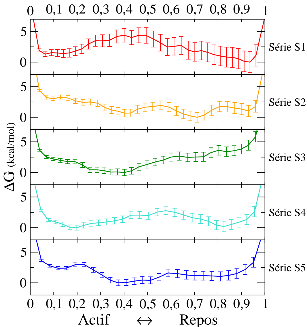
Figure III.8 Potentiel de force moyenne le long des chemins réactionnels. Dernières itérations de Swarms .
