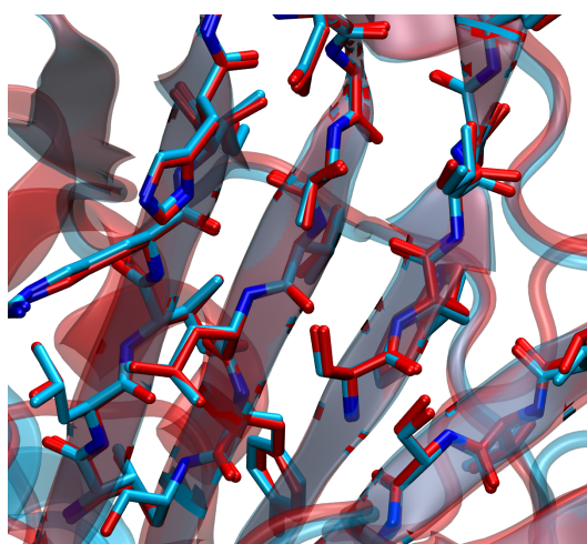
Figure II.1 Similarités structurales locales entre deux états du récepteur GluCl. Comparaison des structures cristallographiques du récepteur GluCl en état actif (bleu) et à l'état de repos (rouge). Vu prise dans la partie extracellulaire du récepteur (feuillets \beta du vestibule).
