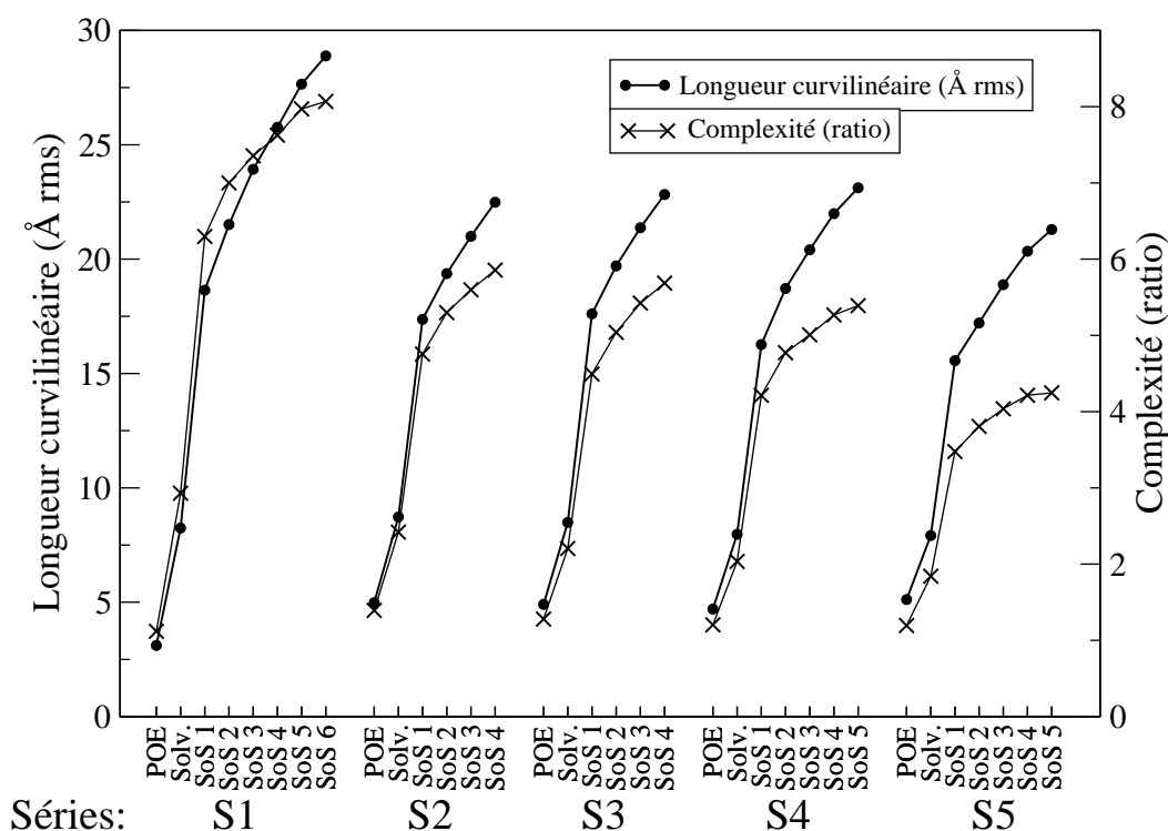
Figure III.7 Longueur curvilinéaire et complexité des chemins POE-SoS. La complexité des chemins après solvatisation et équilibration (Solv.) est donnée à titre indicatif. La complexité est calculée comme le ratio entre la longueur curvilinéaire et la longueur transverse du chemin : \left( \sum_{i=1}^{N-1} \text{RMSD}(X_i, X_{i+1}) / \text{RMSD}(X_1, X_N) \right) .
