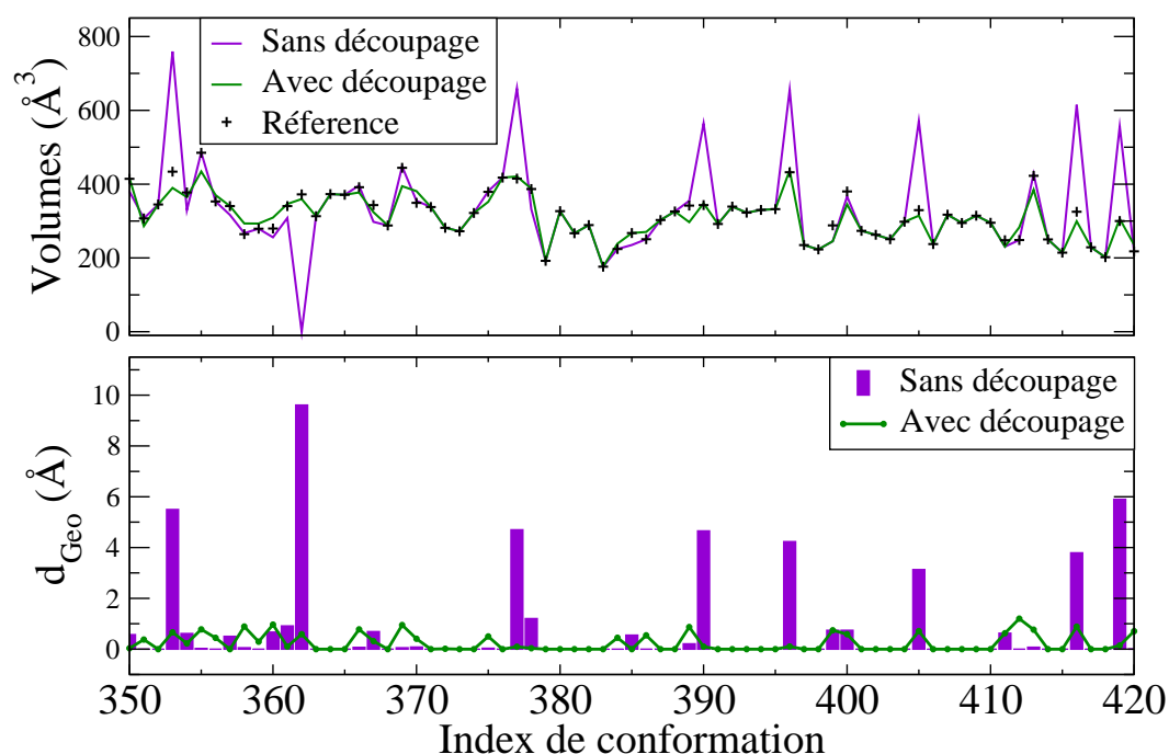
Figure IV.9 Accord entre les cavités de référence et les cavités prédites et effet du découpage des cavités. Comparaison du volume et de la géométrie des cavités de référence et prédites pour les sites \beta OG de la dengue, chaîne B. En haut : suivi du volume de la cavité de référence (+), de la cavité prédite (violet) et prédite après découpage des cavités instantanées (vert). En bas : distance géométrique d_{Geo} entre la cavité de référence et la cavité prédite, sans découpage (violet) et avec découpage (vert).
