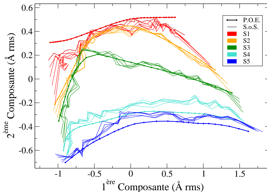
Figure III.6 Projection ACP des structures du récepteur nicotinique pour l'ensemble des 5 séries POE-SoS. Les chemins de transition individuels sont représentés par les courbes en pointillé (POE) et les traits fins (SoS). L'orientation de la première composante place les structures actives à gauche de la figure et les structures de repos à droite. Les deux composantes normalisées permettent d'avoir une estimation des distances entre les structures projetées (en angström).
