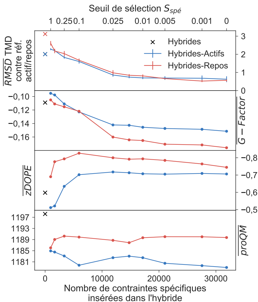
Figure II.8 Choix du seuil S_{spé} . Évolution des propriétés structurales de modèles \alpha 7 hybrides - actifs (courbes bleue) ou - repos (courbe rouge) en fonction du seuil S_{spé} de sélection des contraintes spécifiques (axe des abscisses du haut) et nombre de contraintes remplacées dans les contraintes hybrides correspondant (axe des abscisses du bas). Chaque propriété est moyennée à partir de 1 000 modèles créés en utilisant le seuil S_{spé} . RMSD est le RMSD moyen entre les domaines transmembranaires (sélection des C_{\alpha} et index de résidus supérieur à 204) des modèles Hybride-Repos (respectivement Hybrides-Actif) contre le meilleur modèle Classique-Repos (Classique-Actif) et après alignement des structures. Les scores G-Factor, proQM et zDOPE sont orientés par ordre croissant de qualité des structures (meilleures qualités en haut).
