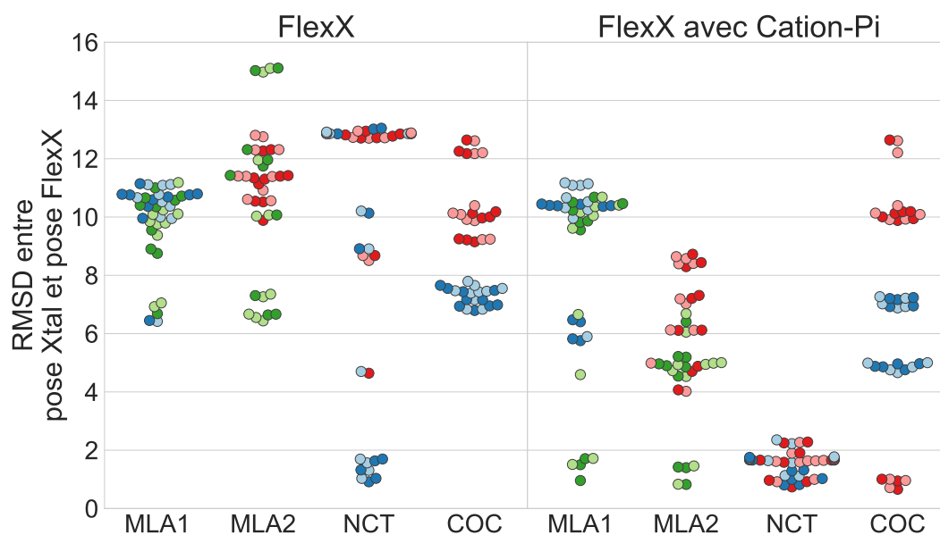
Figure V.3 Distance RMSD à la pose cristallographique pour chacune des 160 poses générées par les dockings . À gauche avec la version originale de FlexX, et à droite après incorporation de l'interaction cation- \pi (avec contribution énergétique à 0,75 kcal/mol). La couleur des points met en valeur les 10 poses d'un même docking , soit 4 couleurs différentes (2 interfaces x 2 énantiomères) pour chaque molécule.
