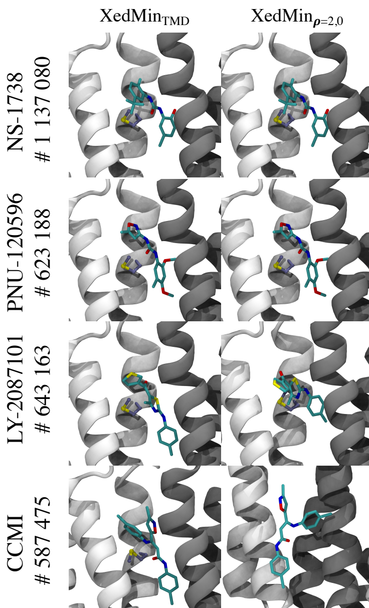
Figure V.10 Poses de meilleures affinités par les scores XedMin TMD et XedMin \rho=2,0 pour chacun des modulateurs allostériques amarrés sur l'ensemble du récepteur \alpha 7 . Meilleures poses XedMin TMD : pose de meilleur score XedMin sur l'ensemble des poses situées dans la partie transmembranaire du récepteur. Meilleures poses XedMin \rho=2,0 : pose de meilleur score XedMin sur l'ensemble des poses placées sur le récepteur et après repondération à \rho = 2,0 des termes d'interaction. Le nombre total de poses considérées est indiqué sous le nom de chaque molécule. Lorsque la pose se situe dans le site 1, la méthionine 253 est représentée en licorice violet.
