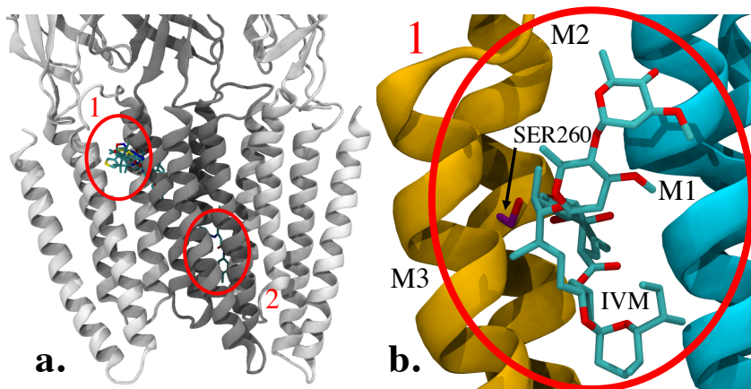
Figure V.9 Localisation des poses de meilleures affinités. a. Localisation des 8 meilleures poses obtenues par le protocole de docking global. La région 1 , la plus représentée, se trouve à l'interface des sous-unités, entre les hélices M3(+), M2(+) et M1(-), et est similaire aux sites de liaison de l'ivermectine des récepteurs GluCl et Glycine. Le site 2 se trouve dans la partie basse du pore, entre les hélices M2. 3 chaînes du récepteur \alpha 7 sont représentées, avec la seconde sous-unité en gris foncé. b. Vue du site de liaison de l'ivermectine, structure PDB : 3RIF avec sous-unités portant la boucle C (+) en orange, et la sous-unité complémentaire (-) en bleu. La serine 260 est visible en licorice violet.
