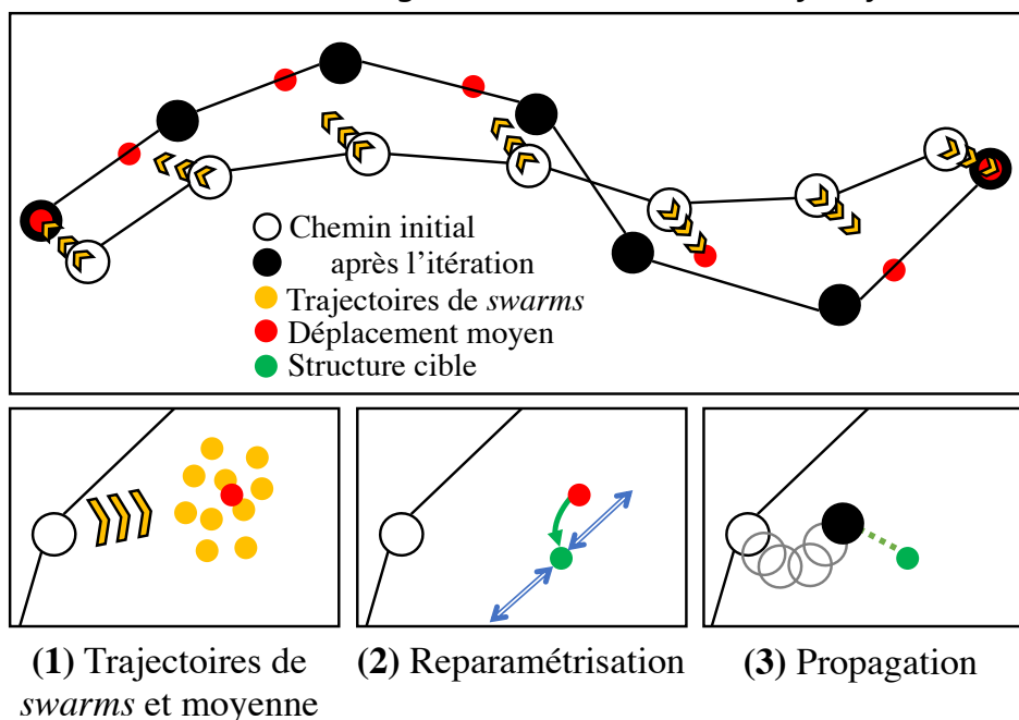
Figure III.1 Principe de la String method with swarms of trajectories . À partir d'une série de structures intermédiaires séparant deux états distincts de la protéine, le chemin est relaxé dans le paysage d'énergie libre par la procédure suivante réalisée sur chacune des structures du chemin : (1) Une multitude de courtes trajectoires de dynamique moléculaire indépendantes et sans contraintes sont lancées à partir de la structure initiale (bille blanche). Les conformations de fin de trajectoires (billes jaunes) sont converties en une structure moyenne (bille rouge), qui pointe la direction du gradient de diffusion. (2) la structure moyenne est reparamétrisée pour limiter une dérive des structures le long du chemin. La structure cible (bille verte) est ainsi créée pour préserver une équidistance entre les structures. (3) une trajectoire de propagation est lancée à partir de la structure initiale et une contrainte harmonique sur la bille cible. La dernière structure de la trajectoire de propagation (bille noire) devient un nouveau point intermédiaire du chemin de transition. Après plusieurs itérations de ce protocole, les chemins produits convergent dans une vallée du paysage d'énergie libre.
