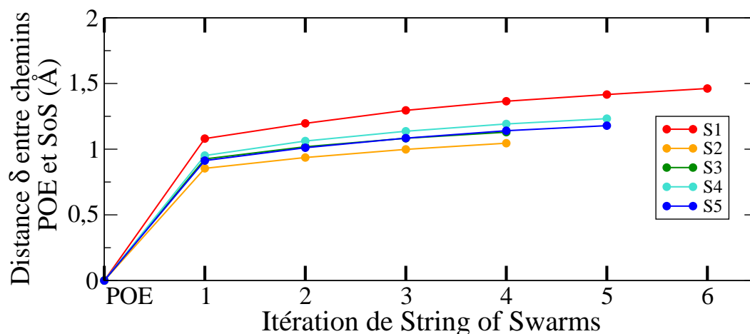
Figure III.13 Convergence géométrique des itérations de String of Swarms . Distance \delta (voir Matériels et Méthodes) entre le chemin POE et chacune des itérations de String of Swarms pour chaque série POE-SoS. Note : la trace du chemin S3 est très proche, mais distincte, de celle du chemin S5.
