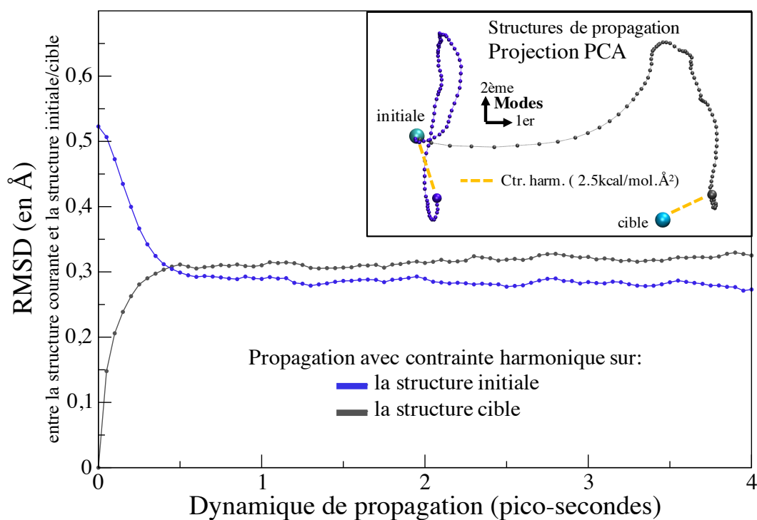
Figure VII.4 Accessibilité de la structure cible lors des trajectoires de propagation. Suivi de la distance (RMSD) à la bille cible lors de la trajectoire de propagation, avec contrainte harmonique sur la cible et sur l'hyperplan bissecteur. Pour comparaison, la bille cible est ensuite remplacée par la bille initiale lors d'une seconde propagation. La projection de l'ensemble des structures sauvegardées sur les deux premiers modes d'une ACP (sur les mêmes structures) permet de visualiser l'évolution des propagations vers leurs cibles respectives. Dès la première picoseconde de simulation, la structure converge très proche de sa cible ( \approx 0,3 \text{ \AA} ) et ne peut s'en rapprocher plus près malgré les 3 ps de simulation suivant. Cette distance minimale de 0,3 \text{ \AA} est incompressible du fait des mouvements aléatoires qui agitent la dynamique moléculaire thermalisée.
