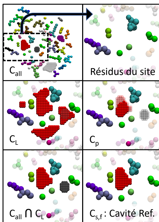
Figure IV.3 Détermination des trajectoires de cavités de référence. Calcule des cavités de référence C_{s,f} pour une conformation f du site de référence s . C_{all} montre les cavités instantanées du système entier. Les cavités sont ensuite calculées avec mkgridXf en ne tenant compte que des résidus du site de référence. C_L correspond à ce résultat, mais doit être corrigé de 2 façons : (1) C_{all} \cap C_L permet de supprimer les points de C_L qui ne sont pas dans C_{all} et qui ne seront donc jamais observés dans une détection de cavités sur la protéine entière. (2) La suppression des cavités périphériques ou trop petites, en ne maintenant que les cavités dont au moins un point de grille est dans C_p .
