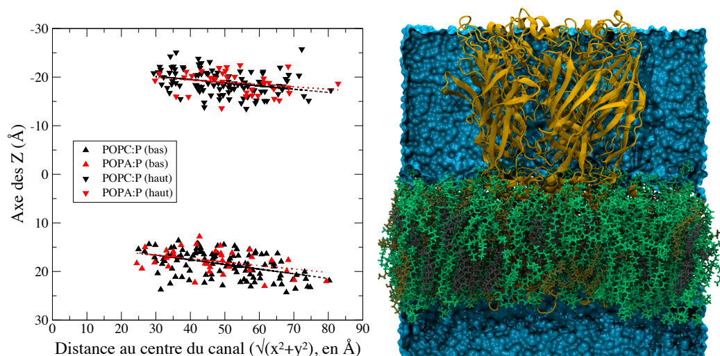
Figure VII.6 Mesure de la stabilité des lipides de la membrane. La hauteur (axe des z) des atomes de phosphore des têtes de lipides en fonction de leur distance au centre du canal ionique ((x,y)=(0,0)) . Cette mesure permet de surveiller que la bicouche lipidique ne se décompose pas au cours des simulations.
