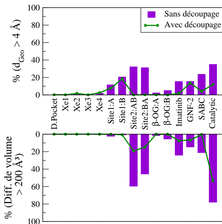
Figure IV.11 Pourcentage de conformations où les cavités présentent de larges déviations par rapport à la cavité de référence. Des exemples de grande dissimilarité géométriques ( d_{Geo} > 4 \text{ \AA} , en haut) et de larges différences de volumes ( > 200 \text{ \AA}^3 , en bas) sont rapportés. Les valeurs pour les cavités prédites sans découpage des cavités sont illustrées en violet, et en vert pour les cavités découpées.
