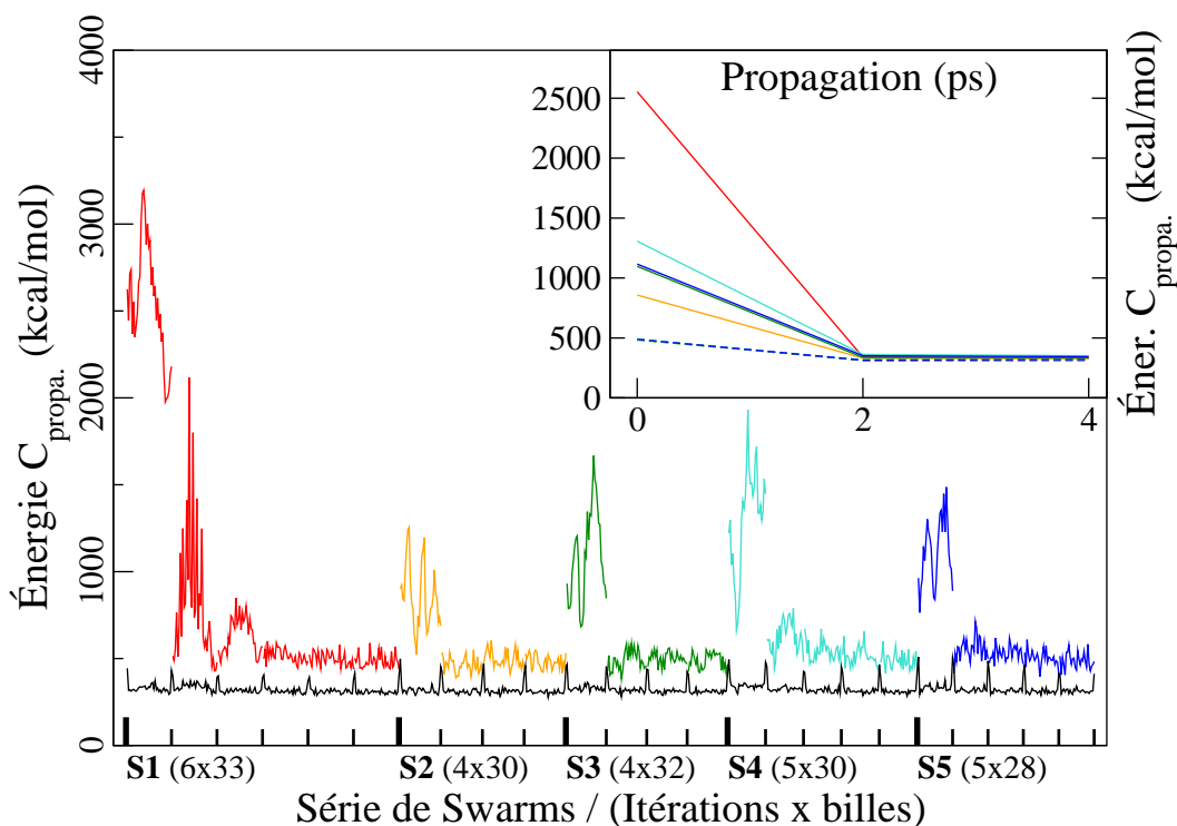
Figure III.12 Évolution de la contrainte de propagation. Le graphe global spécifie pour chacune des billes des chemins SoS, l'énergie de la contrainte à t=0 ps (en couleur) et t=4 ps (en noir). L'encart en haut à droite renseigne la moyenne des énergies sur toutes les billes d'une itération SoS à t=0 ps, t=2 ps et t=4 ps, pour la première (traits pleins) et la dernière (traits pointillés) itération de chaque série de Swarms (différentes couleurs).
