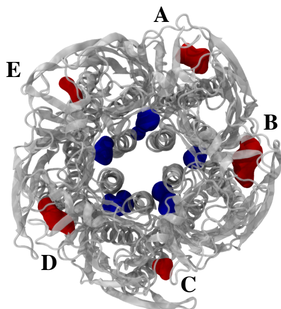
Figure IV.14 Suivi des cavités avec prise en compte de la symétrie de séquence. Bien que spatialement situées à des positions différentes du récepteur, ces cavités instantanées (rouge ou bleu) sont placées dans des sites similaires.
