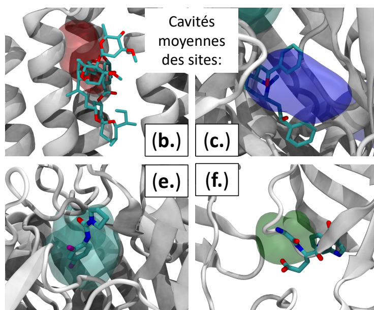
Figure V.8 Alignement de co-cristaux de récepteurs homologues sur la première conformation de la transition. En haut à gauche, cavité moyenne du site b. et structure du récepteur GluCl (PDB : 3RIF) liée avec l'ivermectine (IVM). En haut à droite, cavité moyenne du site orthostérique ( c. ) et structure de la chimère \alpha 7 AChBP (PDB : 5AFH) liée avec la lobéline (LOB). En bas à gauche, cavité moyenne du site e. et structure de la chimère \alpha 7 AChBP (PDB : 5AFK) liée au modulateur allostérique 5VU. En bas à droite, cavité moyenne du site f. et le triplet de résidus conservés GEW définissant le site de régulation par le \text{Ca}^{2+} [295, 296].
