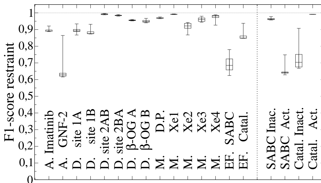
Figure IV.8 Distribution des 100 meilleurs scores F1_{site} . Les systèmes étudiés sont abrégés par A., D., M. et EF. pour abl1, protéine E de la dengue, myoglobine, et EF respectivement. Les diagrammes en boîte retranscrivent : minimum, 1 er quartile, médiane, 3 e quartile et valeur maximale. Sur la droite, F1_{site} est calculé soit sur les 1 000 premières conformations “inactives”, ou sur les conformations 1 001 à 2 000 “actives” de la trajectoire EF pour les sites catalytiques et SABC.
