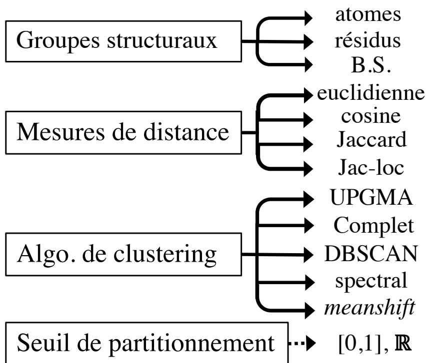
Figure IV.7 Combinatoire des combinaisons d’options pour le suivi des cavités. B.S. : Backbone-Sidechain, UPGMA ou Complet : Partitionnement hiérarchique avec lien moyen ou maximum
