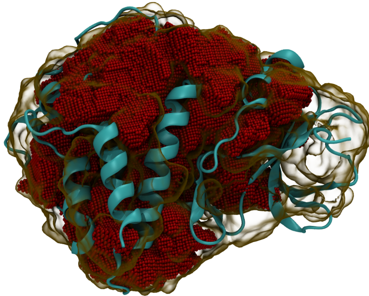
Figure IV.5 Domaine de définition des cavités de la plus large composante connexe du graphe séquentiel. Pour la trajectoire abl1 (points rouges) le volume couvert représente 67,1 % du domaine de définition de l'ensemble des cavités qui apparaissent au cours de la trajectoire (surface transparente).
