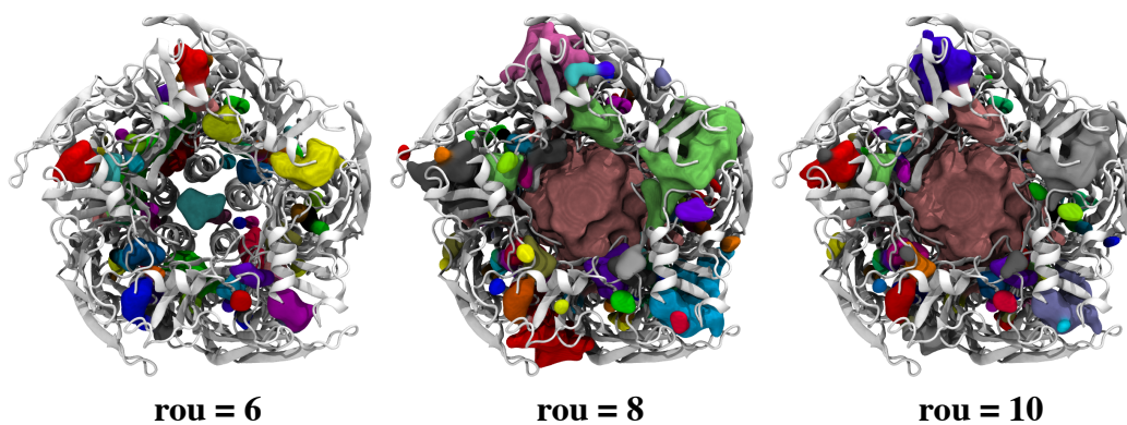
Figure IV.13 Effet du paramètre rou lors de la détection des cavités. Les cavités détectées dans cette conformation (canal en état fermé) ont été calculées avec une valeur du rou égale à 6, 8 et 10 Å. La variation du rayon de la grande sphère de détection de cavités ronge plus ou moins la cavité centrale et segmente les cavités à la surface du pore.
