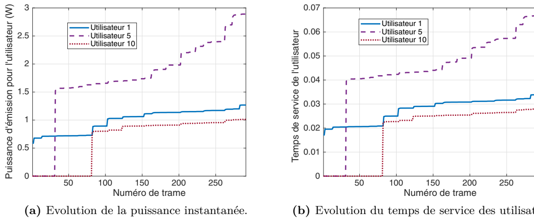
Figure 3.8 – Evolution des temps de service et des puissances instatannées lorsque de nouveaux utilisateurs se connectent au réseau.
