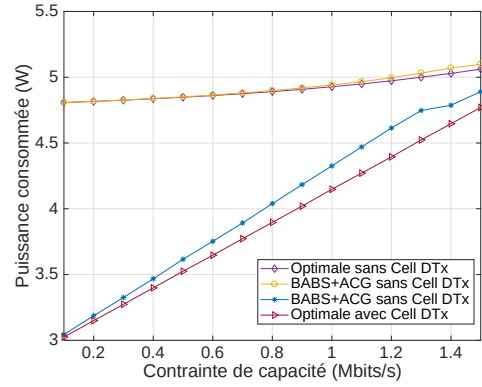
(d) Femto-cellule, \rho_1^M = 5 dB, \rho_2^M = 25 dB
