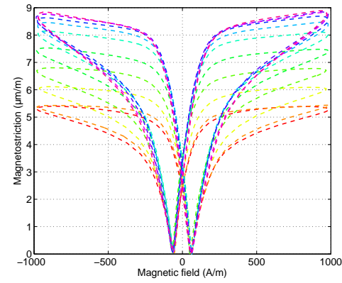
(d) Magnetostrictive deformation at point B: \varepsilon_B^{\parallel}(H)
