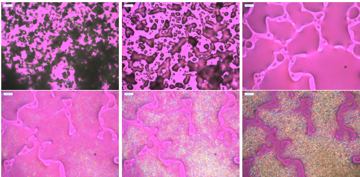
FIGURE 2.43 – Cristallisation de la poudre de PEKK pour un refroidissement à 20 °/min
