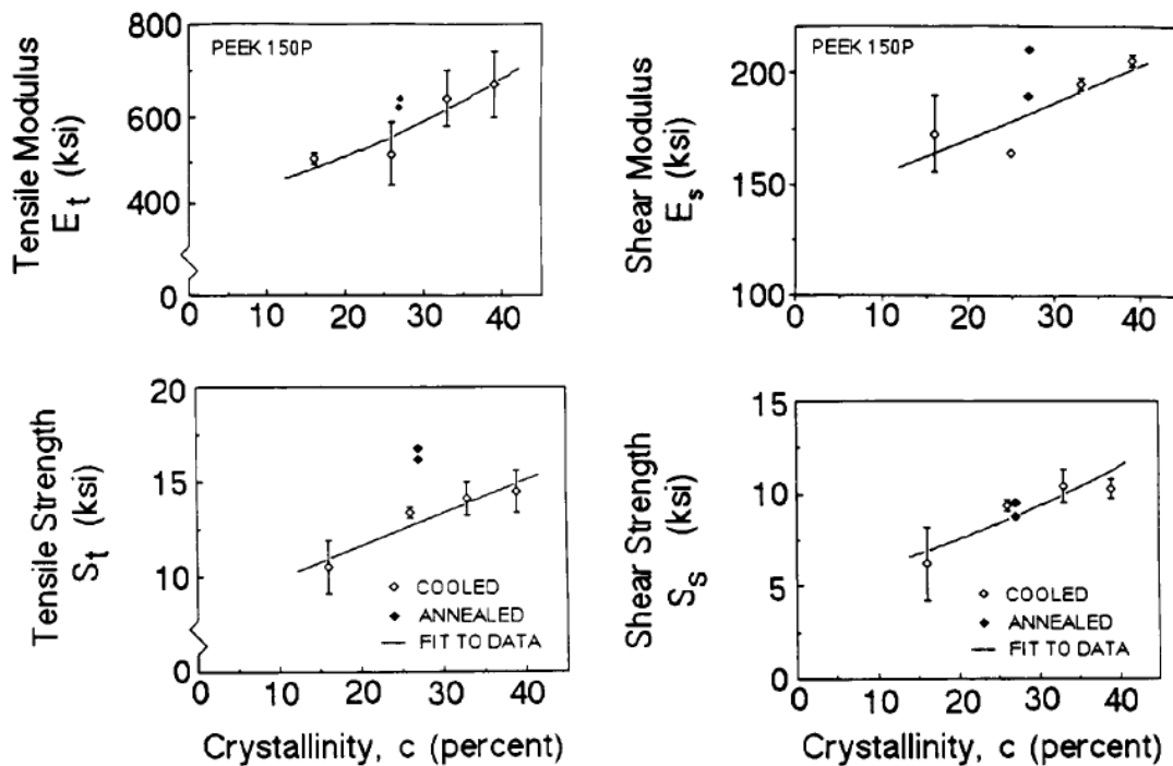
(a) Propriétés en traction du PEEK 150P en fonction du taux de cristallinité
