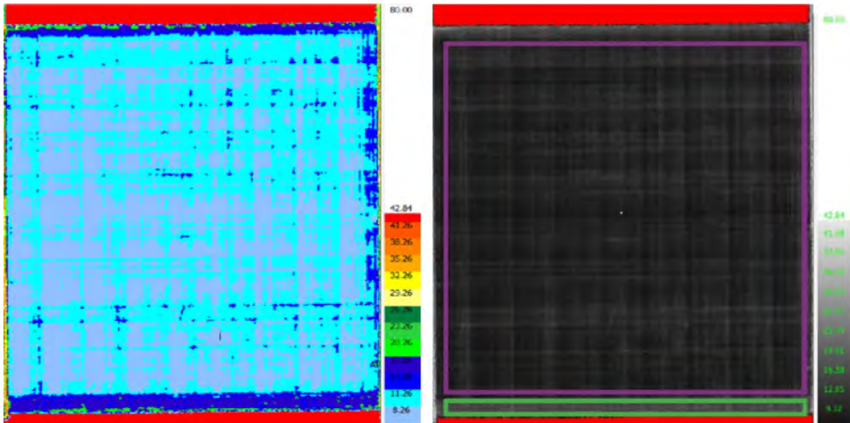
FIGURE 4.5 – Cartographie C-Scan d'une plaque de composite non-chargeé
