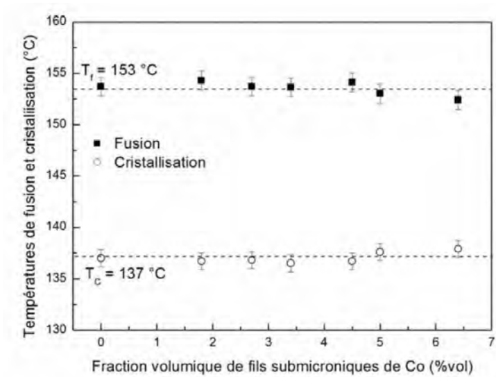
FIGURE 1.24 – Évolution des températures de fusion et de cristallisation avec la fraction volumique de fils submicroniques de cobalt [Nguyen, 2014]
