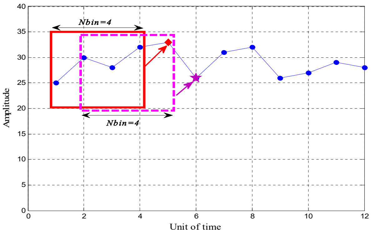
Figure III. 4 : Procédure de traitement numérique en ligne des ANN proposés.
