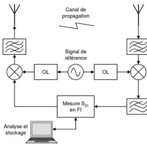
Figure 1-33: Passage du domaine fréquentiel au domaine temporel [136]
