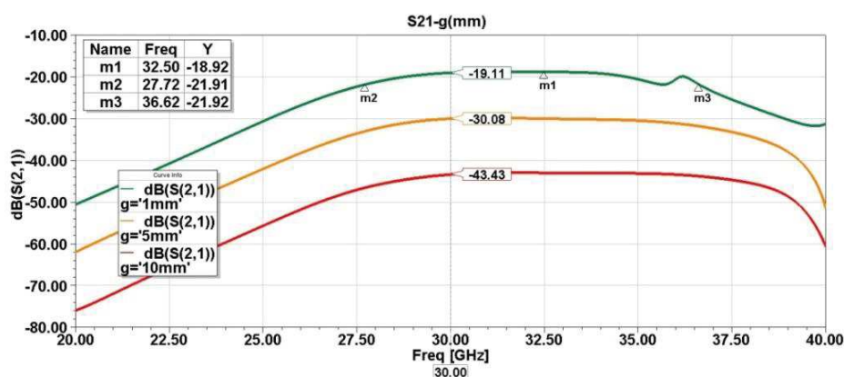
Figure 2-14: Évolution du paramètre S_{21} entre deux dipôles sur Si/Air en bande K_a en fonction de g
