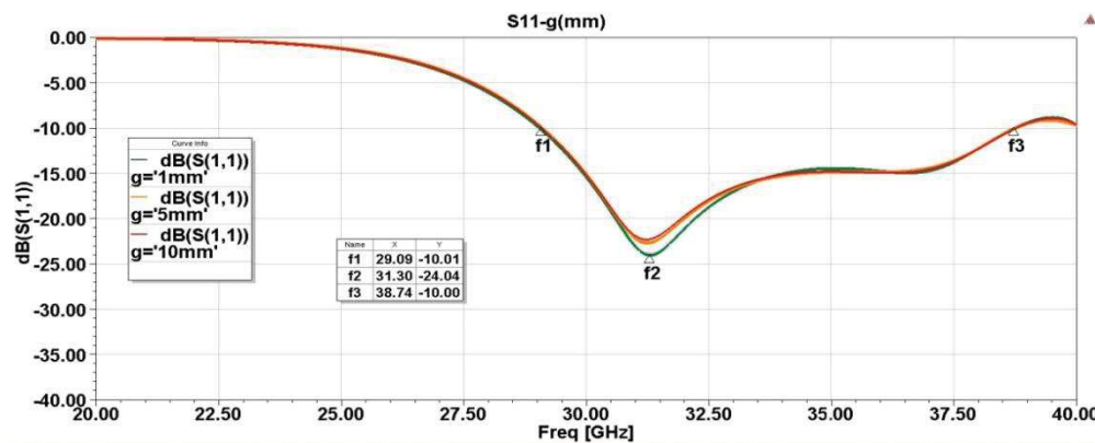
Figure 2-13: Évolution du paramètre S_{11} pour les dipôles sur Si/Air en bande K_a en fonction de g
