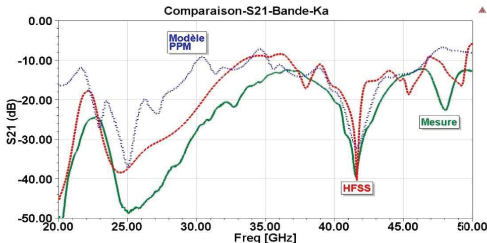
Figure 2-45: Comparaison entre simulation, mesure et modèle PPM de paramètre S_{21} pour un canal en bande K_a
