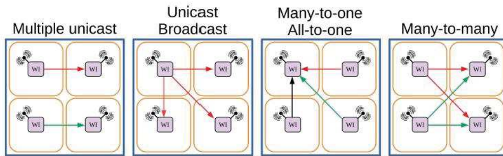
Figure 4-11: Modèles de communication sans fil pour une topologie hybride WiNoC en cluster avec N = 4 clusters [41]
