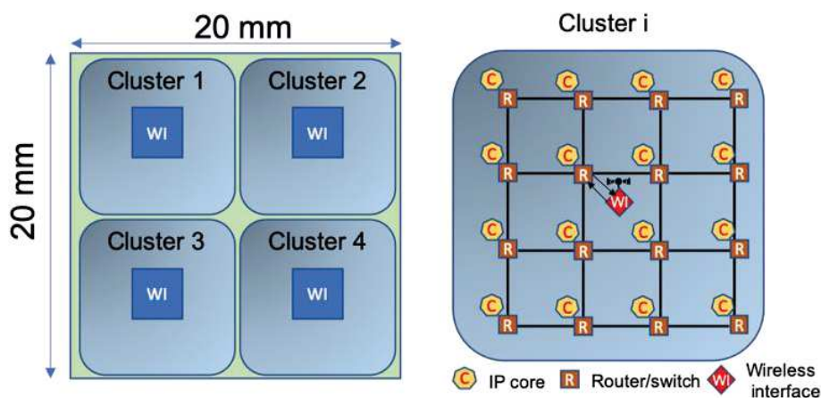
Figure 2: illustration d'un scénario de communication retenu pour le projet BBC
