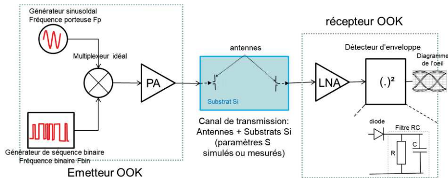
Figure 4-2: schéma fonctionnel d'une chaîne de transmission WiNoC
