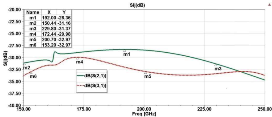
Figure 3-53: Paramètres de transmission entre les monopoles avec un plan métallique supérieur
