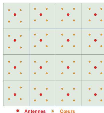
Figure 1-45: Une topologie maillée avec 16 antennes et 64 cœurs
