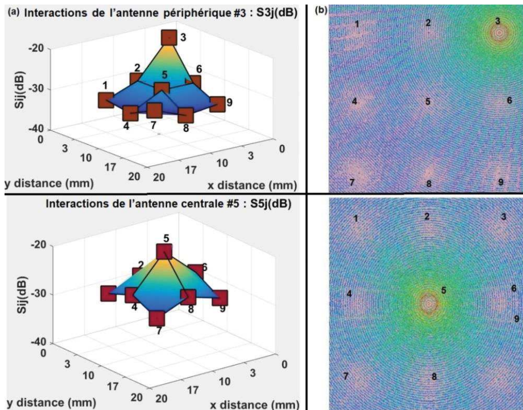
Figure 3-55: (a) Interactions de l'antenne centrale # 5 et de l'antenne périphérique #3 ; (b) leurs distributions de champs électriques respectives
