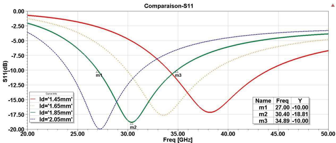
Figure 2-4: Évolution du paramètre S_{11} pour un dipôle sur un substrat infini en bande K_a en fonction de L_d
