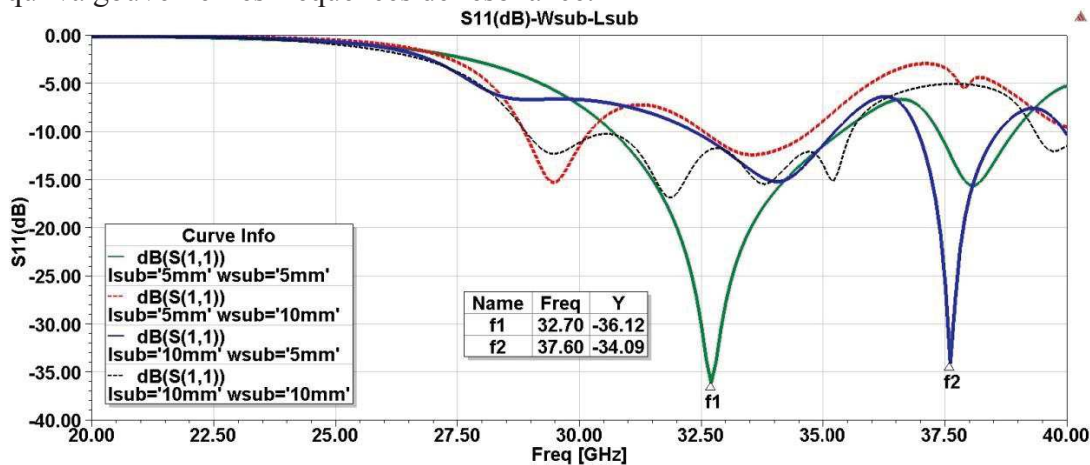
Figure 2-8: Évolution du paramètre S_{11} pour un dipôle sur Si en bande K_a en fonction de W_{sub} et L_{sub}
