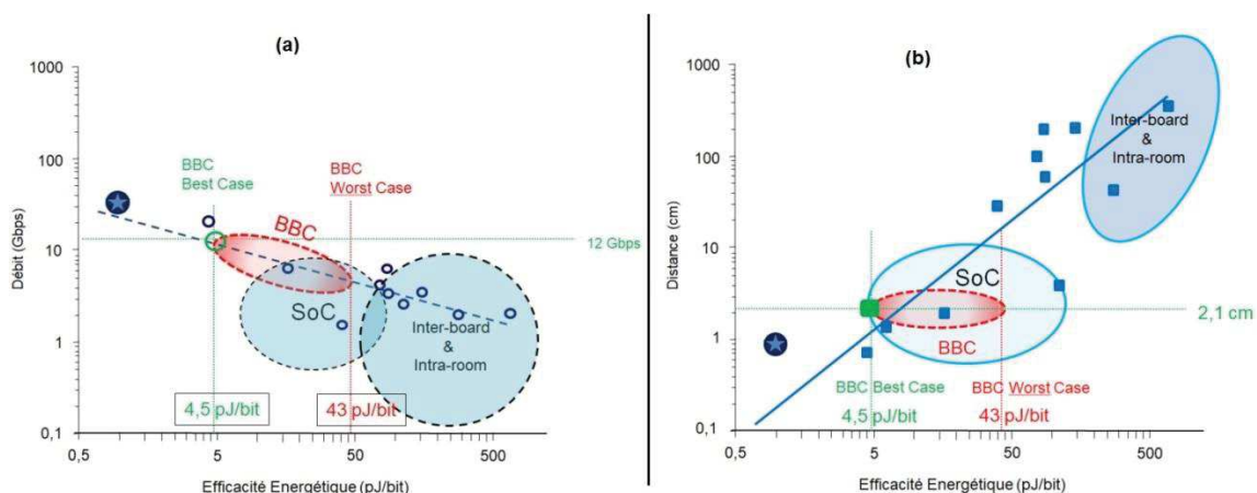
Figure 4-17: Positionnement du projet BBC par rapport à l'état de l'art de WiNoC [180]
