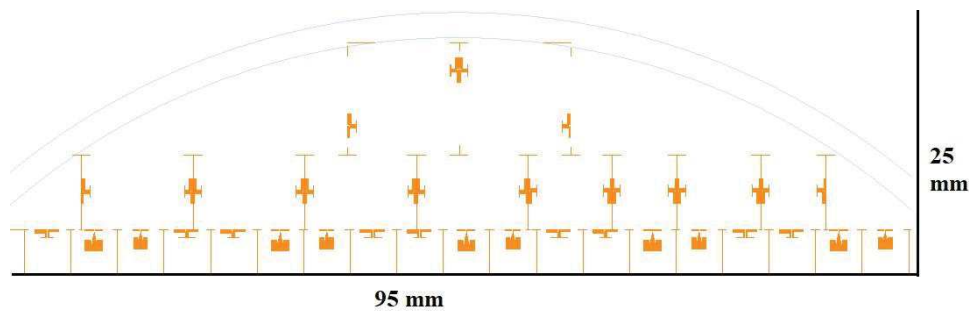
Figure 2-27: Une partie du masque du wafer réalisé
