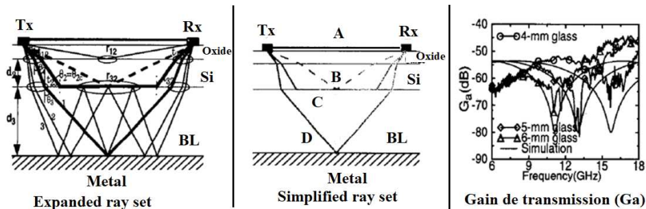
Figure 1-40: Modèles de rayons et gain de transmission correspondant [137]
