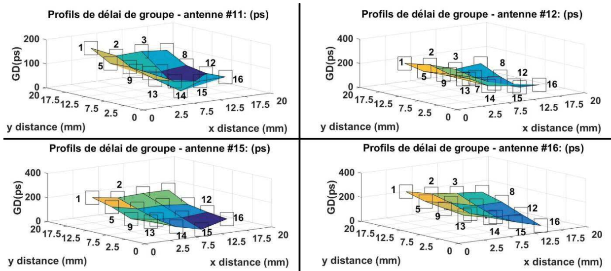
Figure 3-60 : Profils des délais de groupe des antennes #11, #12, #15 et #16
