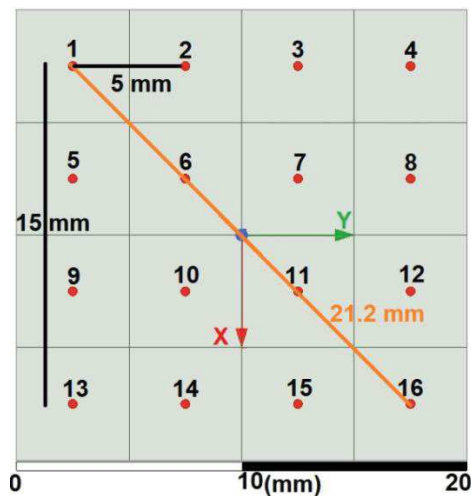
Figure 4-10: Scénario de 16 monopoles
