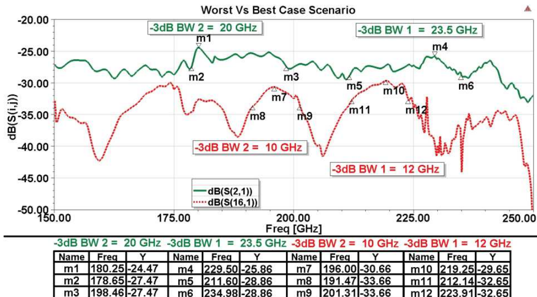
Figure 3-58: Comparaison des Best-Case scenario et Worst-Case scenario des 16 antennes
