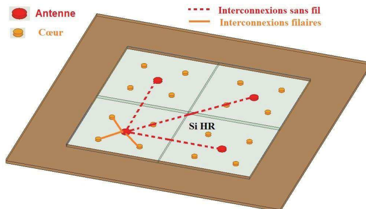
Figure 1-14: Solution hybride avec des interconnexions filaires et sans fils
