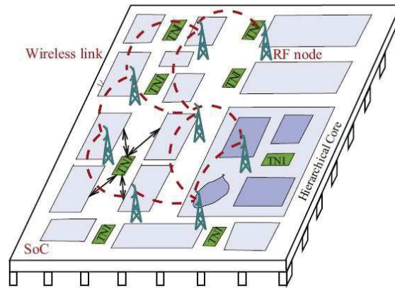
Figure 1-13: Exemple de WiNoC utilisé pour un MPSoC [39]
