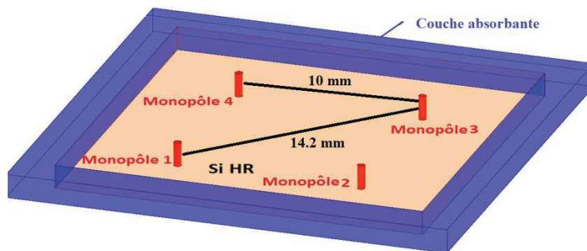
Figure 3-49: Scénario avec 4 monopoles
