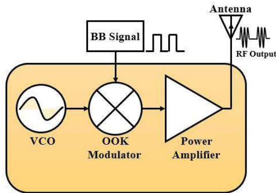
Figure 1-21: Architecture de l'émetteur dans [81]
