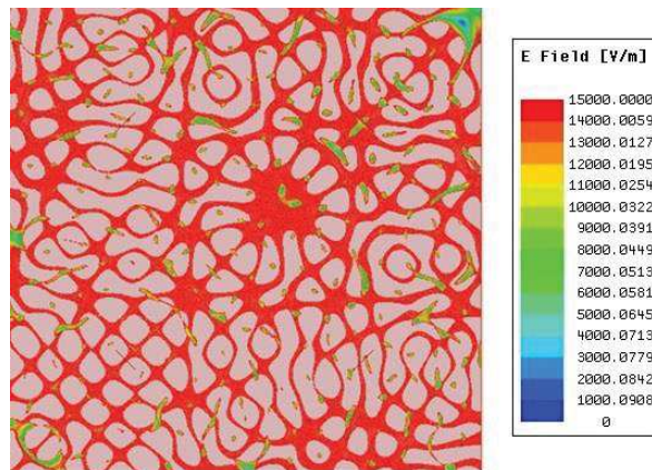
Figure 2-19: Distribution du champ électrique dans la cavité surdimensionnée
