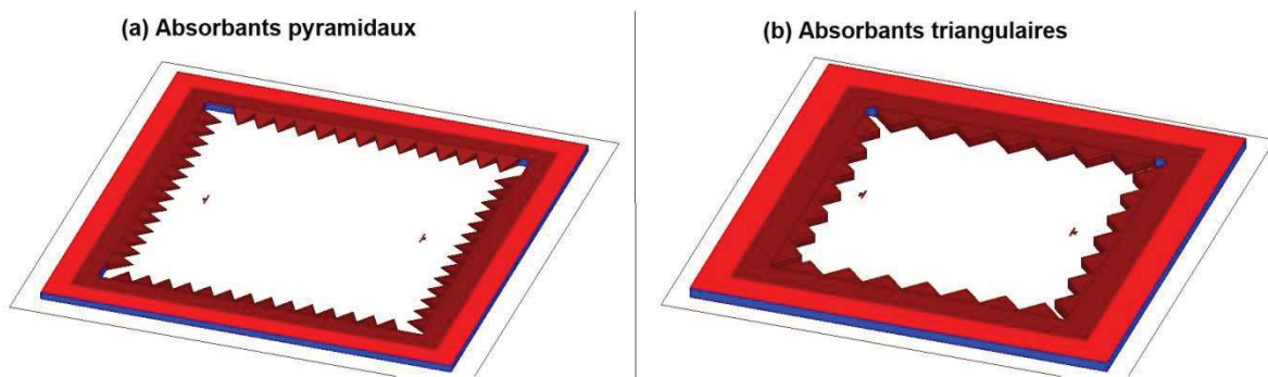
Figure 3-28: Absorbants pyramidaux et triangulaires dans le substrat
