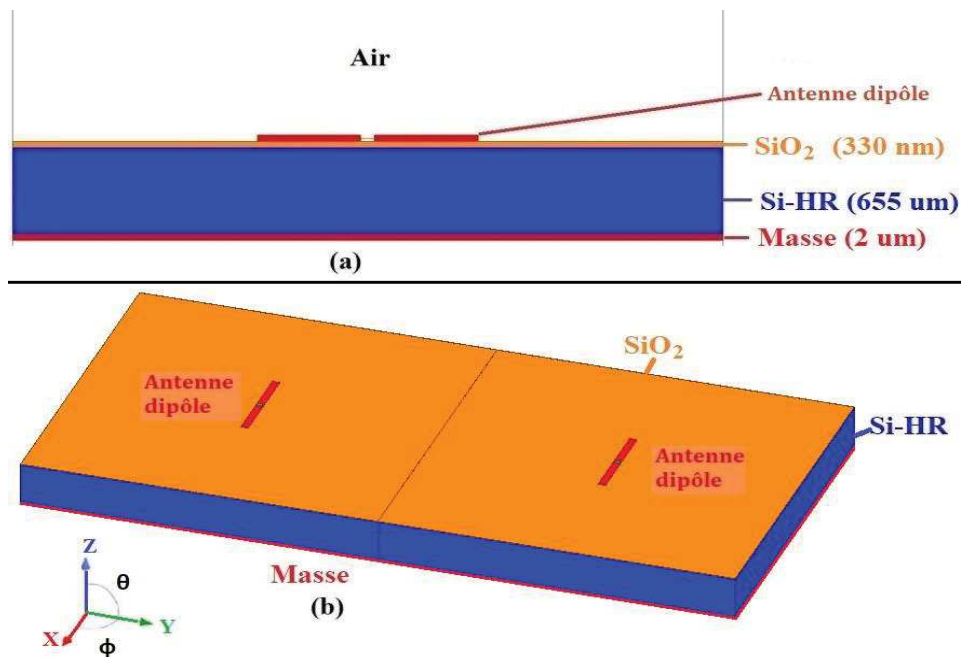
Figure 2-2: Scénario de base d'un canal: (a) vue de profil; (b) vue 3D
