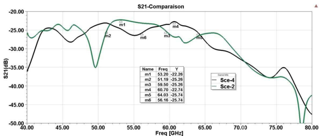
Figure 3-34: Comparaison des paramètres S_{21} des scénarios (2) et (4) dans la bande V
