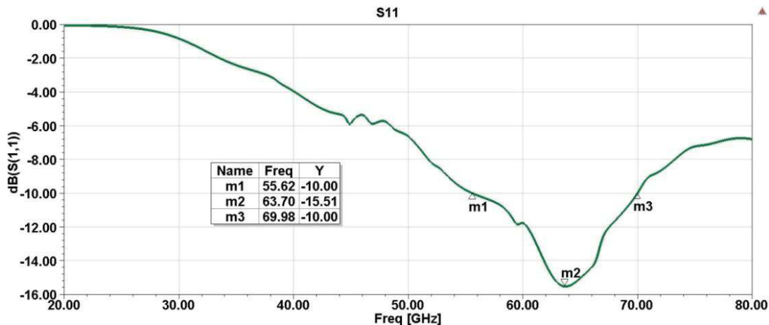
Figure 3-31: Paramètre S_{11} du scénario (2) dans la bande V
