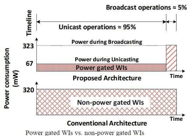
Figure 4-20: Consommation avec ou sans 'Power gating' [58]
