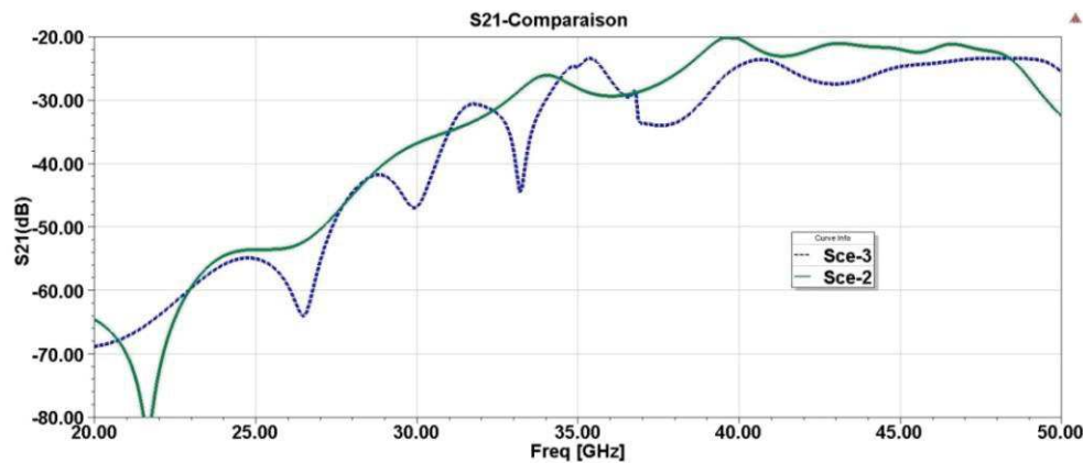
Figure 3-25: Comparaison des paramètres S_{21} des scénarios (2) et (3) dans la bande Q
