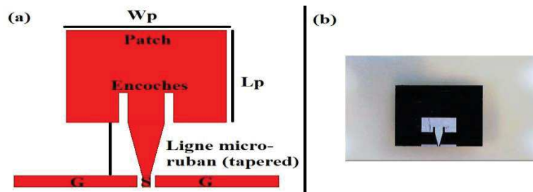
Figure 2-26: (a) Conception des antennes patch et (b) patch réalisé
