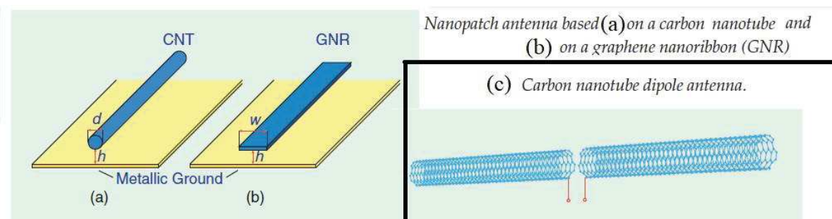
Figure 1-25: Antennes à base de CNT ou du Graphène [104]
