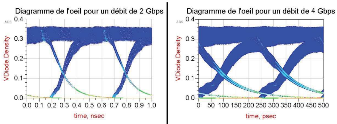
Figure 4-8: Diagrammes de l'œil dans le cas des débits binaires de 2 et 4 Gbps avec un gain de 10 dB
