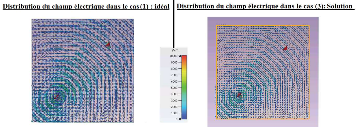
Figure 3-9: Distribution du champ électrique dans le cas (1) et (3)
