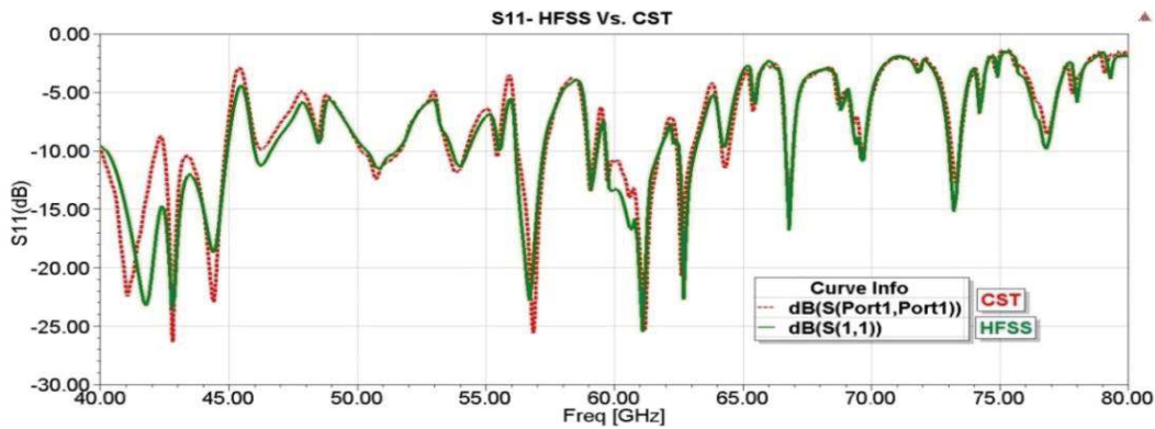
Figure 2-15: Paramètre S_{11} d'un dipôle sur Si en bande V simulé sur CST et HFSS
