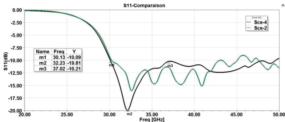
Figure 3-30: Comparaison des paramètres S_{11} des scénarios (2) et (4) dans la bande Q
