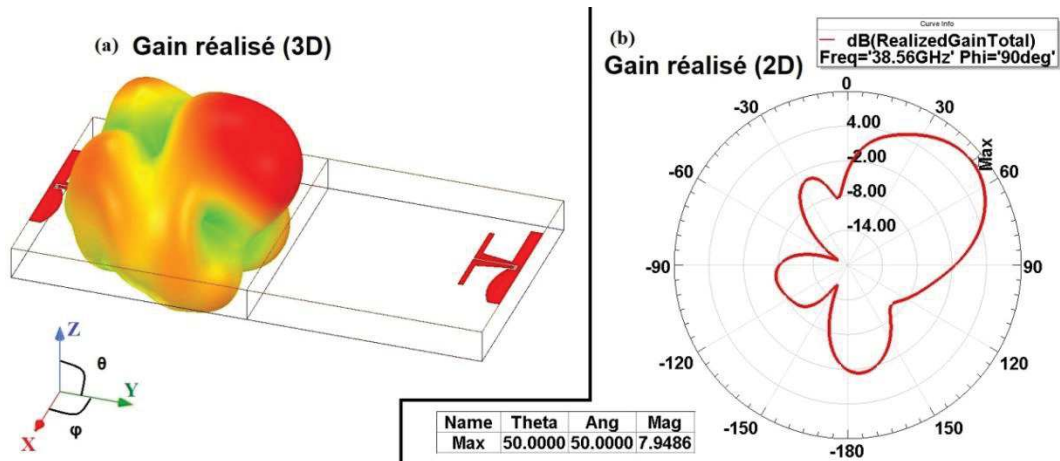
Figure 2-32: Diagramme de rayonnement d'un dipôle: (a) Vue 3D; (b) à \varphi = 90^\circ
