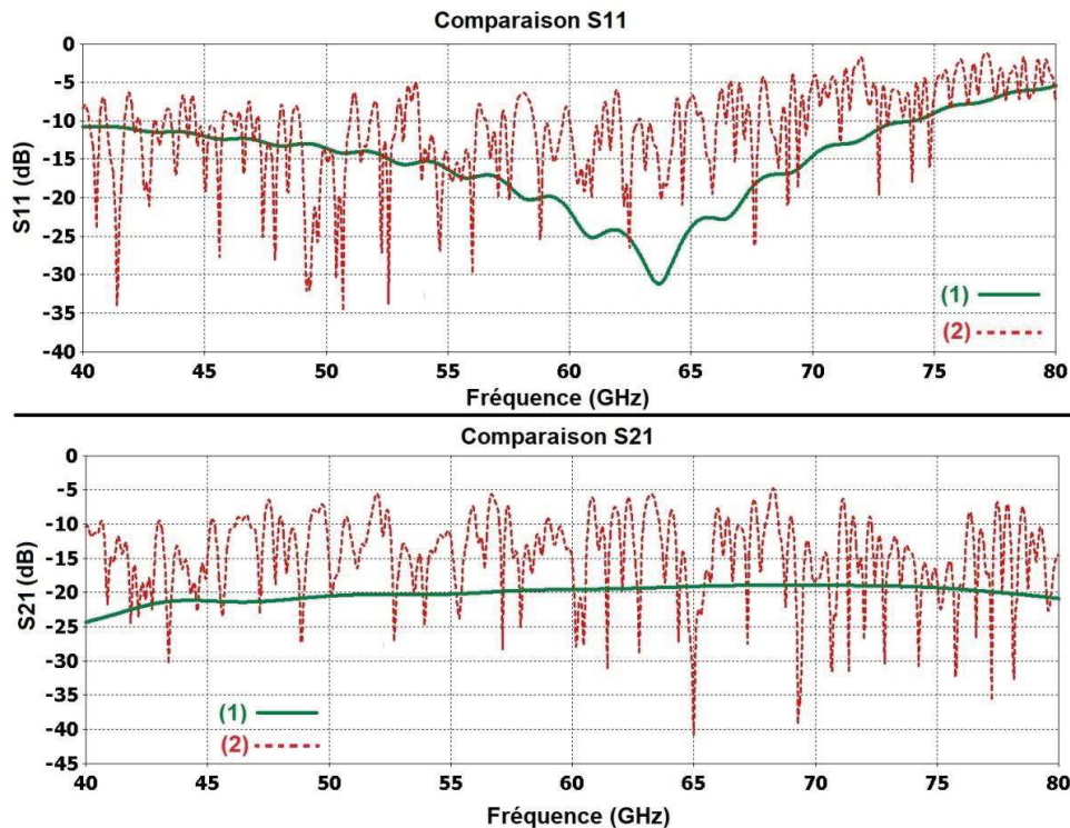
Figure 3-3: Comparaison des paramètres S des cas (1) et (2)
