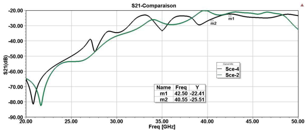
Figure 3-29: Comparaison des paramètres S_{21} des scénarios (2) et (4) dans la bande Q
