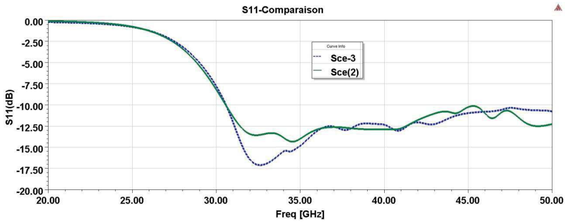
Figure 3-24: Comparaison des paramètres S_{11} des scénarios (2) et (3) dans la bande Q
