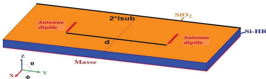
Figure 2-10: Canal de propagation entre deux dipôles en bande Ka
