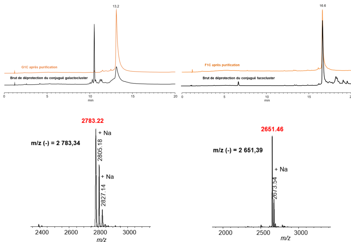
Figure 102 : Chromatogramme HPLC-C18 (gradient : 1 % \text{CH}_3\text{CN} 50 mM TEAAc - 24 % \text{CH}_3\text{CN} 50 mM TEAAc -20 min) à 260 nm et spectre MALDI-TOF du galactocluster mono-catéchol G1C (gauche) et du fucocluster mono-catéchol F1C (droite)
