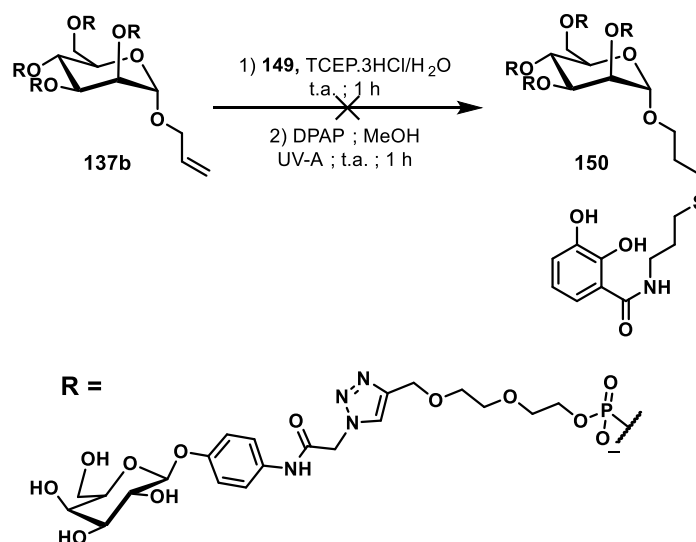
Schéma 39 : Synthèse du conjugué galactocluster mono-catéchol
