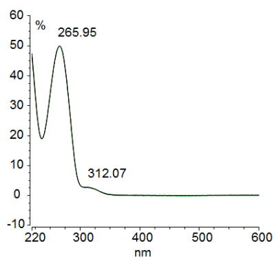
Figure 51 : Spectre UV du composé à 13,3 min
