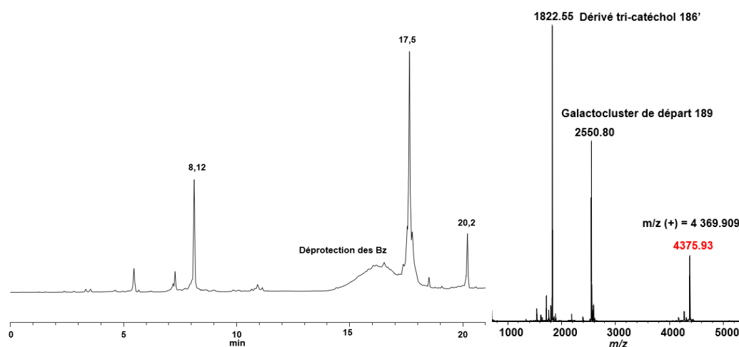
Figure 103 : Chromatogramme HPLC-C18 (gradient : 1 % CH 3 CN 50 mM TEAAc - 24 % CH 3 CN 50 mM TEAAc -12 min- 24 % CH 3 CN 50 mM TEAAc - 80 % CH 3 CN 50 mM TEAAc -7 min et spectre MALDI-TOF en mode positif du brut 190
