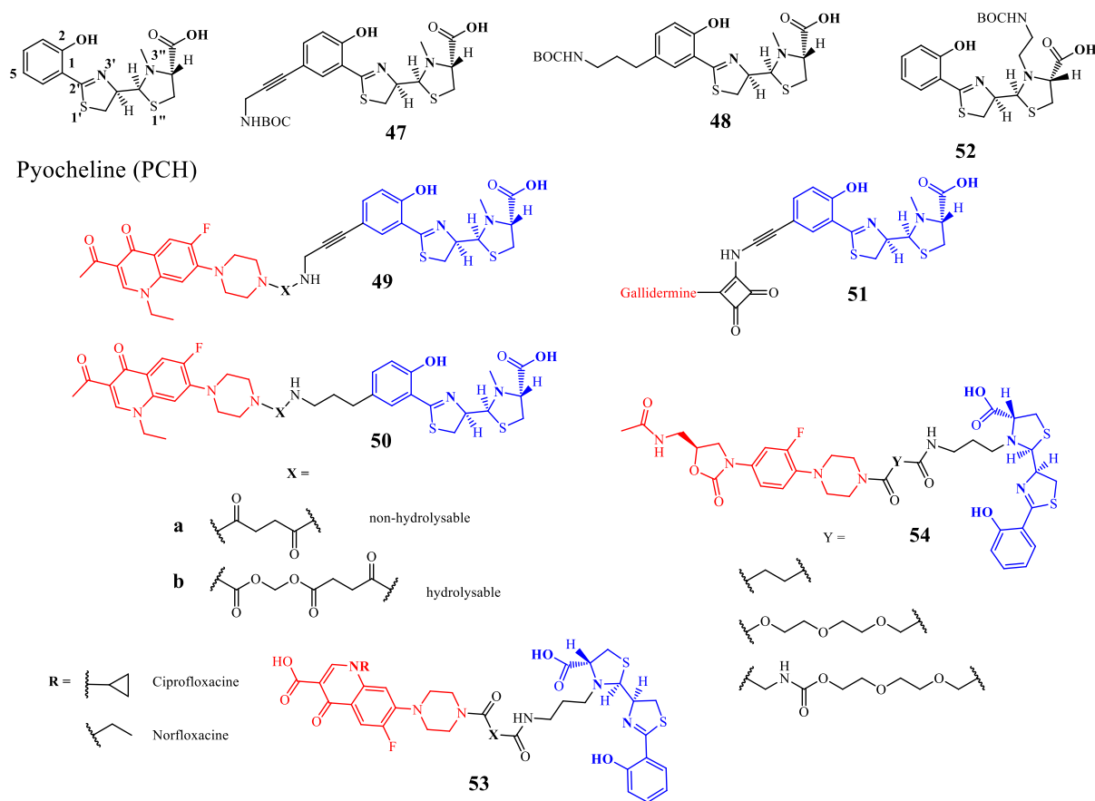
Figure 37 : Structure des conjugués antibiotique-PCH apparu dans la littérature
