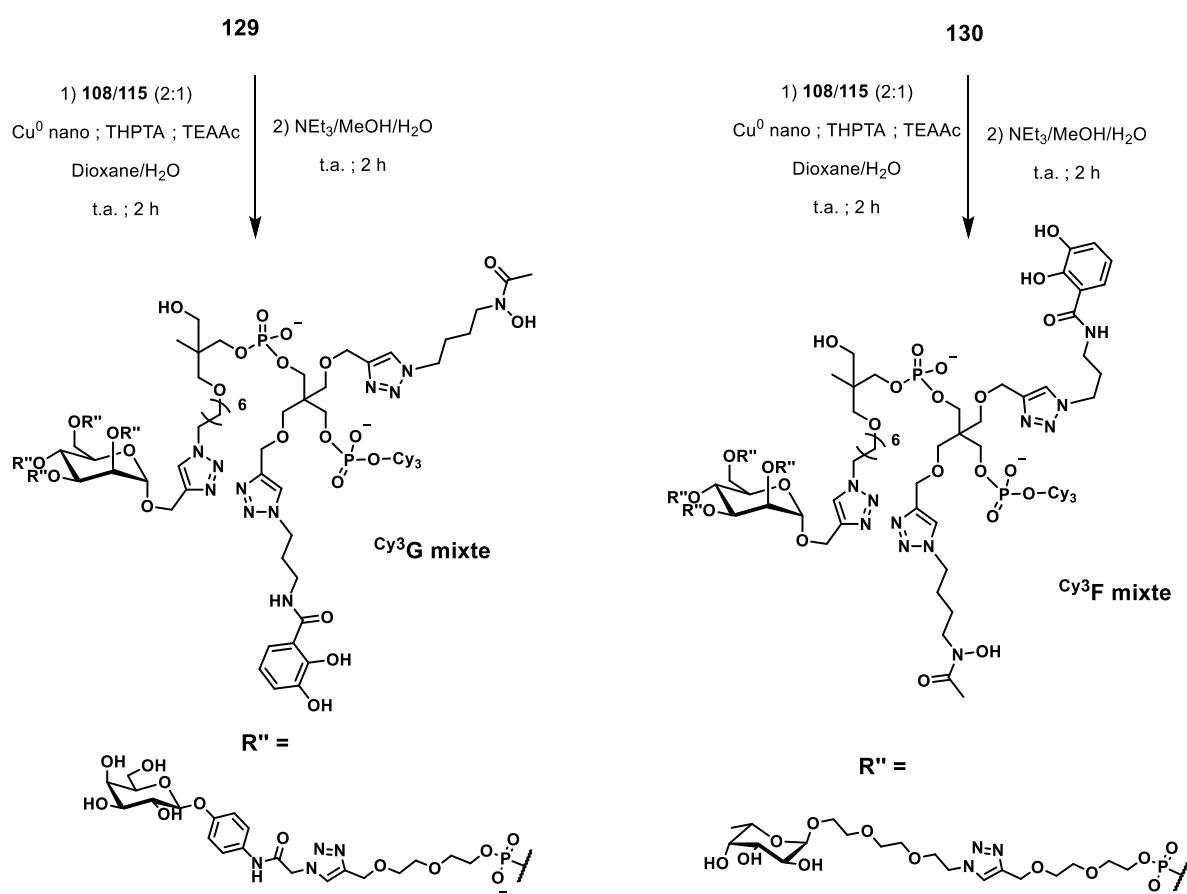
Schéma 31 : Synthèse des conjugués Cy3-glycoclusters pseudo-sidérophores mixtes
