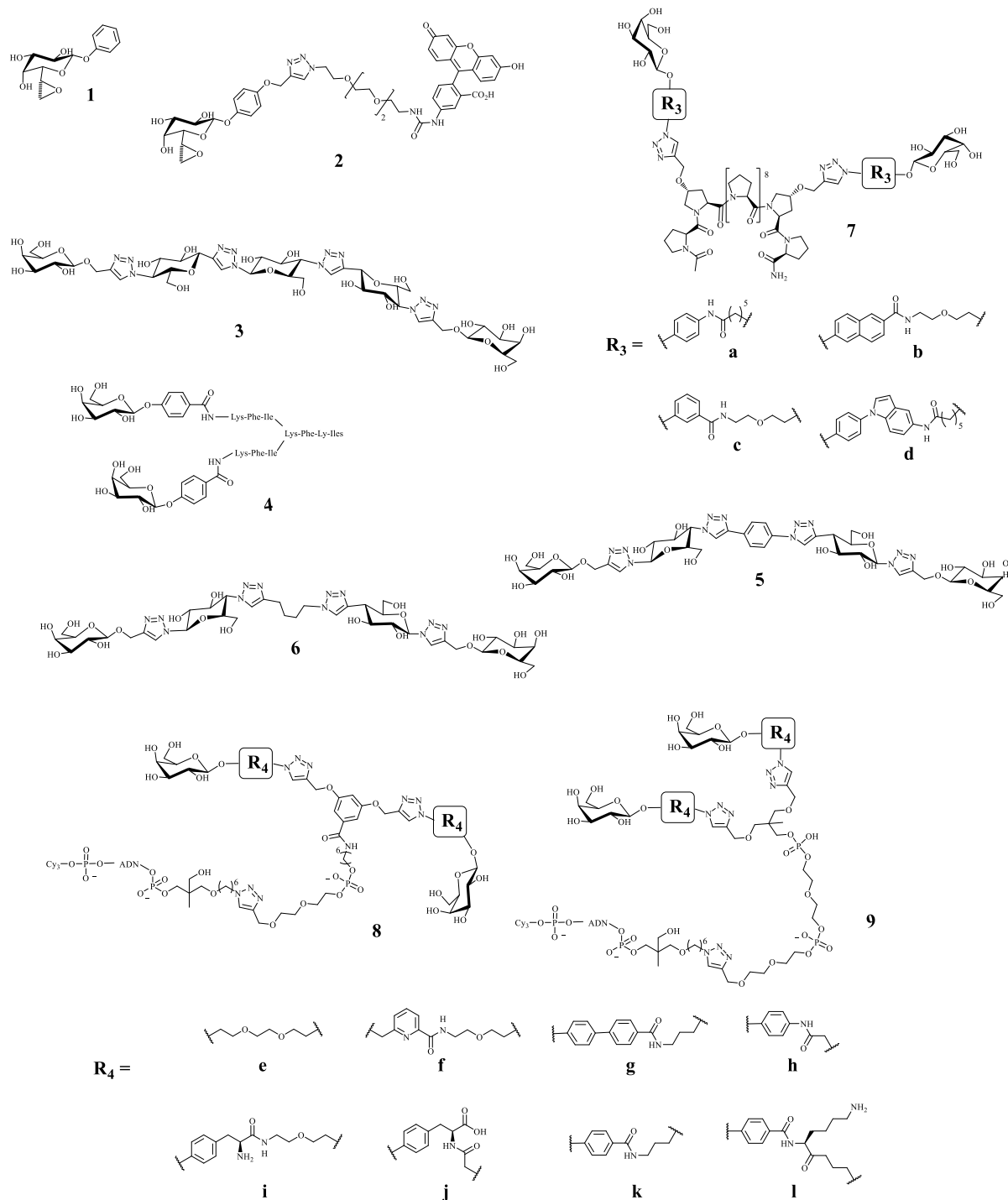
Figure 23 : Structures des ligands mono- et divalents de LecA apparues dans la littérature depuis 2015
