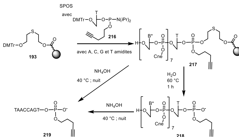
Schéma 62 : Synthèse d'un hétéroooligonucléotide modifié en 3'
