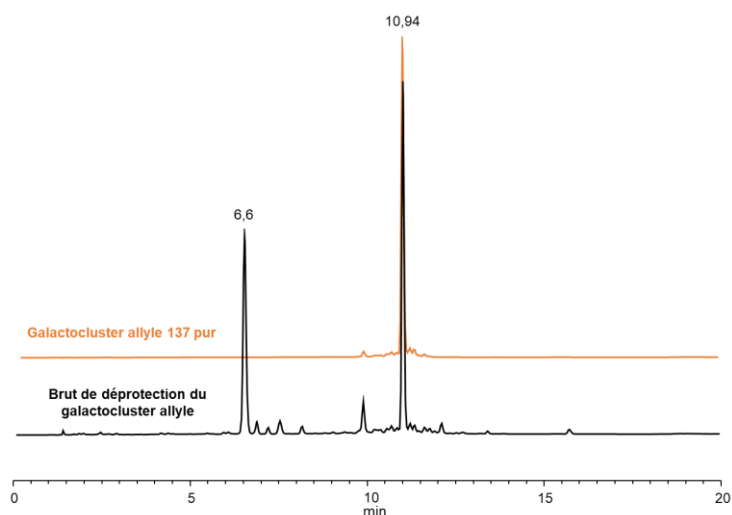
Figure 86 : Chromatogramme HPLC-C18 (gradient : 1 % CH_3CN 50 mM TEAAc - 24 % CH_3CN 50 mM TEAAc -20 min) à 260 nm du brut de déprotection de 137
