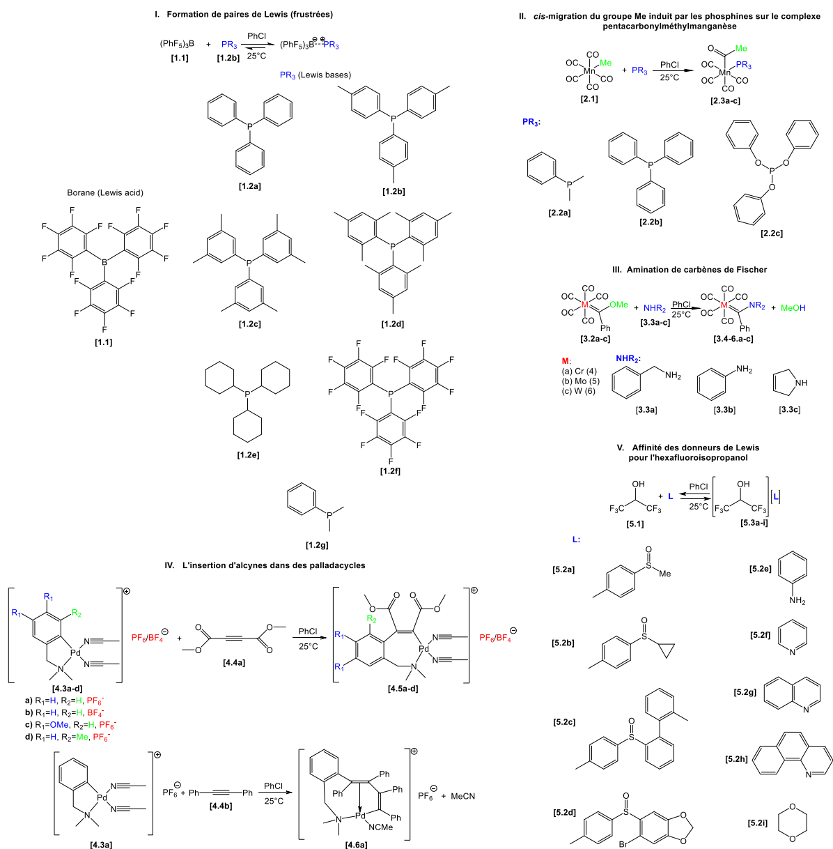
Schéma A1. Représentation schématique des systèmes réactionnels étudiés au cours de la thèse.
