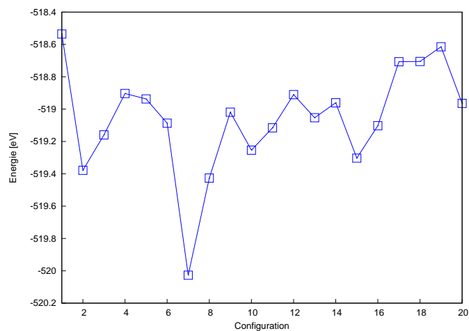
Figure 3.16 – Énergies correspondant aux structures extraites de la trajectoire de dynamique moléculaire totale.
