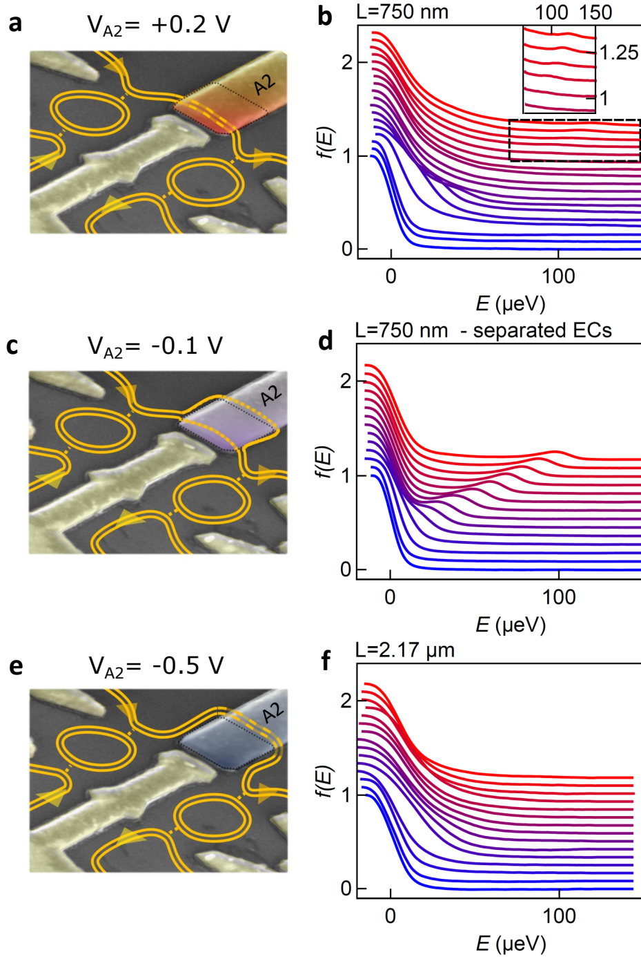
Figure 1.10: a, c, e: Micrographies électroniques à balayage en fausses couleurs d'un échantillon typique, représentant les trajectoires des canaux de bord pour V_{A2} = 0.2 \text{ V} ( a , A2 grille surlignée en orange), V_{A2} = -0.1 \text{ V} ( c , A2 grille surlignée en violet), et V_{A2} = -0.5 \text{ V} ( e , A2 grille surlignée en bleu). Dans a , les deux canaux de bord co-propagent le long d'un chemin court de L \approx 750 \text{ nm} . Dans c , les deux canaux de bord sont séparés spatialement (lignes pointillées orange) lorsqu'ils passent sous la grille A2 . Dans e , les deux canaux de bord co-propagent le long d'un chemin de L \approx 2.17 \mu\text{m} long. b, d, f: Fonction de distribution f(E) mesuré pour les configurations représentées respectivement dans a, c , et e . Chaque courbe, décalée pour plus de clarté, correspond à un incrément d'énergie d'injection \delta E_1 \approx 9 \mu\text{eV} , de E_1 \approx -26 \mu\text{eV} (bleu) à E_1 \approx 122 \mu\text{eV} (rouge, b ) et E_1 \approx 98 \mu\text{eV} (rouge, d et f ). L'encart dans b est un zoom sur la région délimitée par le carré noir pointillé.
