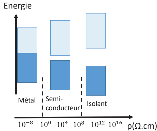
Figure 2.1 – Schéma de bandes pour un métal, un semi-conducteur et un isolant avec en abscisse \rho la résistivité spécifique du matériau permettant de discriminer leur appartenance à un groupe.
