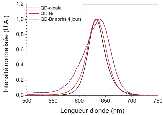
Figure 5.18 – Spectre de luminescence des BQs directement après synthèse avec leurs ligands oléates (noir), après l'échange de ligands (rouge) et 4 jours après l'échange au contact avec l'air (violet).
