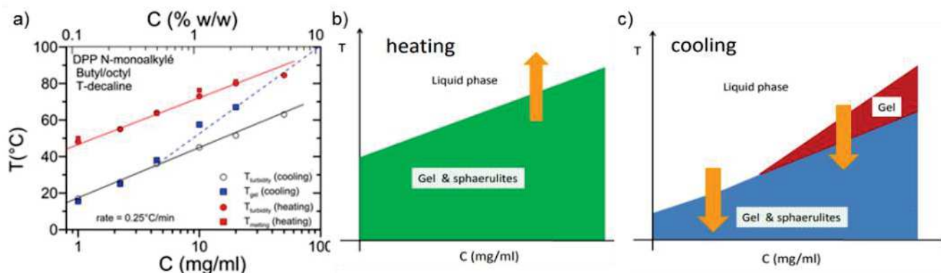
Figure 22: a) Diagramme de phase de BOTDPPma dans la trans -décaldine b) Schémas Simplifiés du diagramme de phase pendant le cycle b) de chauffage et c) de refroidissement
