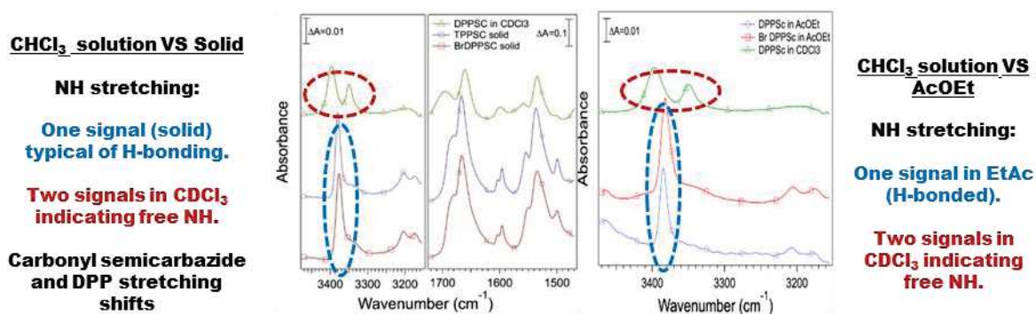
Figure 10: Comparaison des spectres IR de TDPPSC à l'état solide et en solution dans le chloroforme (à gauche) et de TDPPSC dans le chloroforme et TDPPSC et BrTDPPSC dans l'acétate d'éthyle (à droite).
