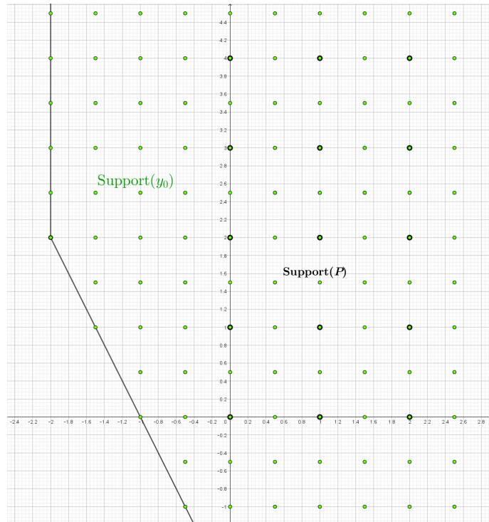
Exemple pour r = 2 , p = 2 et q = 2
