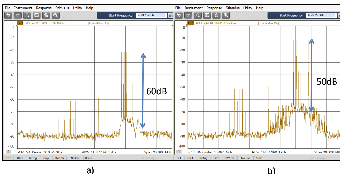
FIGURE 4.30 – Mesure brute (fortement atténuée) du spectre en entrée du DUT avant et après la compression du mélangeur
