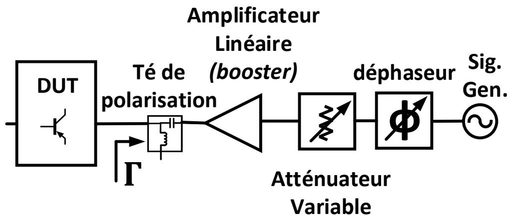
FIGURE 2.9 – load-pull actif en boucle ouverte
