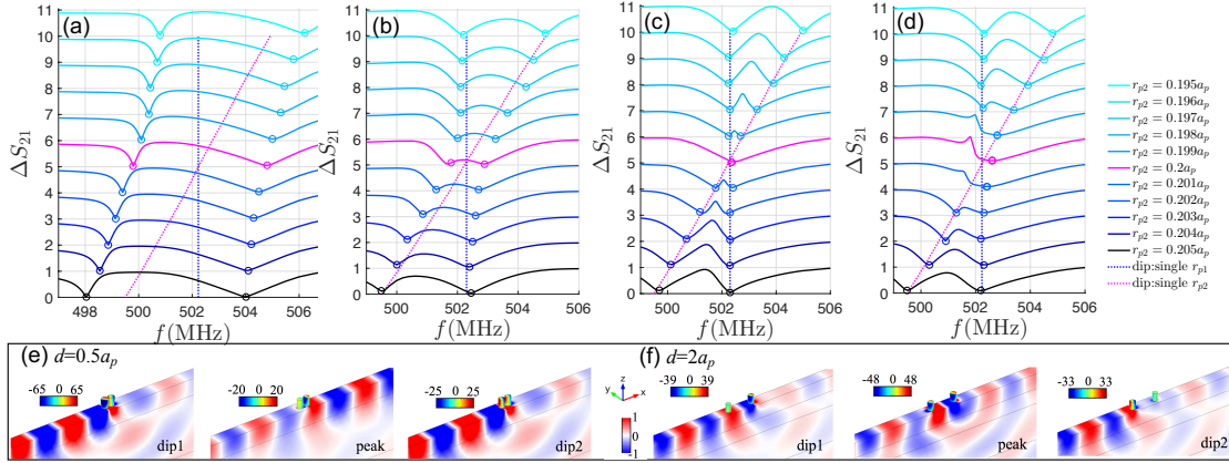
FIGURE 3 – Spectre de transmission relative des ondes de Love avec d = (a) 0,5a_p , (b) a_p , (c) 2a_p , (d) 2,4a_p lors du changement progressif du rayon du deuxième pilier r_{p2} de 0.195a_p à 0.205a_p . Le rayon du premier pilier est r_{p1}=0.2a_p , a_p = 2\mu\text{m} . (e) Champs de déplacement u_y aux creux et au pic pour l'ATS avec d=0,5a_p et r_{p1}=r_{p2}=0,2a_p . (f) est les mêmes que (e) mais pour l'AIT avec d=2a_p , r_{p1}=0,2a_p et r_{p2}=0,202a_p . La résonance FP tombe à d=2a_p .
