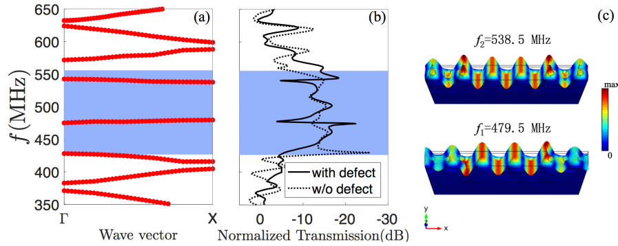
FIGURE 4 – (a) Structure de bande des modes de Love pour le CPn à trous contenant une cavité dans la direction \Gamma X . La région bleu est la bande interdite originale du CPn à trous. La largeur de cavité est W=5a . (b) Spectre de transmission relative des ondes de Love avec et sans défaut (cavité). Le nombre de trous à chaque côté est N_{CPn}=4 . (c) Champs de déplacement totaux et déformations dans la supercellule pour les deux modes de cavité. Conditions périodiques sont appliqués suivant la direction y . r_h=0,2a , H=0,6a , a=4\mu\text{m} .
