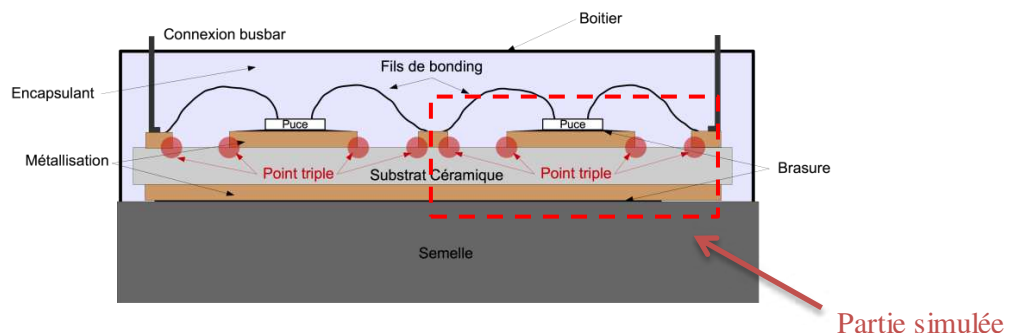
Figure 20 : Coupe schématique du module de puissance
