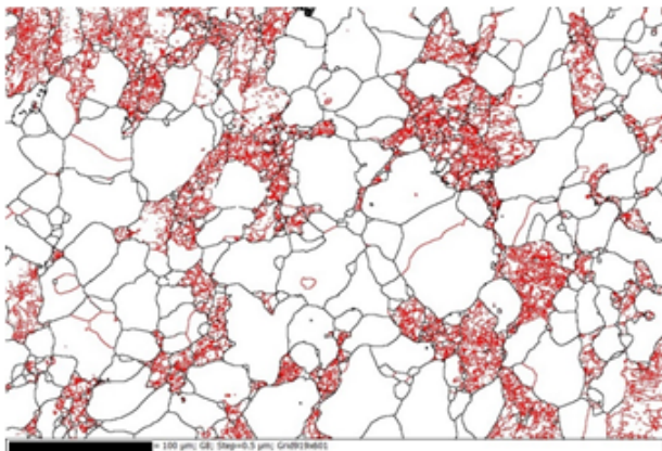
FIGURE C.a – Cartographies EBSD réalisées sur 3 échantillons de tungstène
