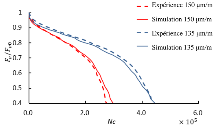
Figure 6: Comparaison d'expériences et de simulations sous différents niveaux de contrainte.
