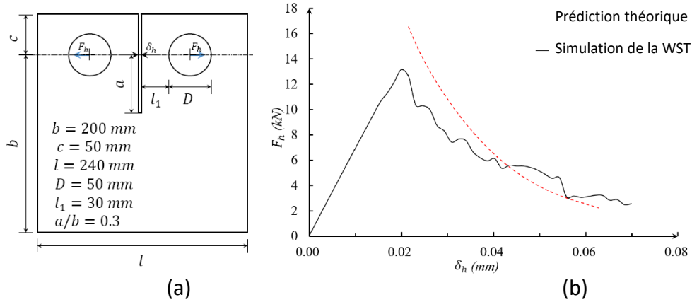
Figure 2: (a) Géométrie de la WST. (b) Le résultat de la simulation et l'ajustement par LEFM
