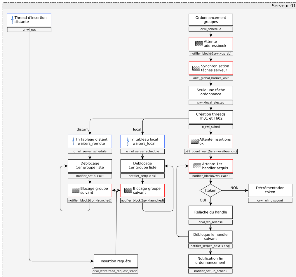
Figure 4.5: Processus d'ordonnement des groupes de requêtes d'insertion
