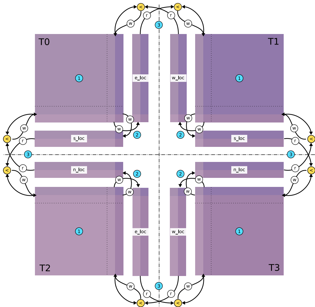
Figure 5.8: Principe ORWL de local update / global update appliqué à la mise à jour de la carte d'attache aux données
