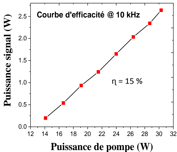
Figure III.19 : La courbe d'efficacité laser obtenue pour une Frép de 10 kHz.
