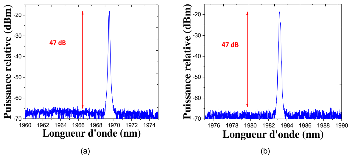
Figure II.18 : Spectre mesuré en sortie de la cavité, montrant l'émission laser obtenue avec (a) le VBG centré à 1970 nm (pic laser à 1969,6 nm), (b) le VBG centré à 1984 nm (pic laser à 1983,2 nm).
