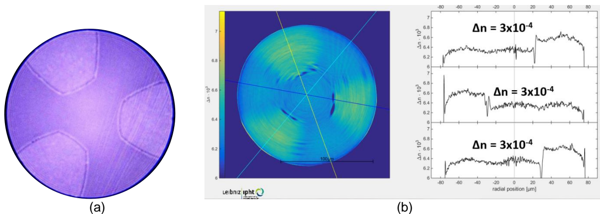
Figure III.9 : La fibre de test constituée d'un barreau utilisé pour la gaine passive dopée aluminium entouré de trois barreaux actifs et trois barreaux utilisés pour la gaine passive (a), et les résultats obtenus de la mesure d'indice réalisée selon trois axes différents avec l'appareil commercial IFA100 (Inter Fiber Analysis), montrant une valeur de \Delta n = +3 \times 10^{-4} .
