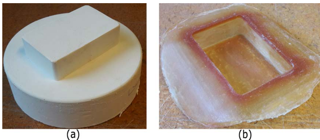
FIGURE II.18 – Photographies : (a) du contre-moule en plâtre; (b) du moule en latex obtenu après séchage de couches successives de latex liquide.
