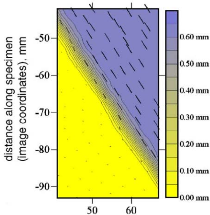
FIGURE I.10 – [Rec06] Champ de déplacement au niveau d'une bande de cisaillement dans un matériau granulaire soumis à un test biaxial. Dans le référentiel du bloc du bas, on observe un fort gradient au niveau de la bande de cisaillement.
