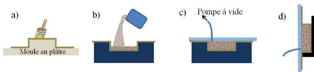
FIGURE II.19 – [LB14]. Schéma des étapes de préparation des échantillons : a) application de couches successives de latex liquide sur un contre-moule en plâtre; b) remplissage du moule avec le matériau granulaire; c) dépressurisation de l'échantillon; d) installation de l'échantillon sur le bâti expérimental.
