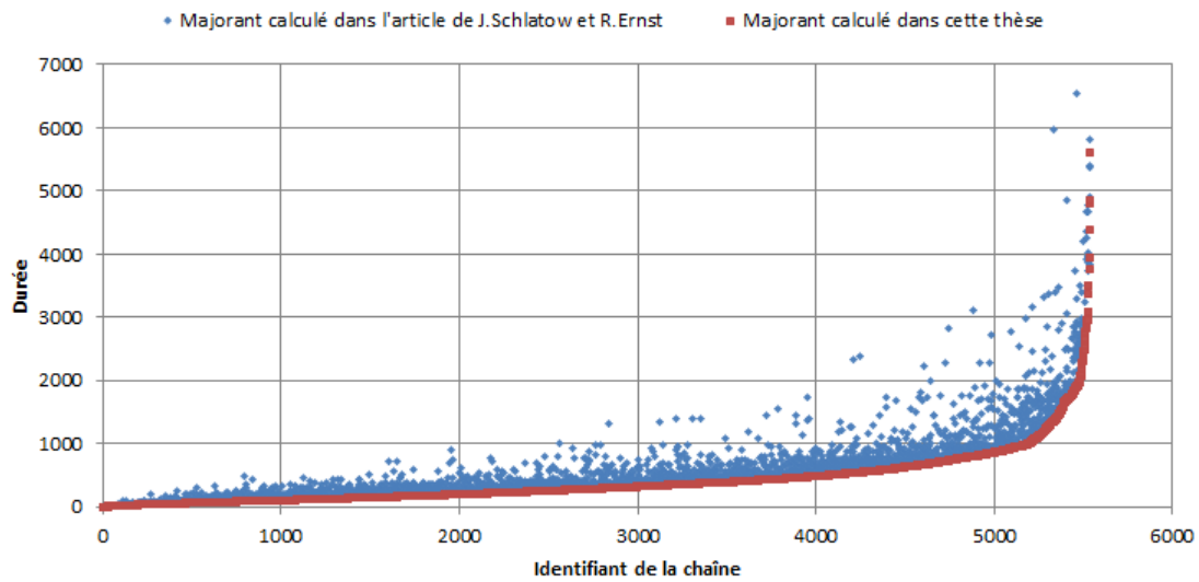
FIGURE 3.12 – Comparaison des majorants sur la latence au pire cas quand les chaînes sont sporadiques ou périodiques, et synchrones. En abscisse les identifiants des chaînes ordonnées selon la valeur du majorant calculé dans le chapitre 3.
