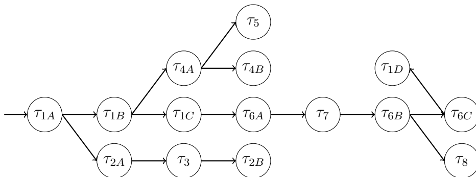
FIGURE 2.9 – Exemple d’arbre
