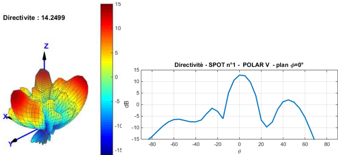
Figure 76 : diagramme de rayonnement pour un réseau totalement excité
