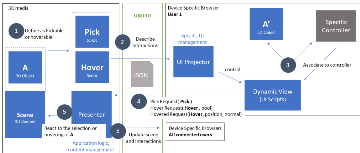
FIGURE 2.8 – Fonctionnement des briques d'interaction Pick et Hover permettant la sélection et le pointage d'objets 3D.
