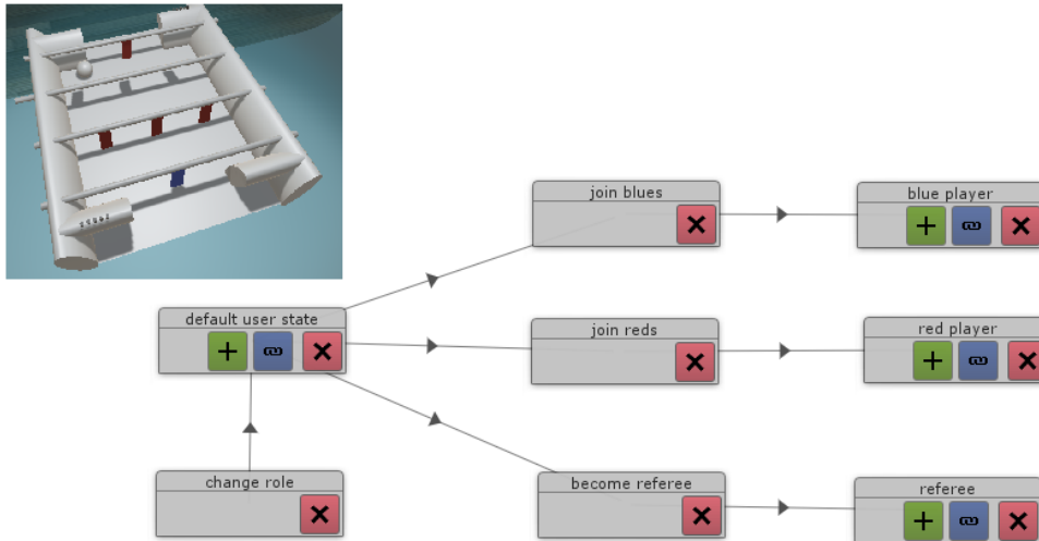
FIGURE 3.3 – Exemple : Graphe des états utilisateur pour un jeu de babyfoot virtuel
