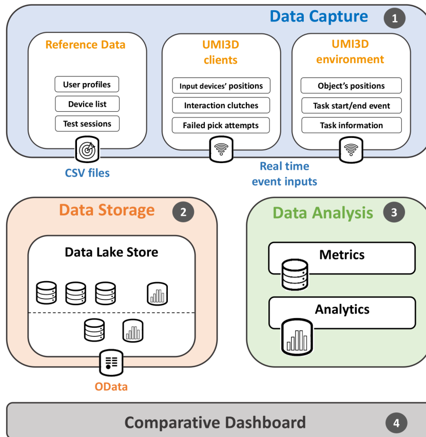
FIGURE 5.2 – Utilisation d'une plateforme Big Data pour l'évaluation des navigateurs UMI3D.
