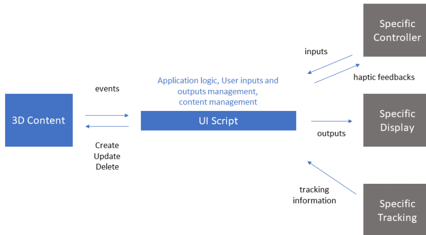
FIGURE 2.1 – Architecture naïve pour les applications 3D
