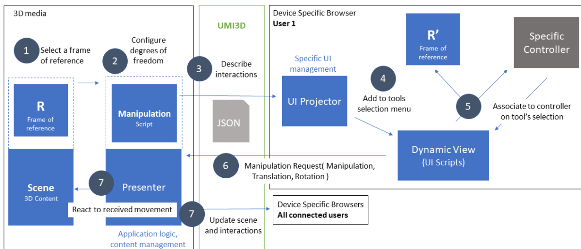
FIGURE 2.10 – Fonctionnement de la brique manipulation.
