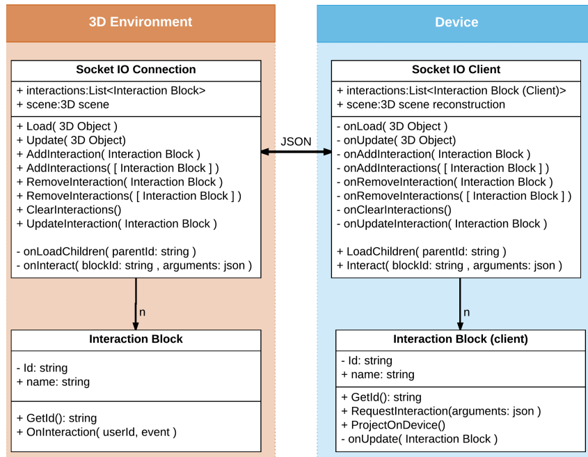
FIGURE 2.15 – Communication entre un navigateur UMI3D et un média 3D
