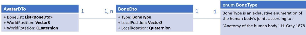
FIGURE 4.1 – Modèle de données pour le suivi utilisateur dans UMI3D.
