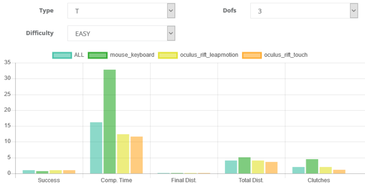
FIGURE 5.5 – Moyennes des métriques pour la tâche de translation avec trois degrés de liberté et une faible difficulté
