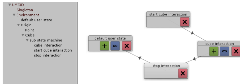
FIGURE 3.4 – Stockage d'un sous-graphe d'états utilisateur dans un objet préfabriqué.
