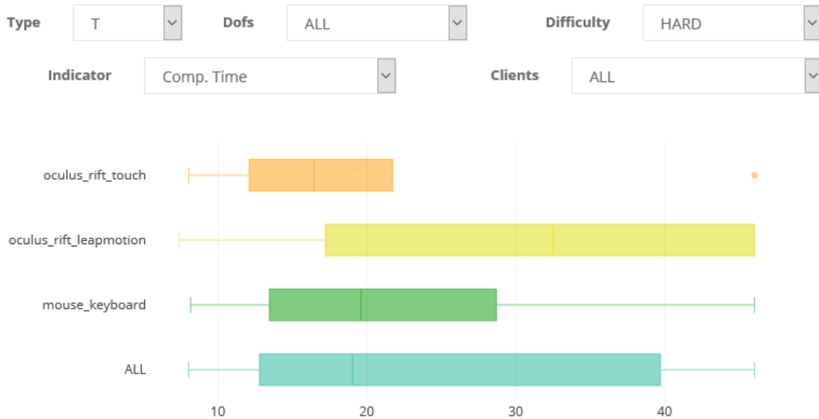
FIGURE 5.6 – Boîtes à moustaches du temps de complétion pour les tâches de translation avec une haute difficulté
