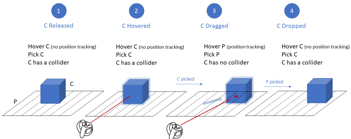
FIGURE 2.9 – exemple : glissé-déposé sur un plan 2D.
