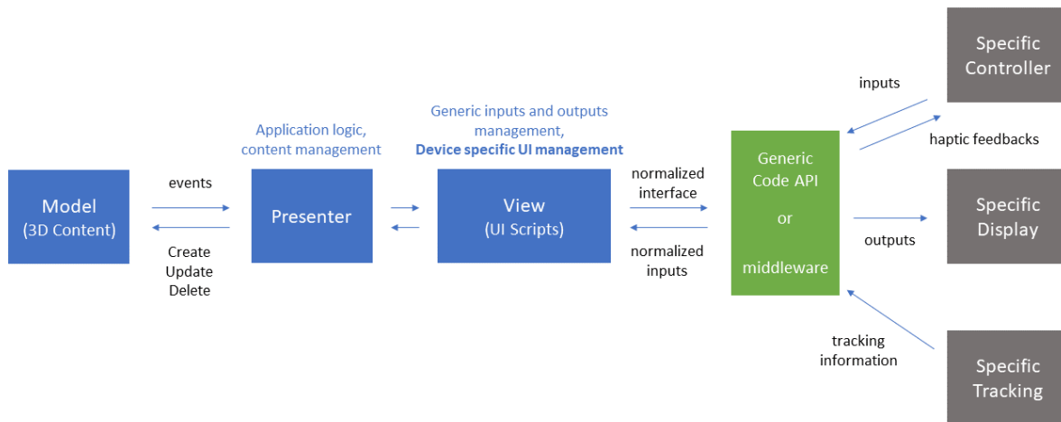
FIGURE 2.3 – Positionnement des standards et outils existants (Middle VR, WebVR, OpenXR, etc.)
