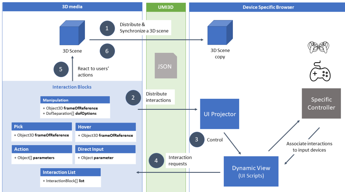
FIGURE 2.7 – Fonctionnement du protocole UMI3D : définition de contrats d'interaction avec un support quelconque à l'aide d'un nombre finis de briques d'interaction.
