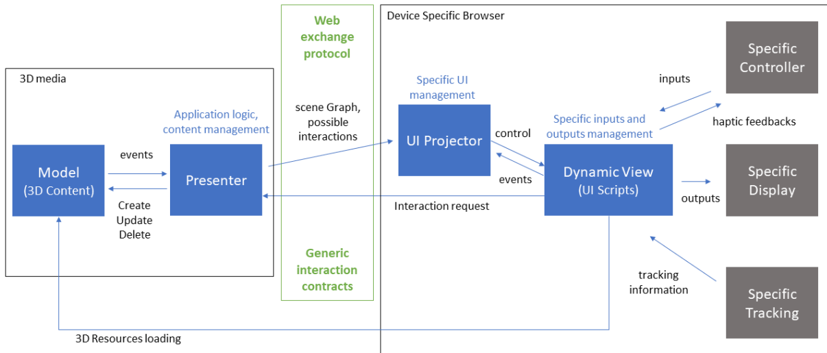
FIGURE 2.4 – Architecture proposée pour des médias 3D permettant la collaboration multi-supports en RV/RA.
