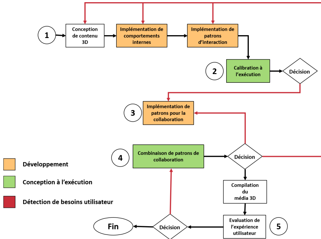
FIGURE 3.6 – Proposition d'un processus de conception des médias 3D
