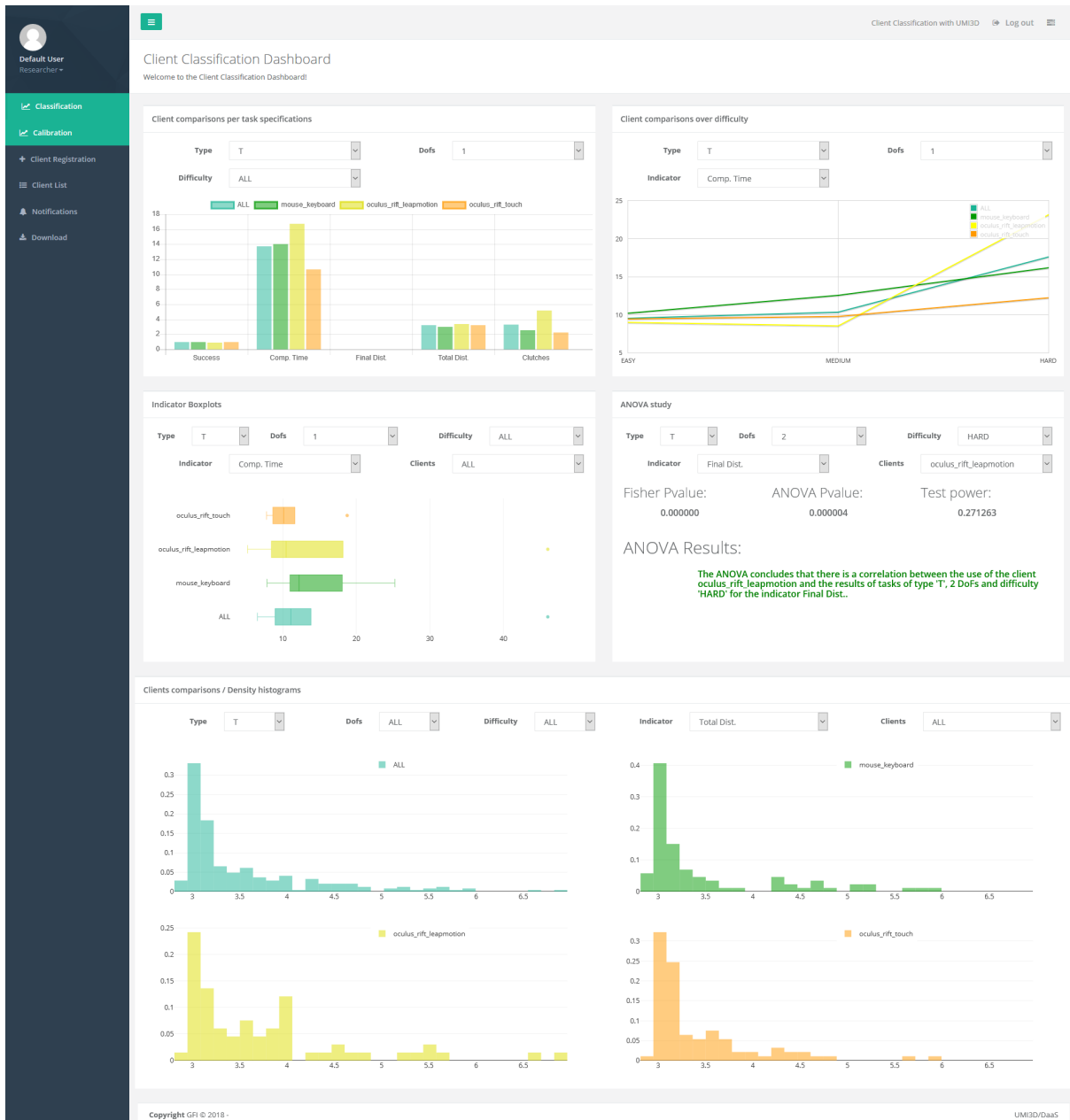
FIGURE 5.4 – Aperçu des tableaux de bord
