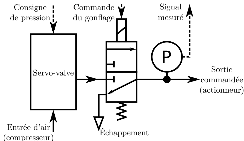
FIGURE 4.11 – Schéma fonctionnel du banc d'essai pneumatique.
