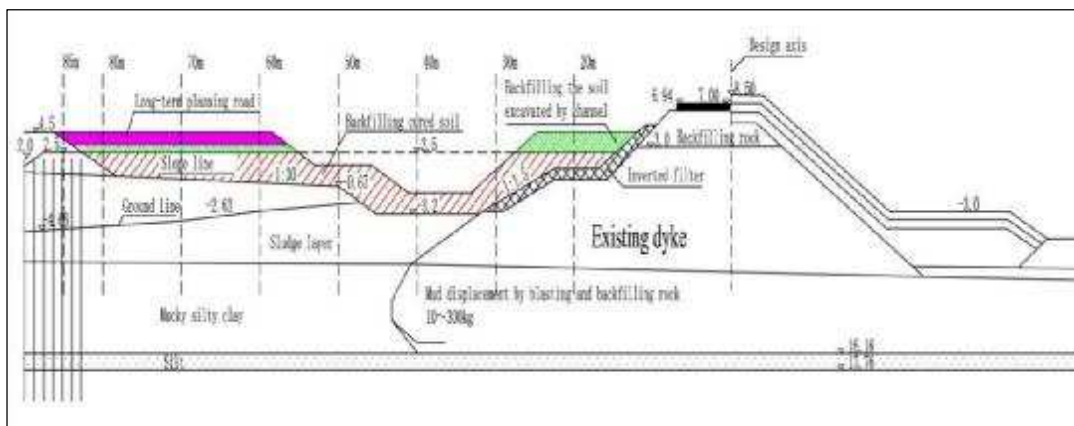
Figure 3.4-7. Étape 4: mise en place de la plate-forme définitive (projet à venir)
